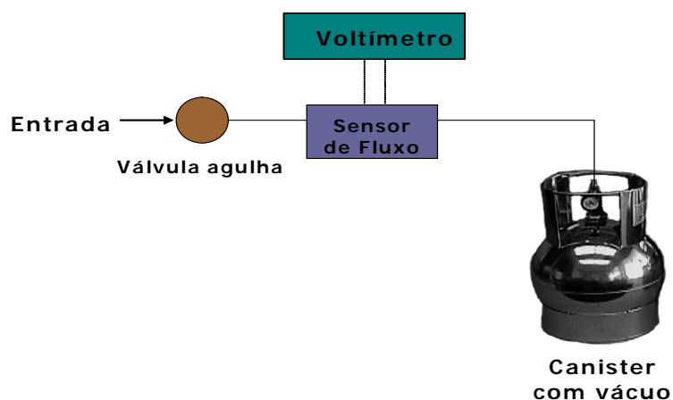
Figura 33 - Esquema do sistema de amostragem de ar adaptado para canister.
