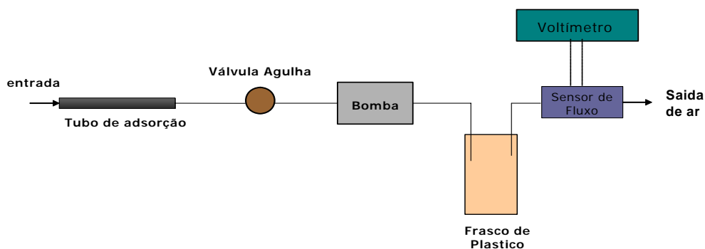
Figura 30 - Esquema do sistema de amostragem de ar em tubos adsorventes, desenvolvido pelo pesquisador Jim Greemberg do NCAR.
