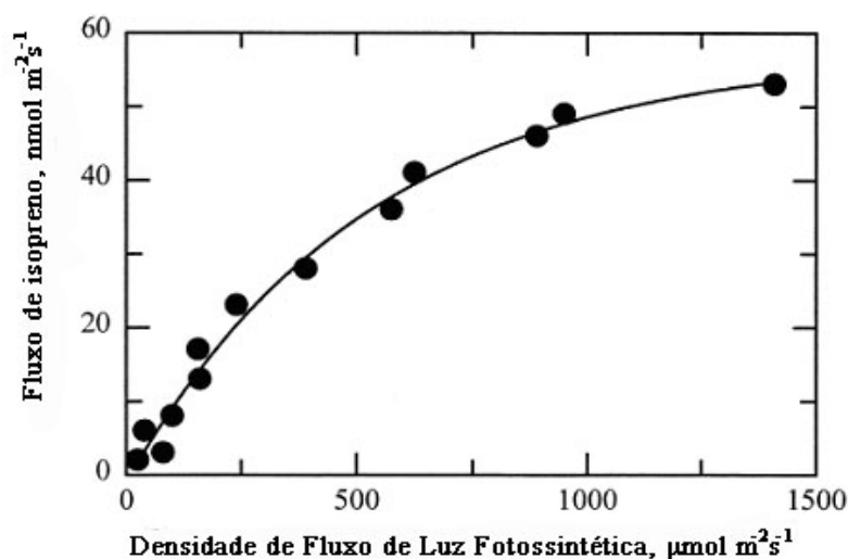
Figura 13 - Emissão de isopreno pela oak branca ( Quercus alba ) em função da densidade de fluxo de fótons fotossintéticos. Fluxos são expressos por unidade de área de folha (dados de HARLEY et al. 1996).
