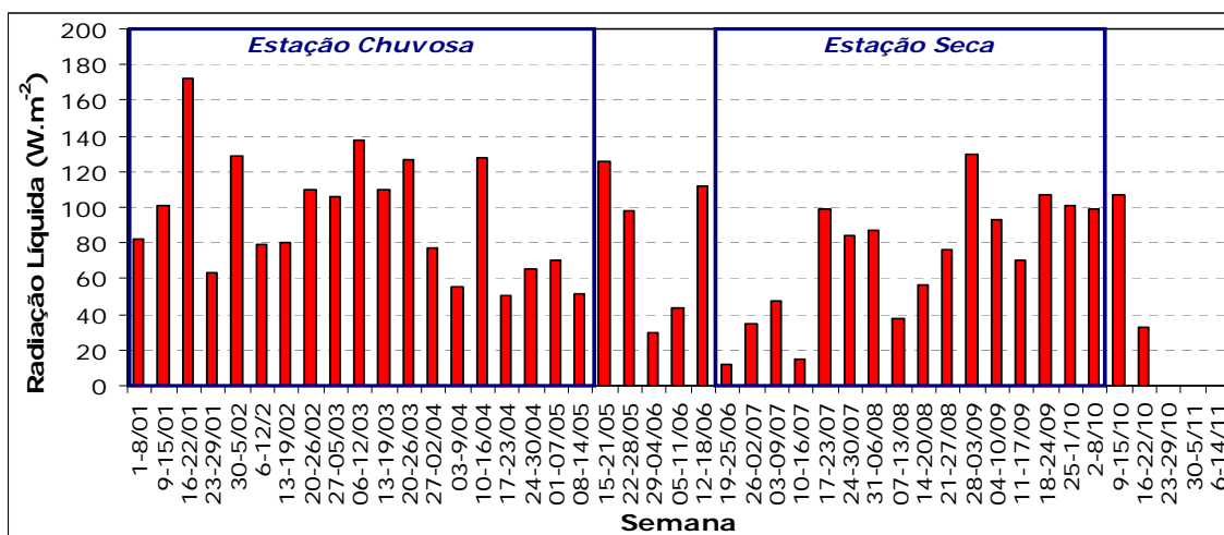
Figura 47 - Média Semanal de PAR, durante o ano de 2002, na pastagem na FNS (TROSTDORF – 2004).
