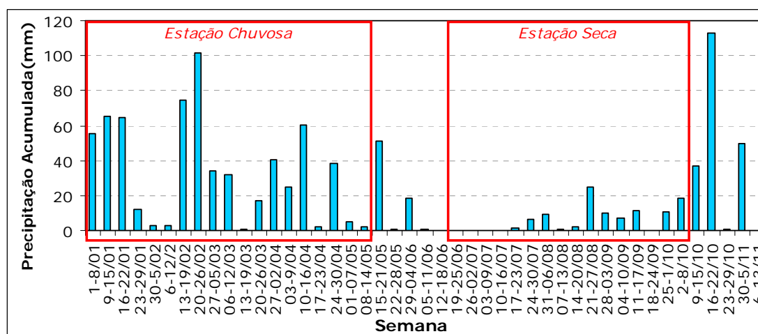
Figura 45 - Precipitação Acumulada Semanal durante o ano de 2002 na pastagem – FNS – RO (TROSTDORF – 2004).
