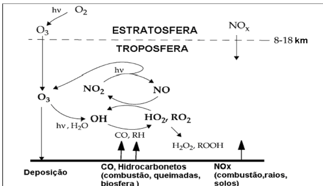
Figura 17 - Esquema ilustrando a química do ozônio troposférico, acoplando os ciclos químicos de O_3 , NO_x , HO_x . ( RO_2 = radicais peroxi orgânicos) (adaptação de Jacob, 2000).
