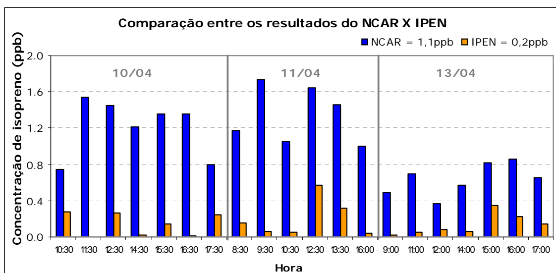
Figura 37 - Comparação dos resultados de isopreno obtidos pelo IPEN e pelo NCAR, utilizando tubos adsorventes.
