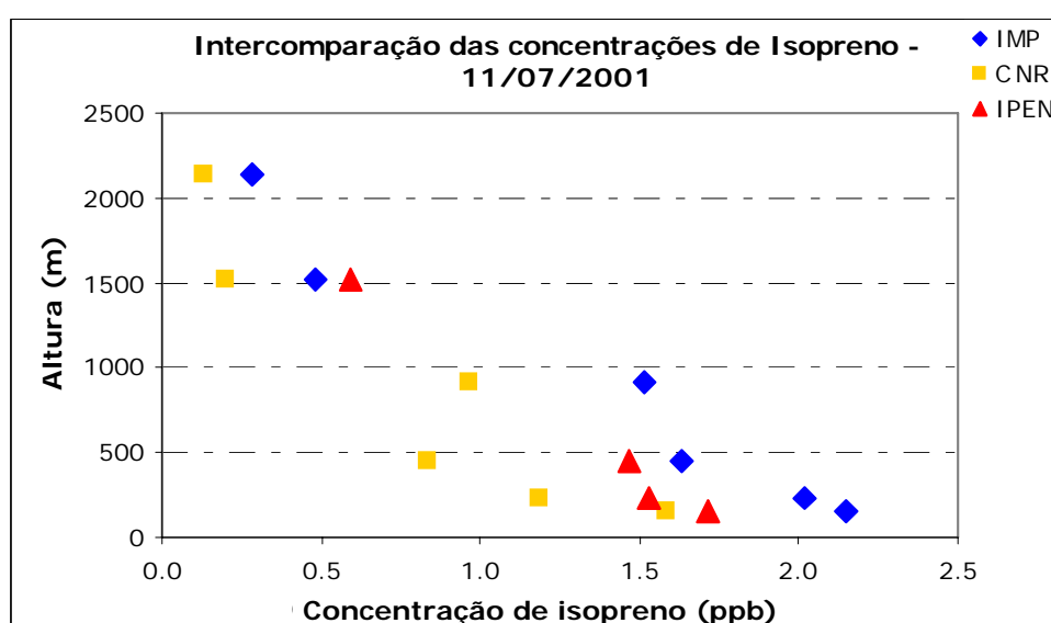
Figura 38 - Intercomparação dos resultados de isopreno obtidos pelo IPEN, pelo MPI e pelo CNR.
