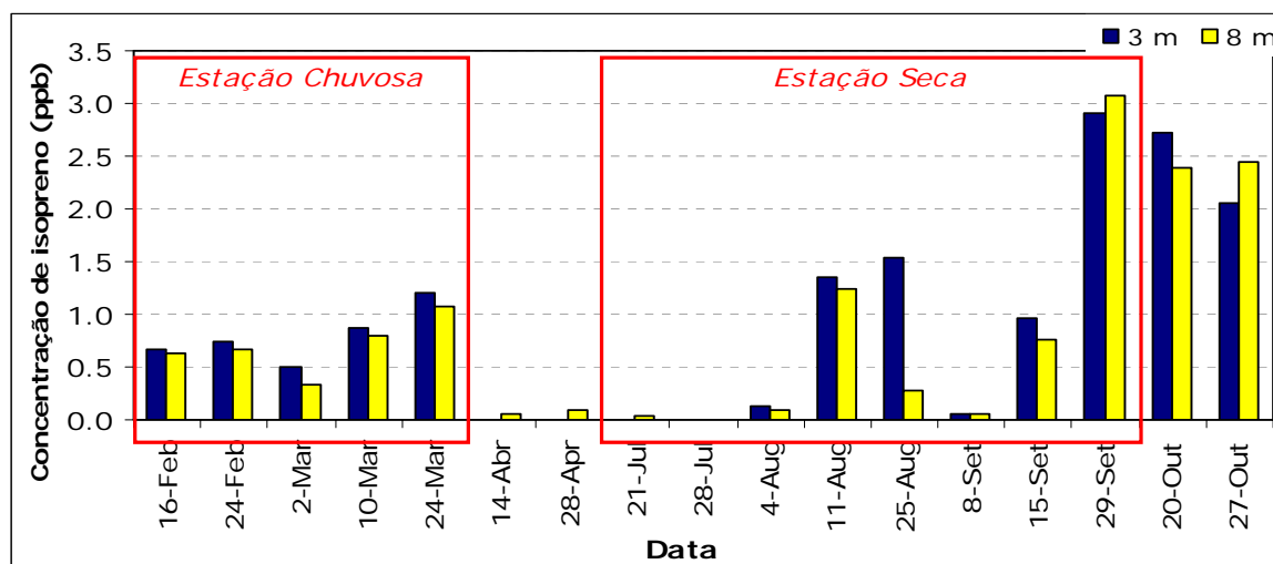
Figura 51 - Concentração de Isopreno durante o ano de 2002 na FNS (Pasto).
