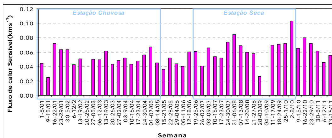
Figura 42 - Média semanal de Fluxo de Calor-ano 2002 – Rebio Jaru. (TROSTDORF – 2004)
