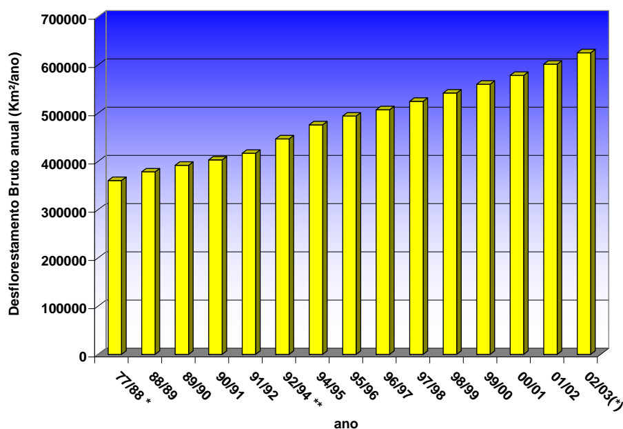
Figura 3 - Extensão de desflorestamento acumulado bruto (em km 2 ) de abril de 1988 a agosto de 2000. (CPTEC).
