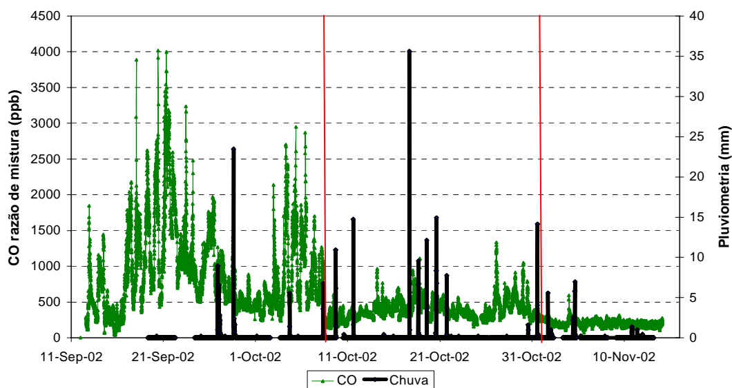
Figura 40 - Concentração de Monóxido de Carbono (CO) e a precipitação durante os meses de setembro de 2002 a novembro de 2002. (TROSTDORF – 2004)
