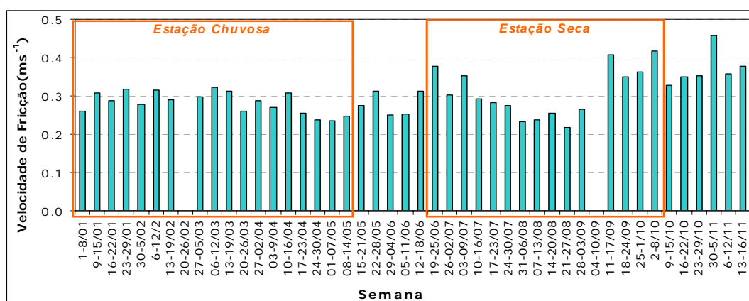
Figura 43 - Média semanal de Velocidade de Fricção-ano 2002 – Rebio Jaru. (TROSTDORF – 2004)
