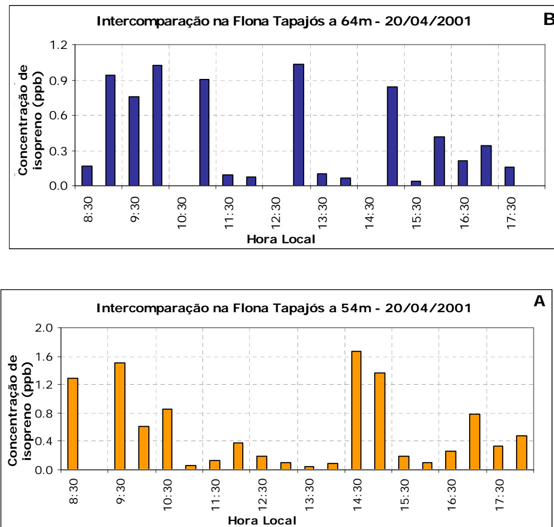
Figura 36 - Concentração de isopreno nos tubos de adsorção do IPEN, em duplicata, a cada hora a 54m (A) e a 64m (B) de altura.
