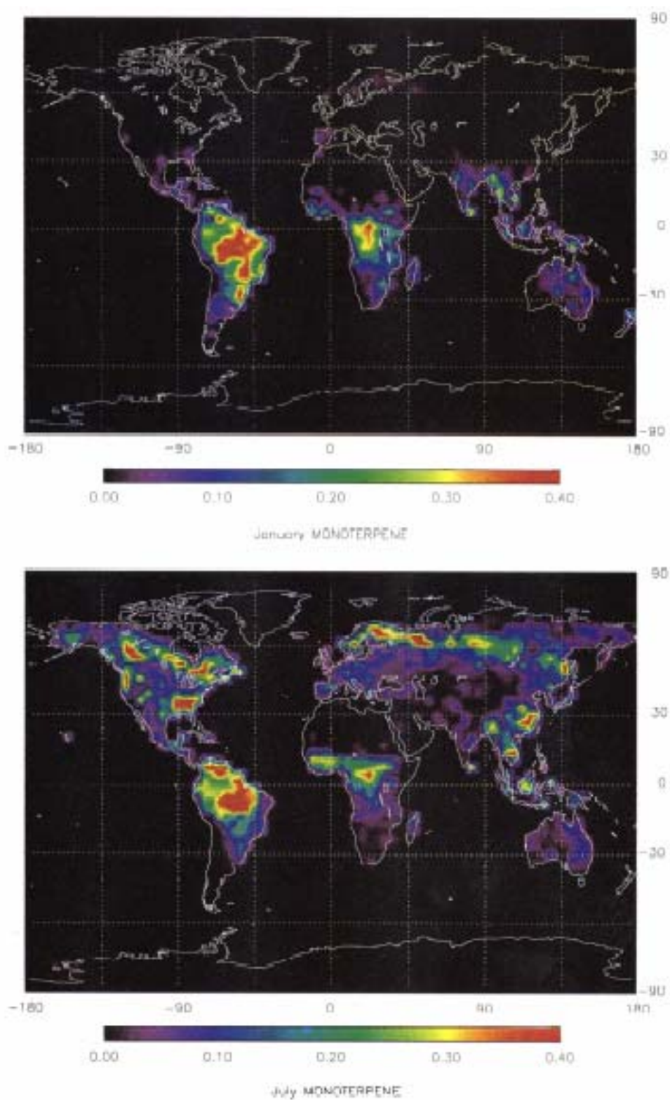
Figura 11 - Distribuição Global da emissão dos monoterpenos, g.C.m -2 .mês -1 , estimada para os meses de Janeiro (acima) e Julho (abaixo). (GUENTHER et al., 1995).
