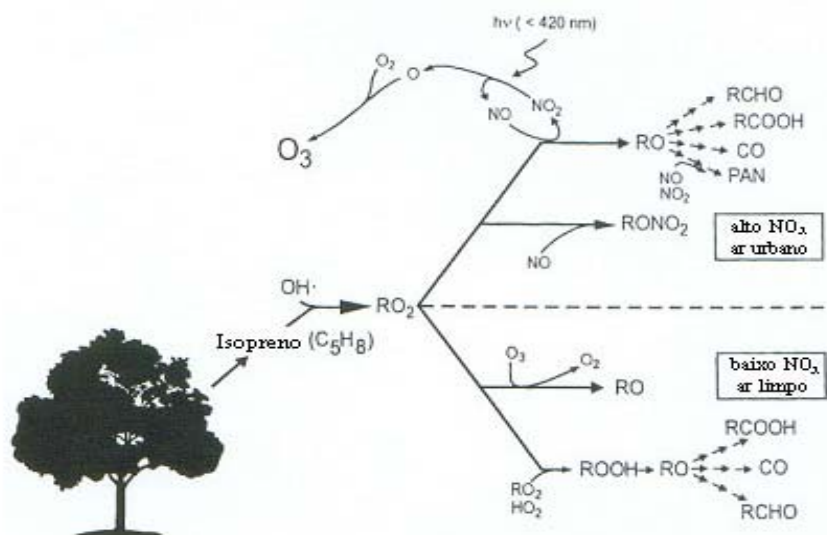
Figura 16 - Esquema de reação extremamente simplificado para ilustrar os produtos finais de oxidações de isopreno através do radical OH. A metade superior da figura ilustra a situação de ar poluído, contendo altas concentrações de NO x e a metade inferior ilustra a situação de ar limpo. (HARLEY et al., 1999).
