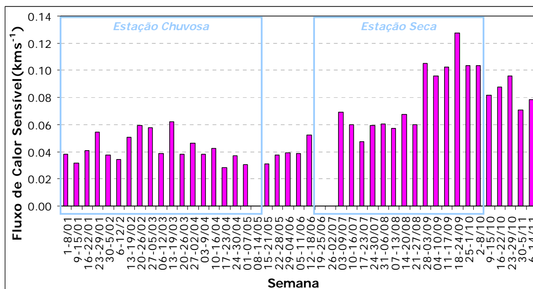
Figura 48 - Média Semanal de Fluxo de Calor Sensível durante o ano de 2002 na pastagem na FNS (TROSTDORF – 2004).
