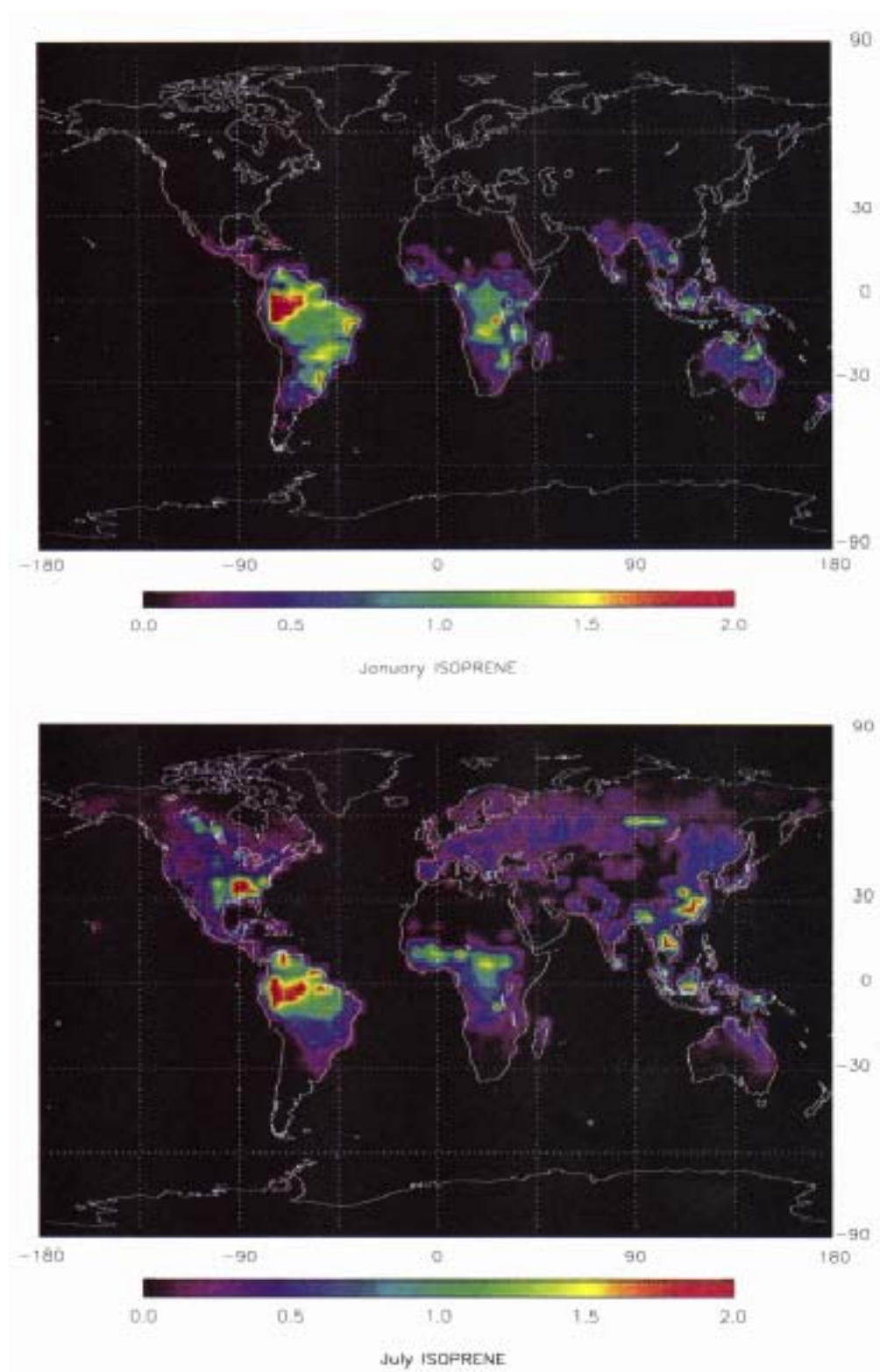
Figura 10 - Distribuição Global da emissão de isopreno, em \text{g.C.m}^{-2}.\text{mês}^{-1} , estimada para os meses de Janeiro (acima) e Julho (abaixo). (GUENTHER et al., 1995).
