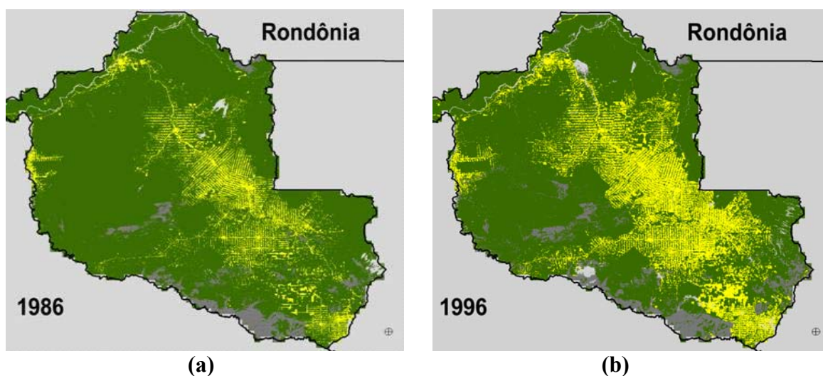
Figura 5 - Imagens de Satélite da Região de Rondônia, centralizando o desmatamento da BR 364 durante o ano de 1986 (a), BR 364 durante o ano de 1996 (b). FONTE: IPAM e INPE
