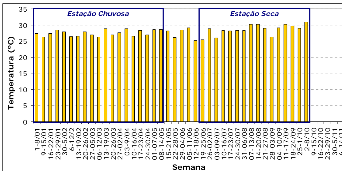
Figura 46 - Média Semanal de Temperatura, durante o ano de 2002, na pastagem na FNS (TROSTDORF – 2004).
