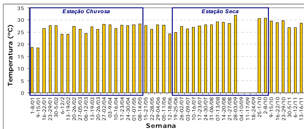
Figura 41 – Média semanal de Temperatura – ano 2002 – Rebio Jaru. (TROSTDORF – 2004)
