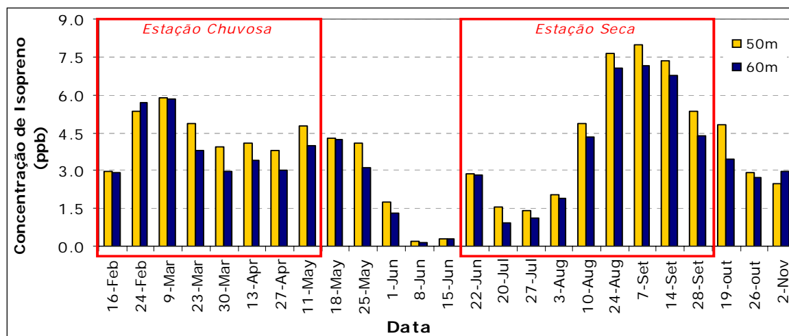
Figura 50 – Concentração de Isopreno durante o ano de 2002 na Rebio Jarú.
