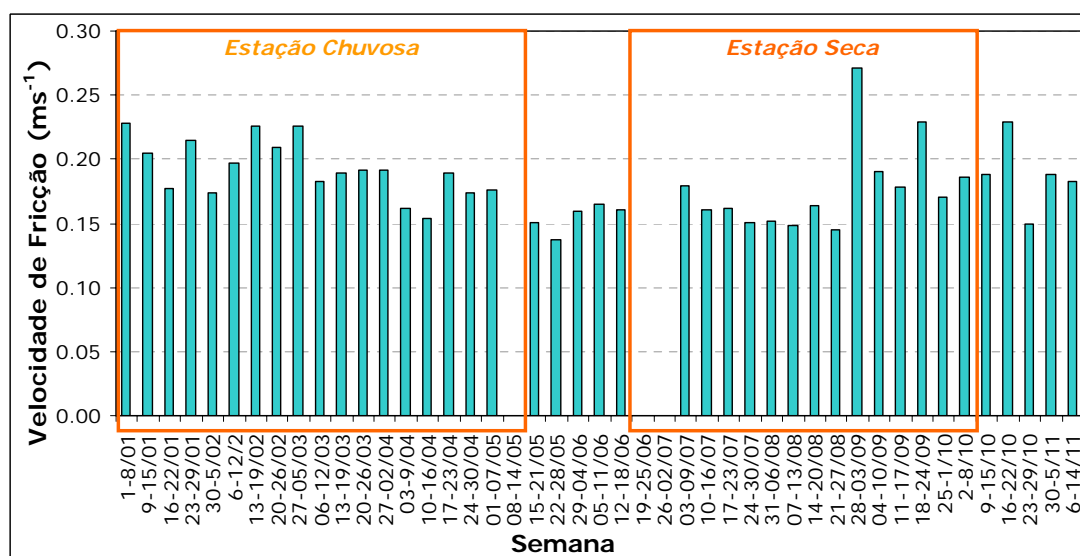
Figura 49 - Média Semanal de Velocidade de Fricção, durante o ano de 2002, na pastagem na FNS (TROSTDORF – 2004).
