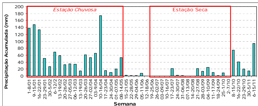
Figura 39 - Precipitação Acumulada Semanal durante o ano de 2002 na Rebio Jarú. (TROSTDORF – 2004)
