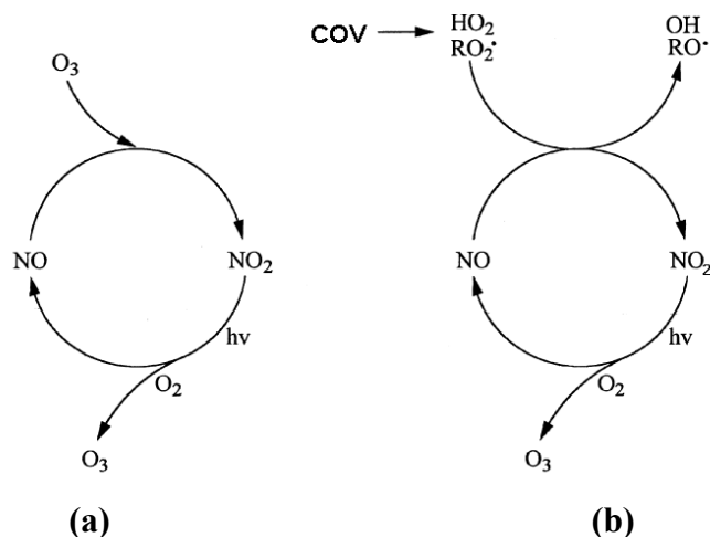
Figura 18 - Esquema das reações envolvidas na conversão NO-NO 2 e formação de O 3 em [a] sistema NO-NO 2 -O 3 em ausência de COVs e [b] sistema NO-NO 2 -O 3 na presença de COVs (adaptado de ATKINSON, 2000).
