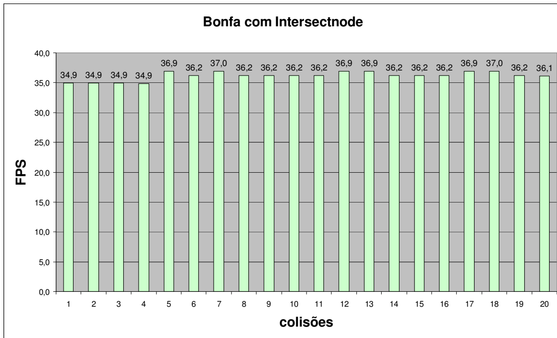
Figura 6.7 – FPS de 20 colisões com Intersectnode do protótipo Bonfa
