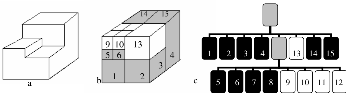
Figura 3.12 - Representação do sólido por Octree. a) sólido b) divisão recursiva do sólido c) Octree representada.
