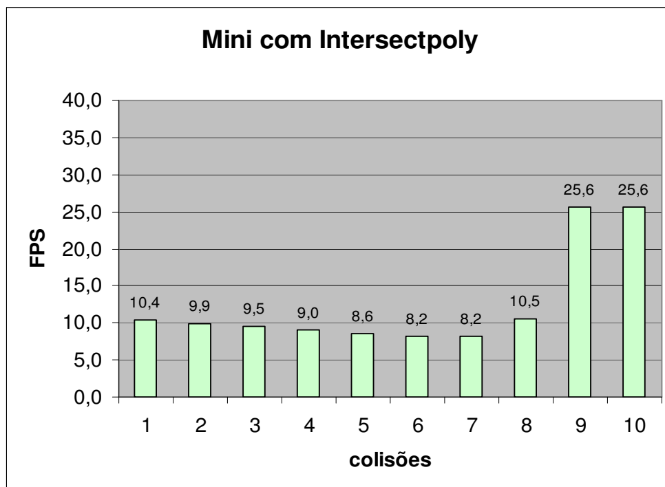
Figura 6.13 – FPS de 10 colisões com Intersectpoly do protótipo Mini
