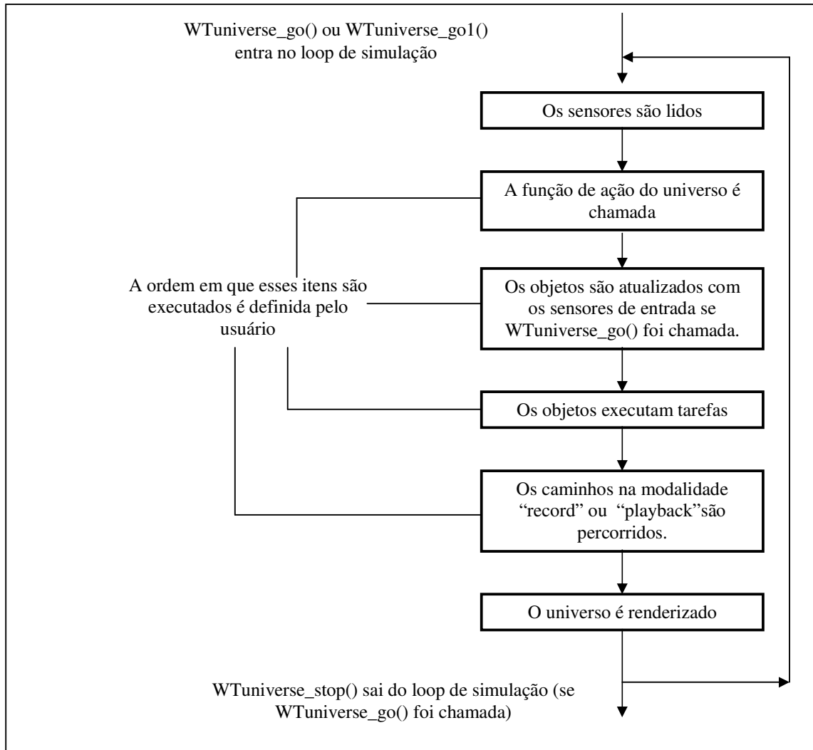
Figura 4.1 – Loop de simulação padrão
