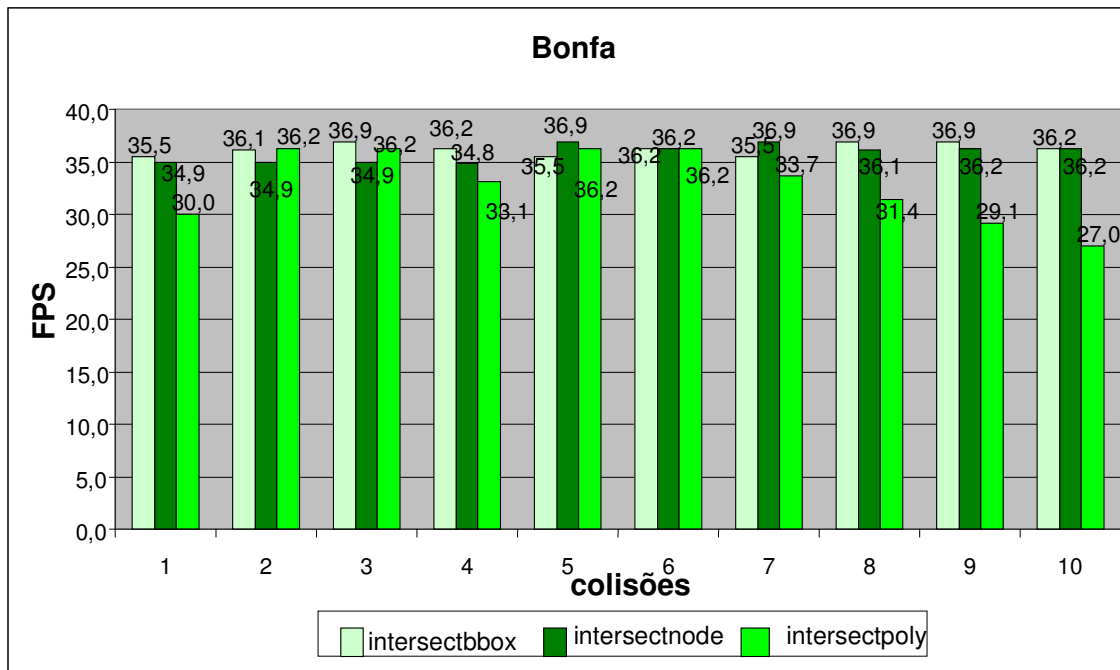
Figura 6.5 – FPS com 10 colisões entre as três técnicas com o Protótipo Bonfa
