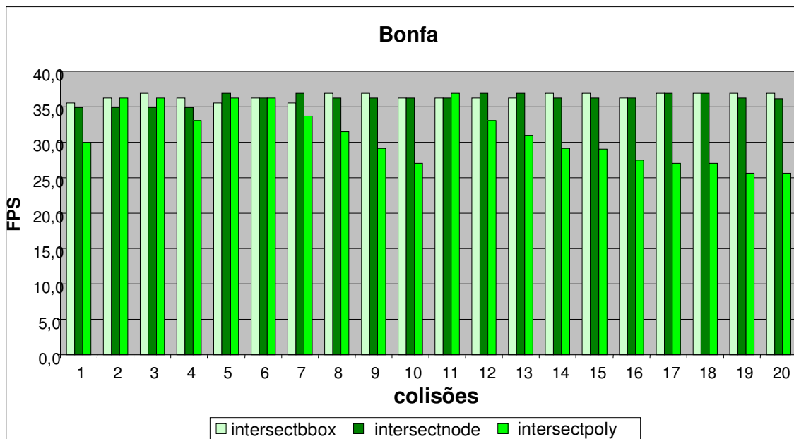
Figura 6.9 – FPS com 20 colisões entre as três técnicas com protótipo Bonfa
