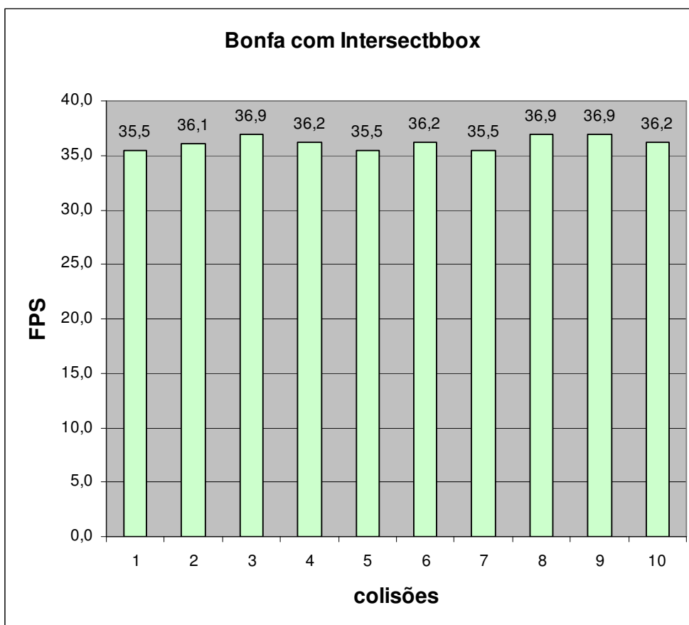
Figura 6.2 – FPS de 10 colisões com Intersectbbox do protótipo Bonfa
