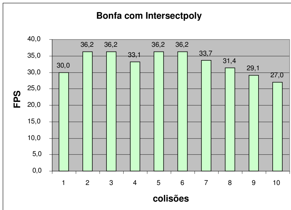
Figura 6.4 – FPS de 10 colisões com Intersectpoly do Protótipo Bonfa
