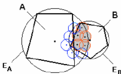
Figura 3.4 – Visualização dos prováveis Pontos de colisão (Nascimento, 2003).
