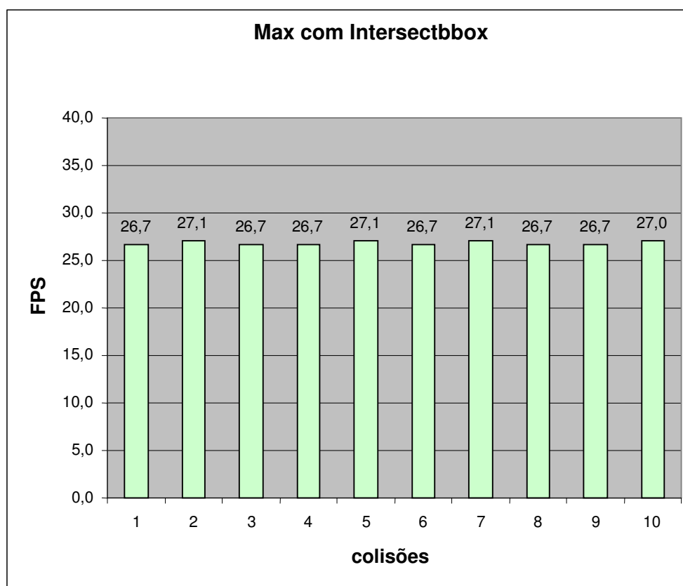
Figura 6.20 – FPS de 10 colisões com Intersectbbox do protótipo Max
