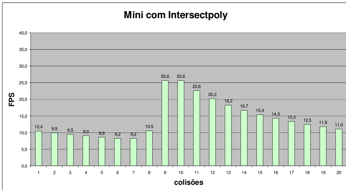
Figura 6.17 – FPS de 20 colisões com Intersectpoly do protótipo Mini
