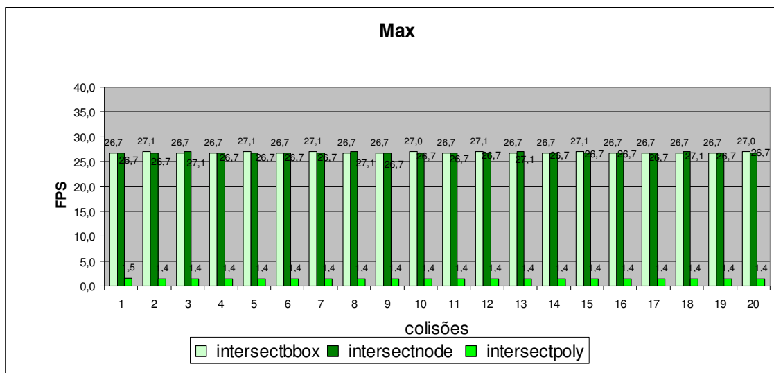
Figura 6.27 – FPS com 20 colisões entre as três técnicas do protótipo Max
