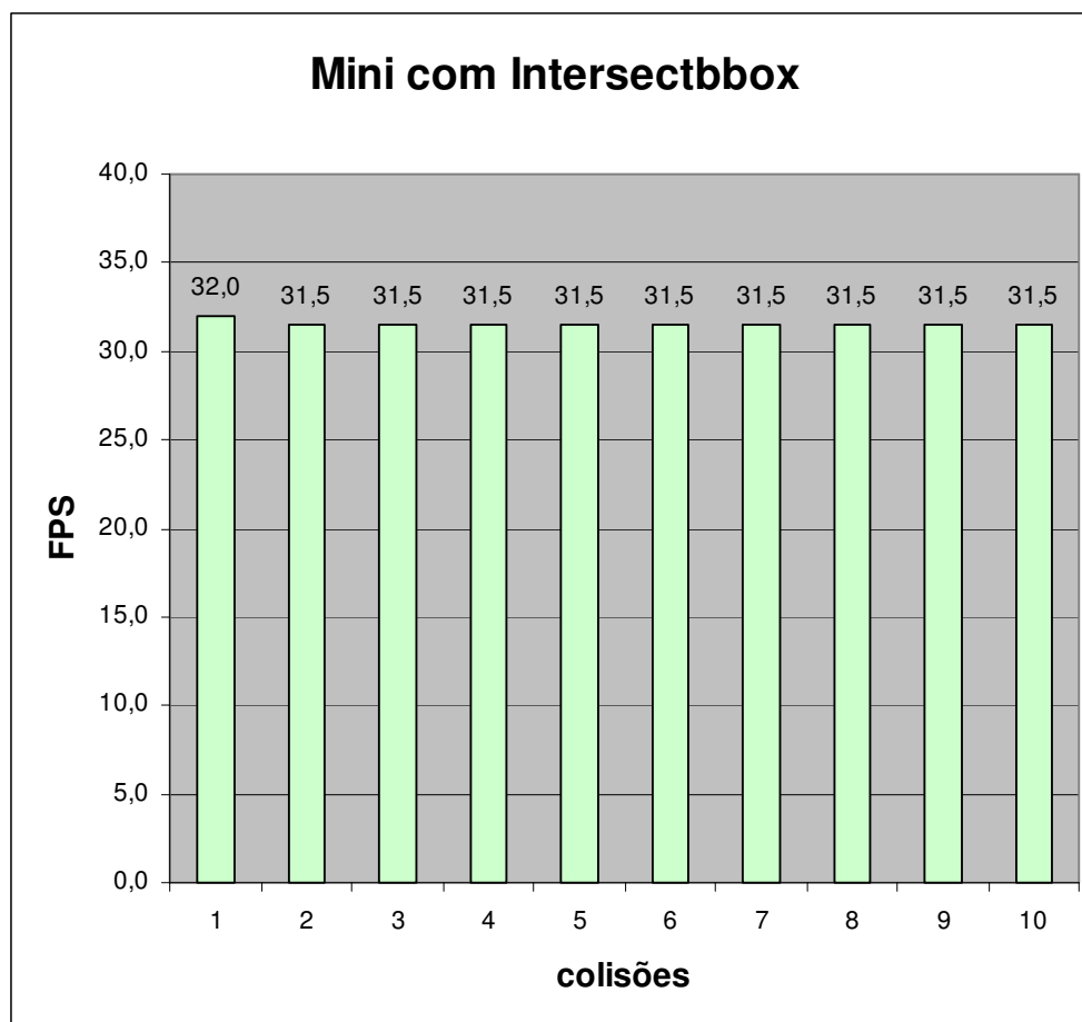
Figura 6.11 – FPS de 10 colisões com Intersectbbox do protótipo Mini
