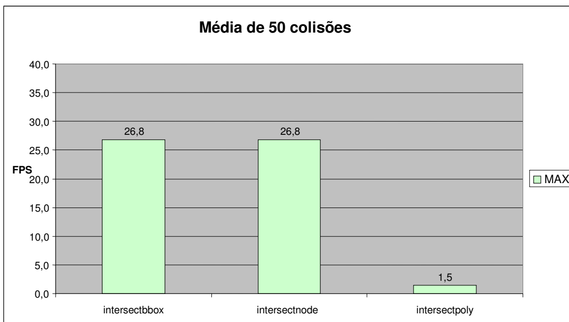
Figura 6.28 – Média de 50 colisões com o protótipo Max
