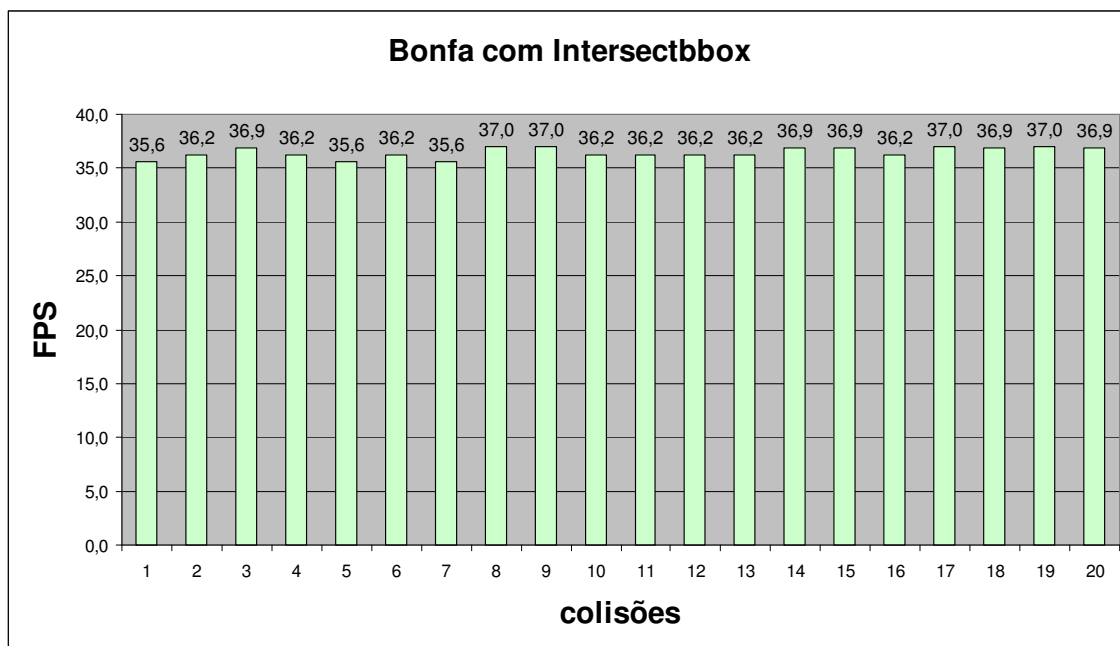
Figura 6.6 – FPS de 20 colisões com Intersectbbox do Protótipo Bonfa
