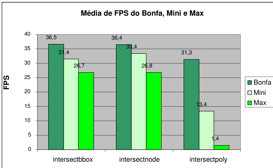
Figura 6.29 - Média geral dos FPS dos três avatares com 50 colisões
