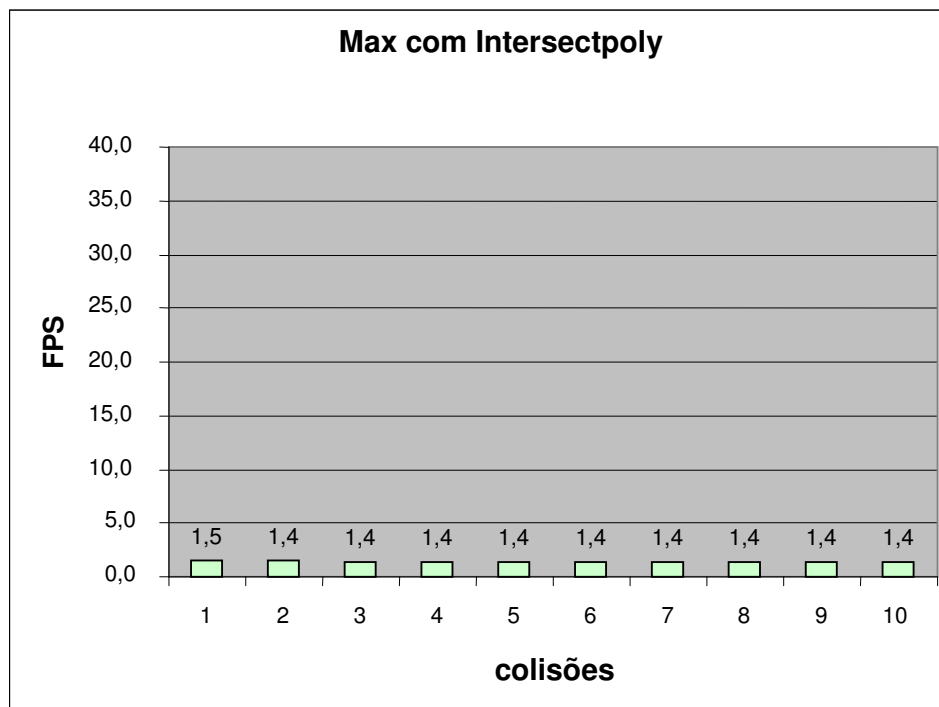
Figura 6.22 – FPS de 10 colisões com Intersectpoly do protótipo Max
