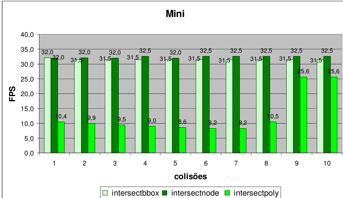
Figura 6.14 – FPS com 10 colisões entre as três técnicas do protótipo Mini
