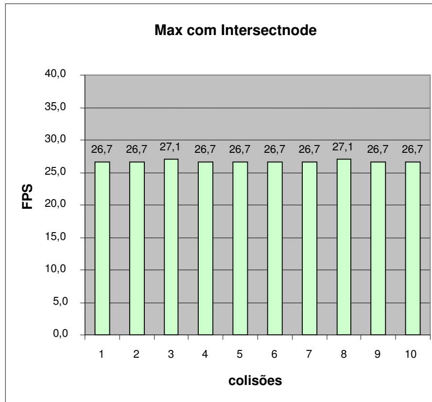
Figura 6.21 - FPS de 10 colisões com Intersectnode do protótipo Max
