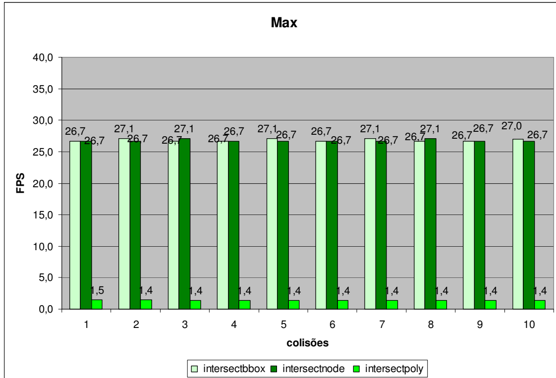
Figura 6.23 – FPS com 10 colisões entre as três técnicas com protótipo Max
