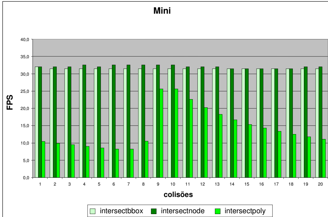
Figura 6.18 – FPS com 20 colisões entre as três técnicas com protótipo Mini
