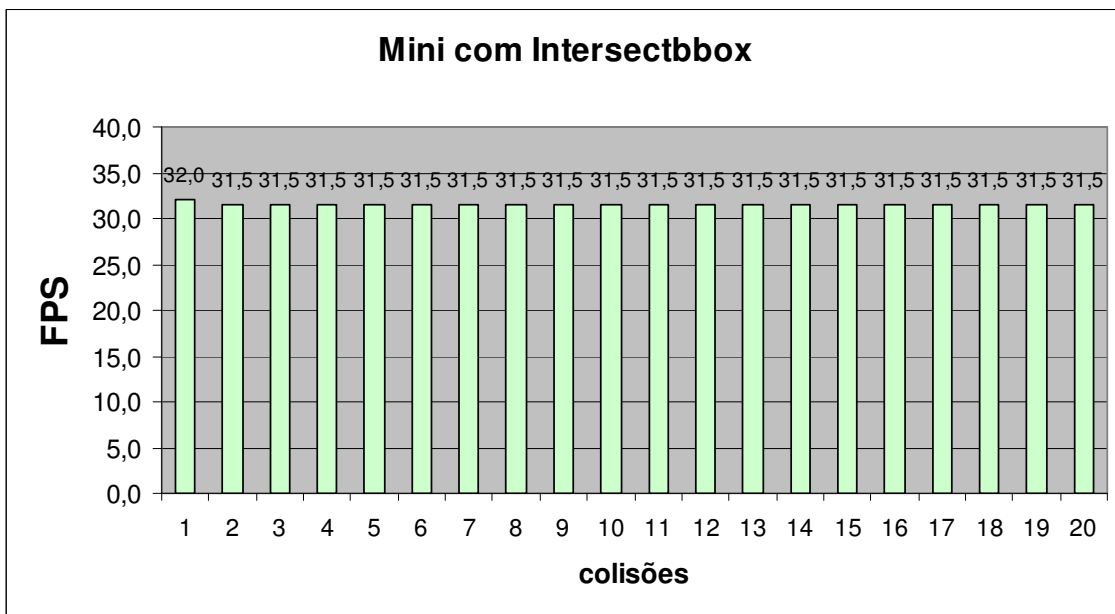
Figura 6.15 – FPS de 20 colisões com Intersectbbox do protótipo Mini
