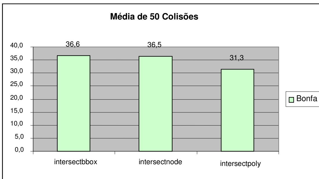
Figura 6.10 – Média de 50 colisões com o protótipo Bonfa
