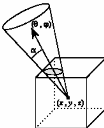
Figura 3.9. Obtenção do cone que define conjunto de movimentos das partículas de uma célula da grade pentadimensional (Steigleder, 1997).
