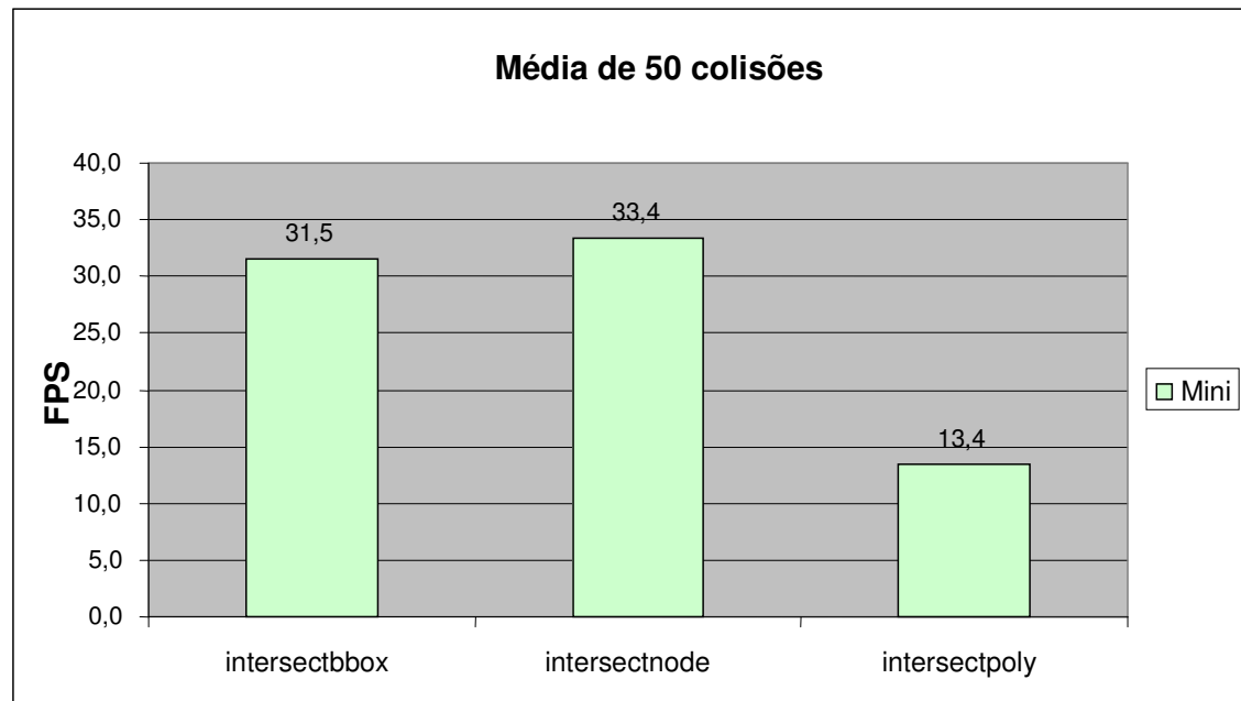
Figura 6.19 – Média de 50 colisões com o protótipo Mini
