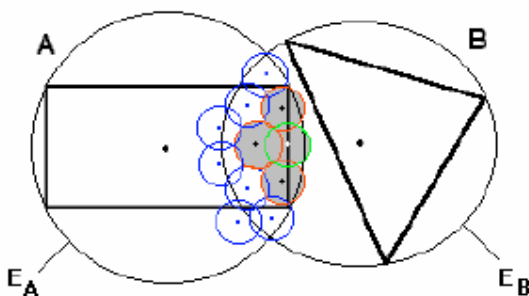
Figura 3.5 - Prováveis pontos de colisão
