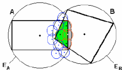
Figura 3.6 - Pontos de colisão (Nascimento, 2003)
