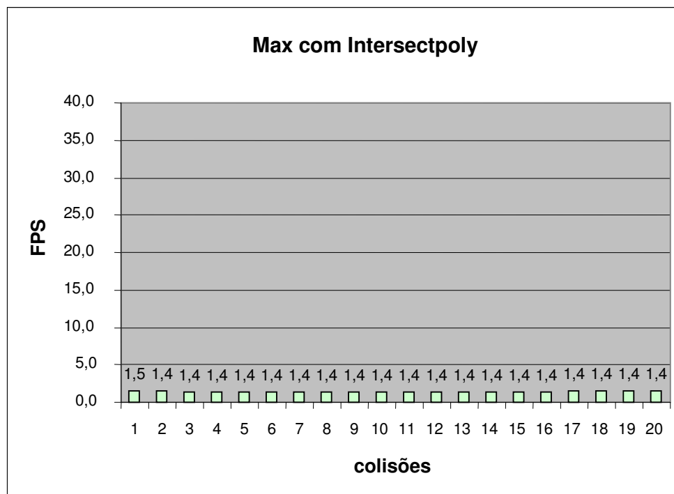
Figura 6.26 – FPS de 20 colisões com Intersectpoly do protótipo Max
