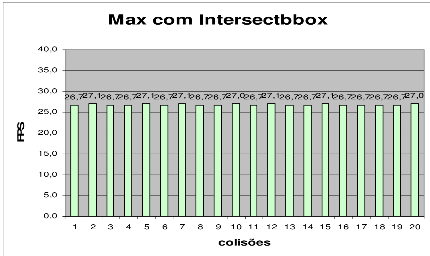
Figura 6.24 – FPS de 20 colisões com Intersectbbox do protótipo Max
