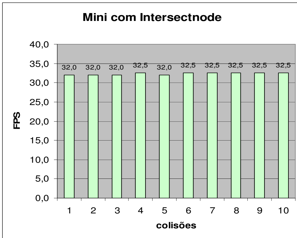
Figura 6.12 – FPS de 10 colisões com Intersectnode do protótipo Mini
