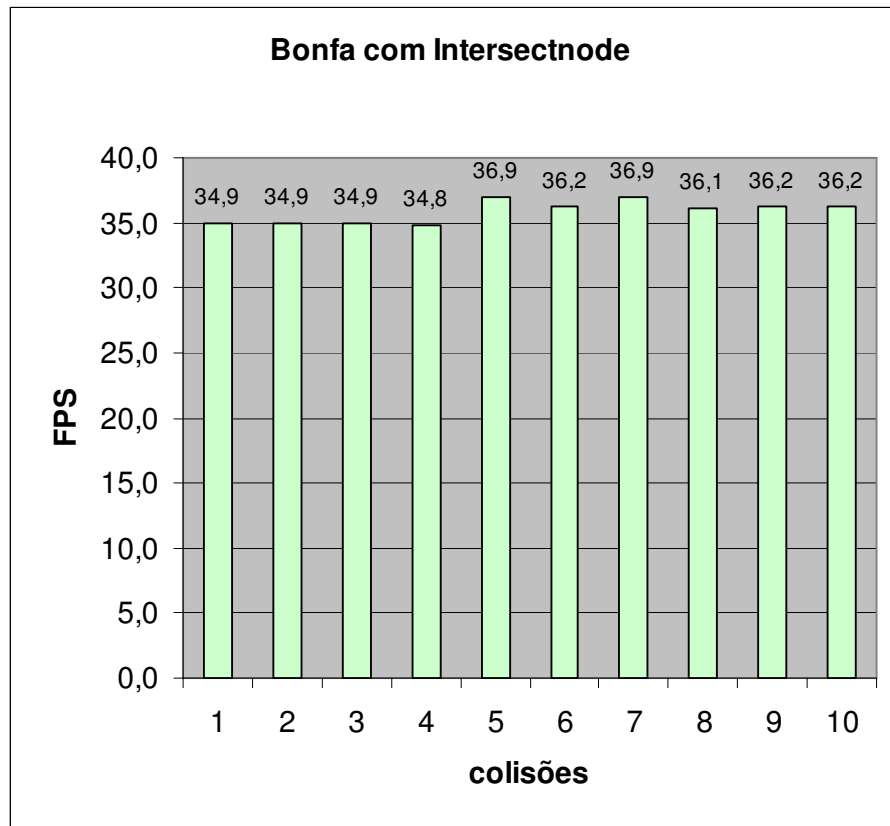
Figura 6.3 – FPS de 10 colisões com Intersectnode do protótipo Bonfa
