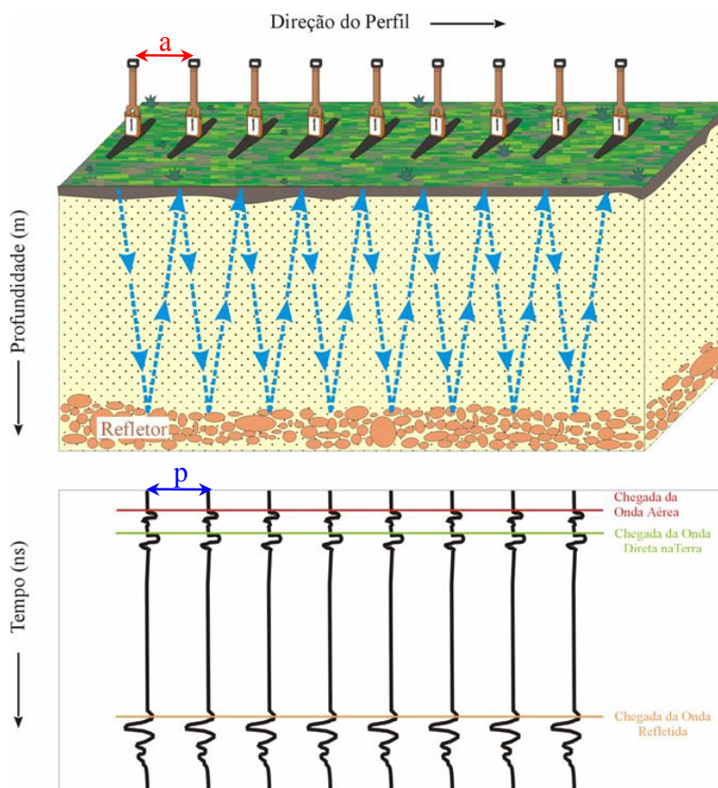
Figura 15 – Esquema de aquisição com GPR, no modo caminhamento, passo a passo ( p ), com afastamento constante. a) Procedimento envolvendo movimentos repetitivos das antenas transmissora e receptora, com espaçamento constante ( a ) entre as antenas; b) oito traços esquemáticos de GPR mostrando a chegada da onda aérea, da onda direta na terra e da onda refletida no substrato em subsuperfície. (modificado de BORGES, 2002).
