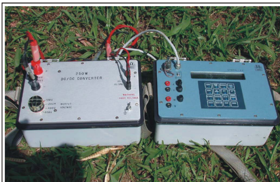
Figura 8 – Resistivímetro Syscal R2- Íris. À esquerda o conversor de corrente e à direita o console principal.
