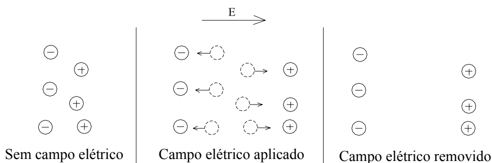
Figura 11 – Movimentação de cargas associada à corrente de condução (ANNAN, 1992).
