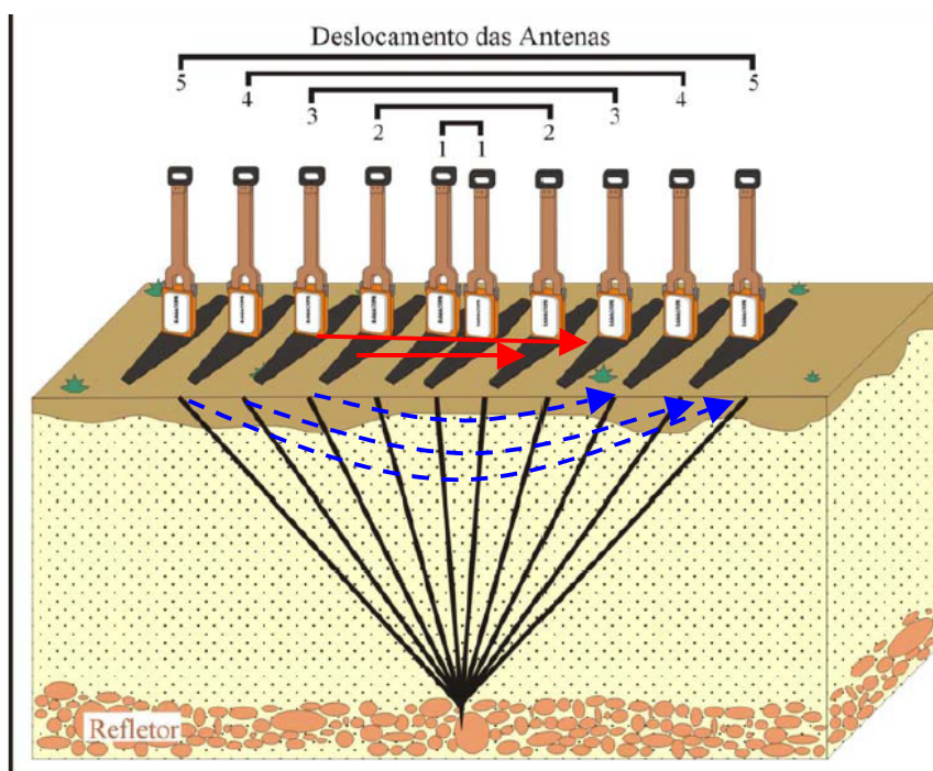
Figura 13 – Sondagem de velocidade do tipo CMP. À esquerda a antena transmissora e à direita a antena receptora. Os números acima indicam a posição seqüencial das antenas durante a aquisição. As linhas vermelhas indicam o caminho das ondas aéreas. As linhas azuis indicam o caminho das ondas diretas no solo. As linhas pretas representam o percurso das ondas refletidas no ponto comum. (Modificado de BORGES, 2002).
