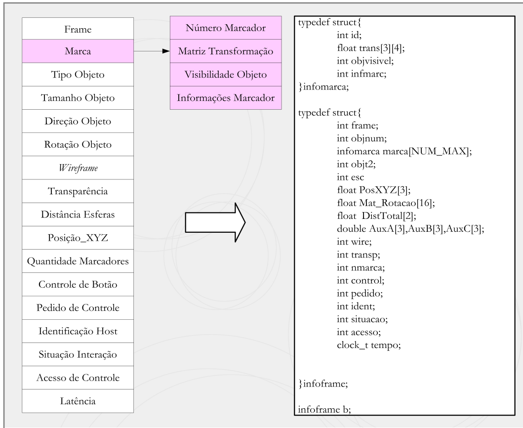
Figura 4.28: Formato da mensagem enviada pela aplicação servidora
