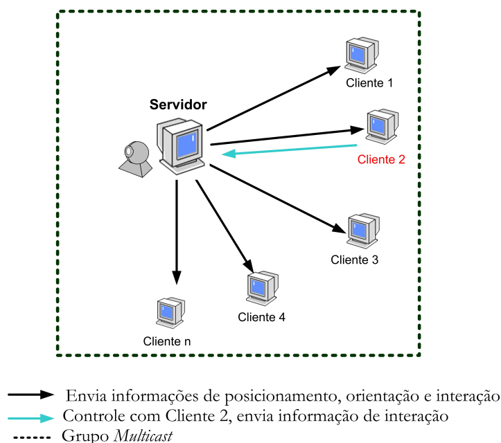
Figura 4.30: Aplicação de Realidade Aumentada Distribuída controle com o Cliente
