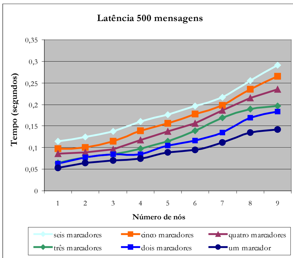
Figura 5.5: Latência para 500 mensagens
