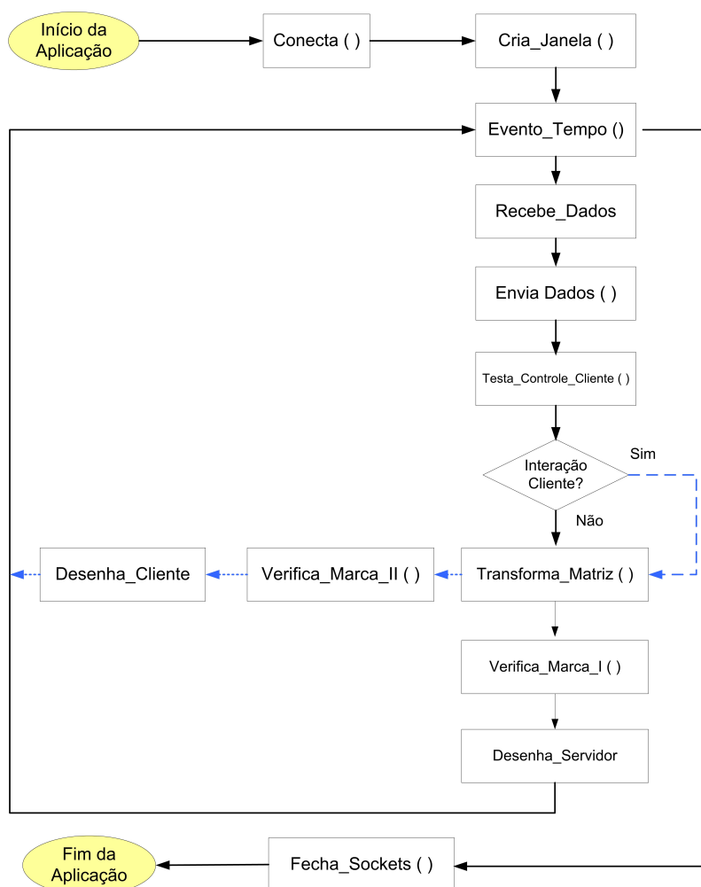
Figura 4.32: Diagrama da Aplicação Cliente
