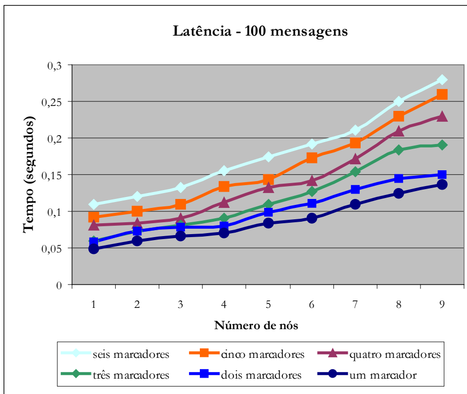
Figura 5.4: Latência para 100 mensagens
