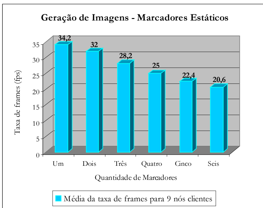
Figura 5.7: Geração de Imagens: Marcadores Estáticos
