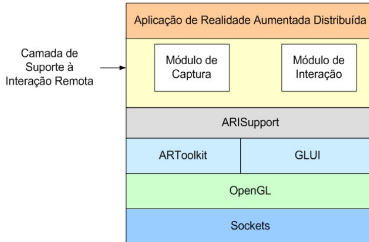
Figura 4.1: Diagrama da Arquitetura do Projeto
