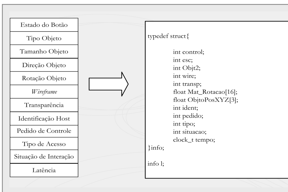
Figura 4.31: Formato da mensagem enviada pela aplicação cliente
