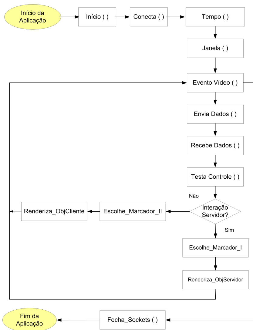
Figura 4.29: Diagrama da Aplicação Servidora
