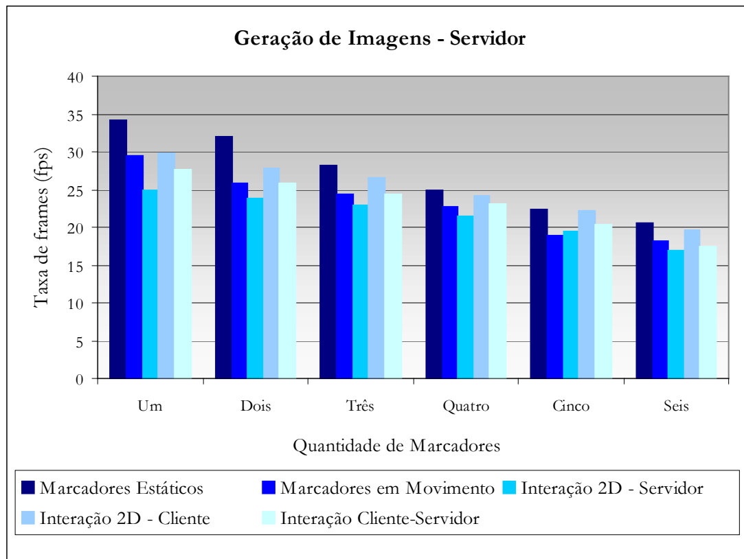
Figura 5.13: Geração de Imagens – Taxa de frames – Comparação I
