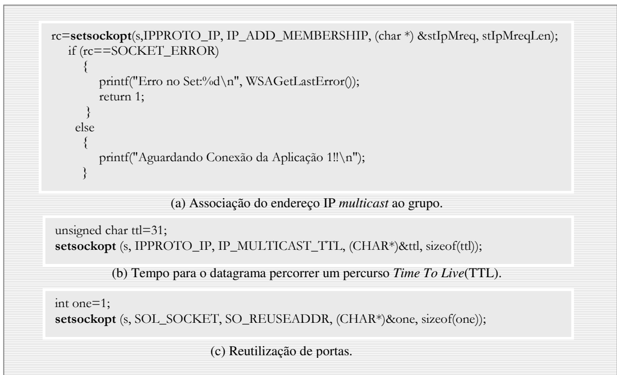
Figura 4.23: Demonstração da função setsockopt
