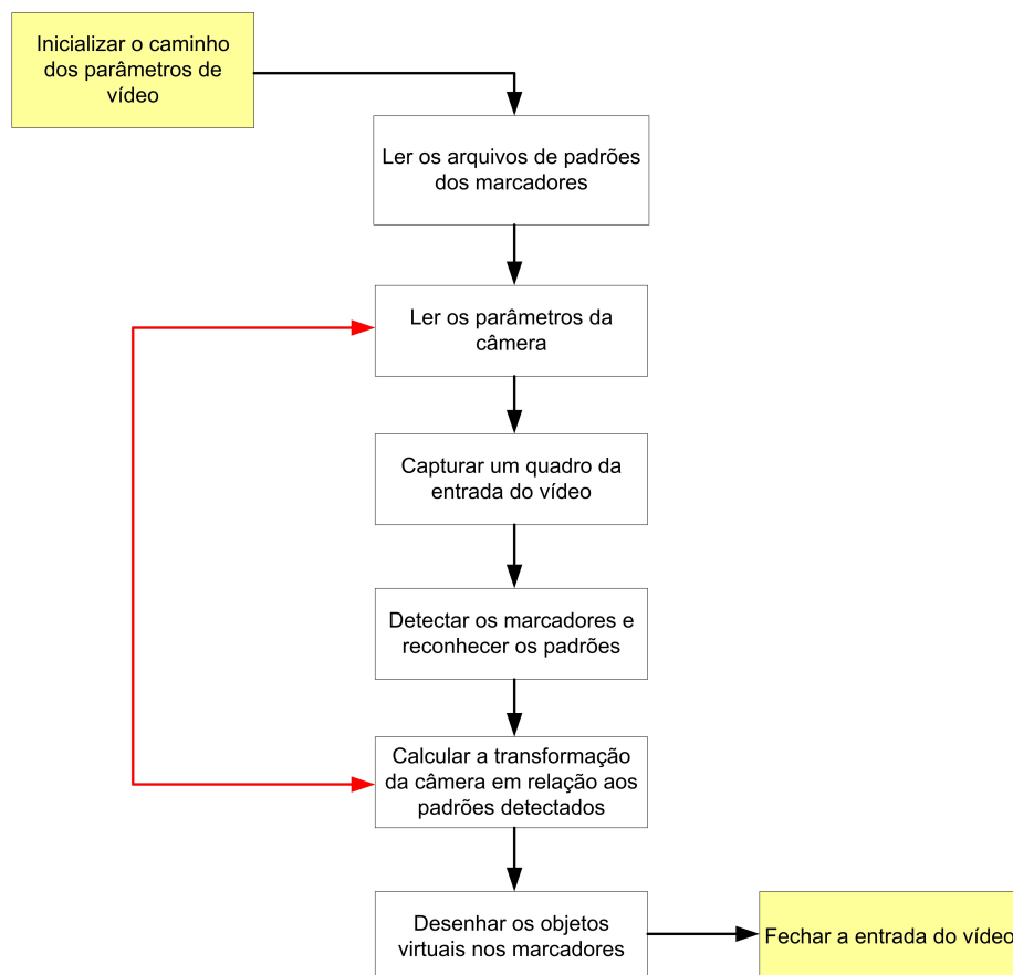
Figura 3.6: Etapas para o desenvolvimento de uma aplicação utilizando o ARToolkit
