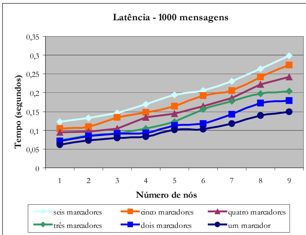
Figura 5.6: Latência para 1000 mensagens
