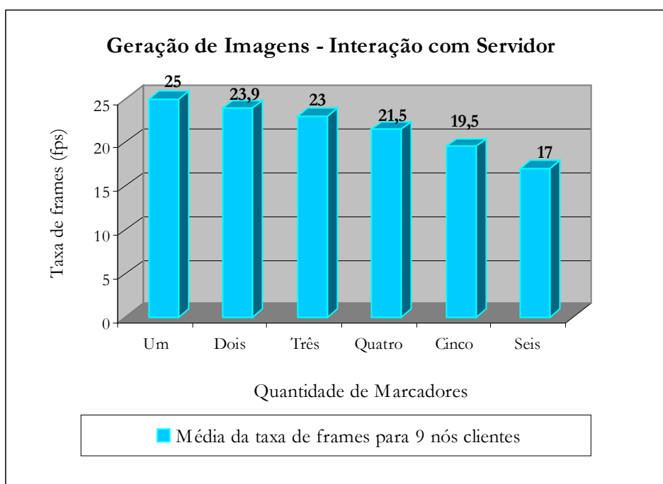
Figura 5.9: Geração de Imagens: Interação 2D Servidor
