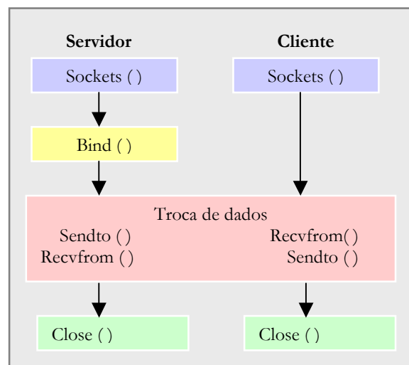
Figura 4.16: Utilização de Sockets UDP
