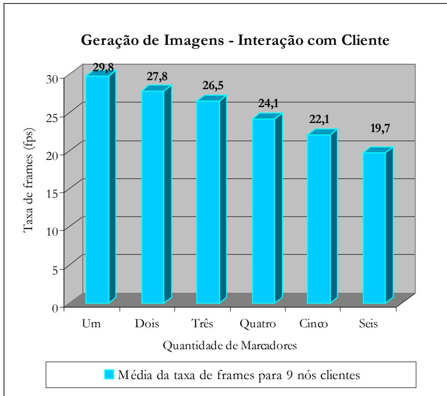
Figura 5.11: Geração de Imagens: Interação 2D - Cliente
