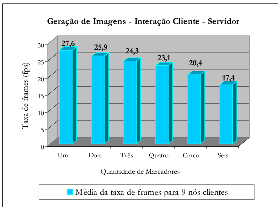
Figura 5.12: Geração de Imagens: Interação Cliente-Servidor
