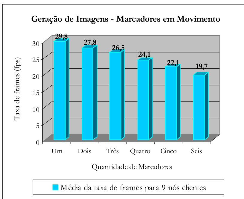
Figura 5.8: Geração de Imagens: Marcadores em Movimento
