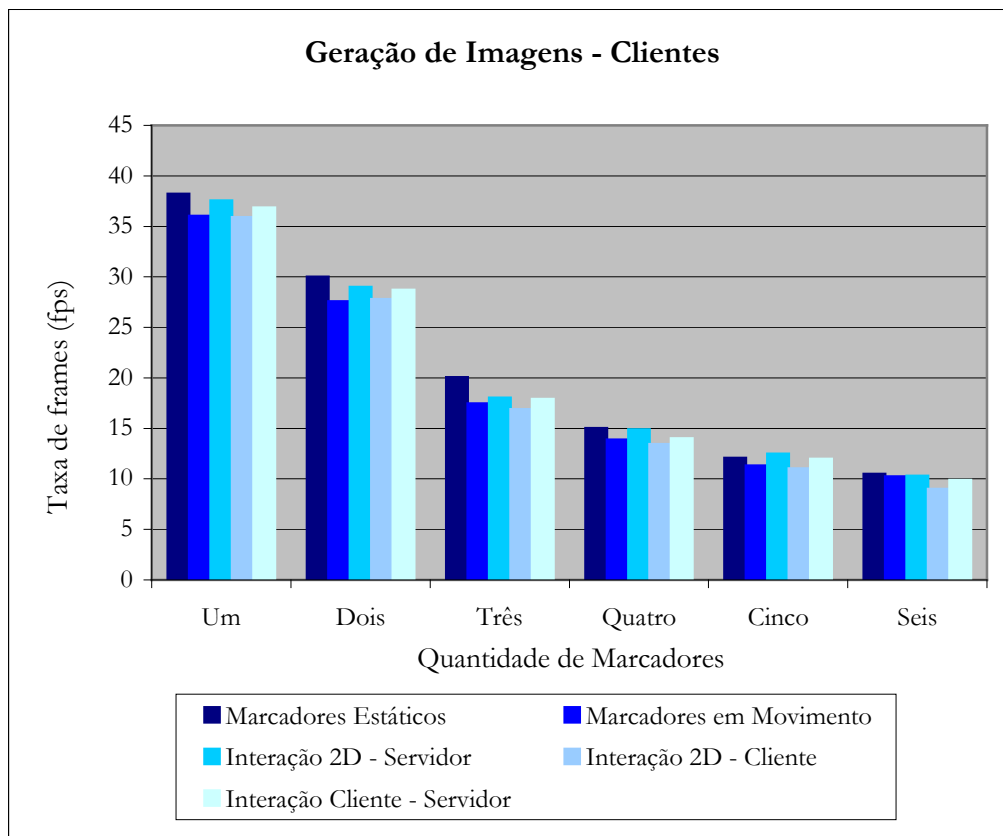
Figura 5.14: Geração de Imagens – Taxa de frames – Comparação II
