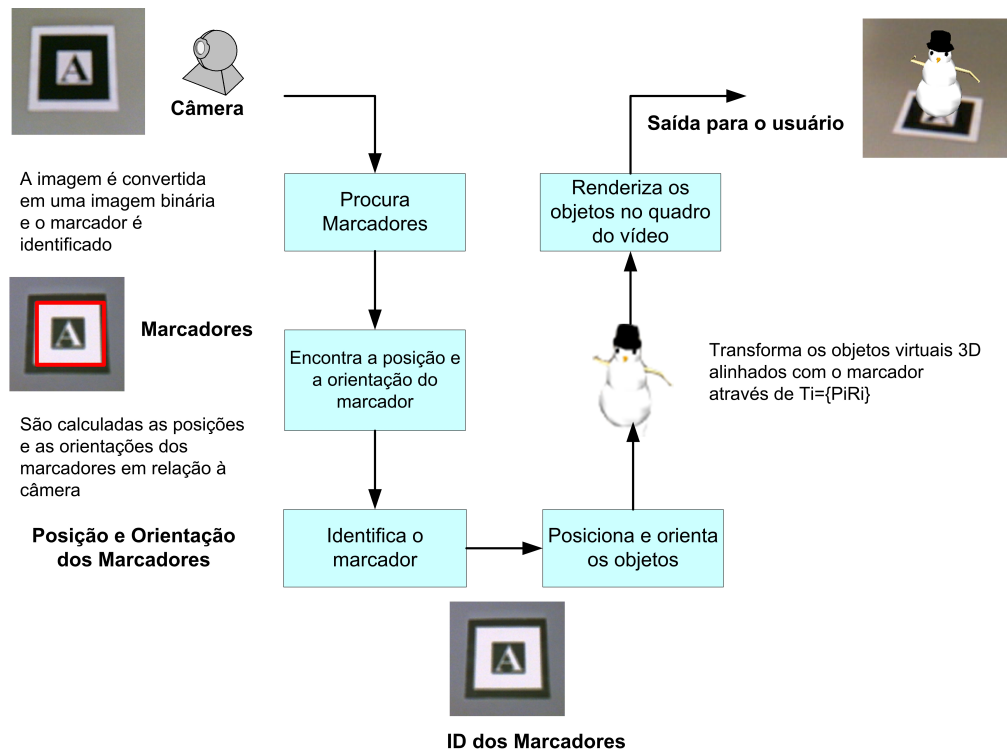
Figura 3.5: Técnicas de Rastreamento e Registros
