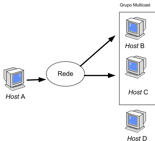
Figura 3.4: Modelo de Comunicação Multicast
