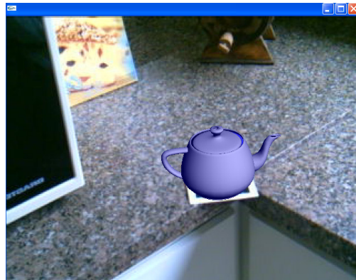
Figura 2.2: Realidade Aumentada
