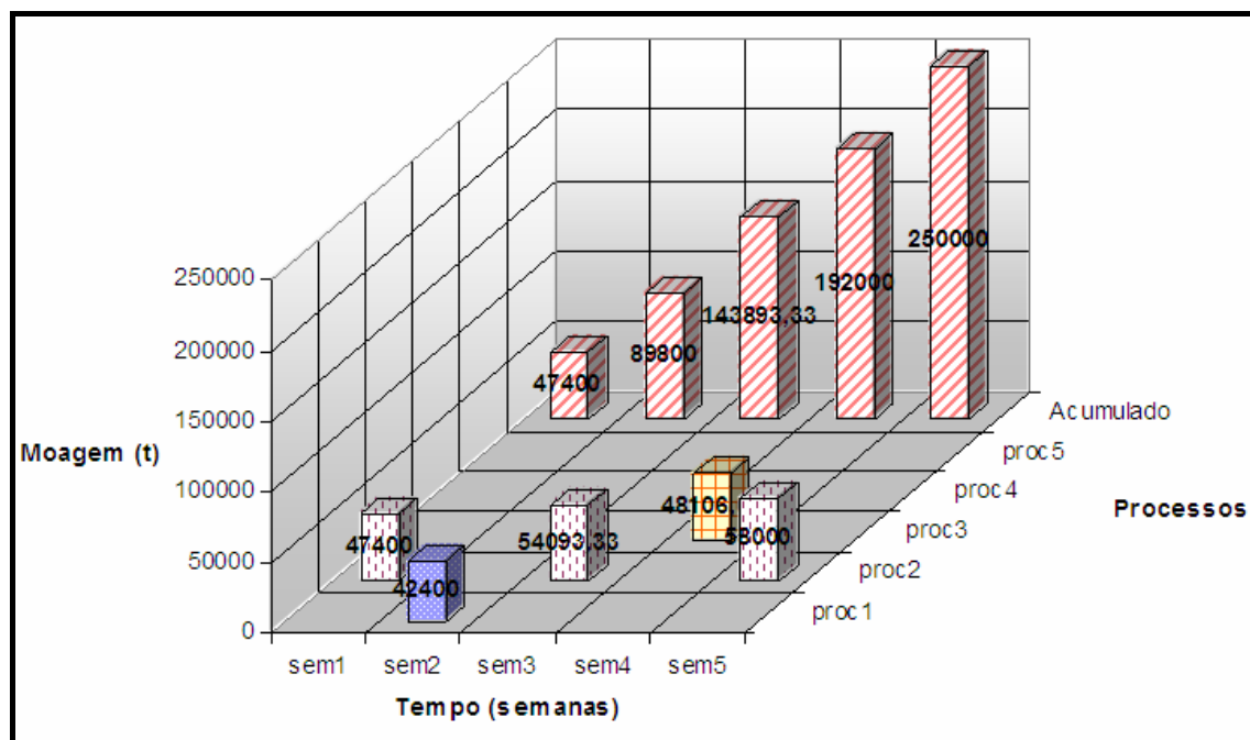
Figura 13. Plano de produção encontrado para o cenário IV
