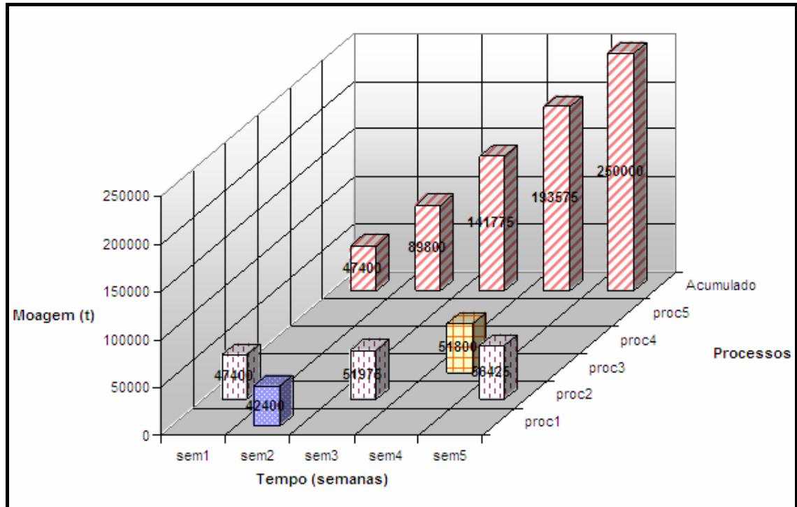
Figura 14. Plano de produção encontrado para o cenário V
