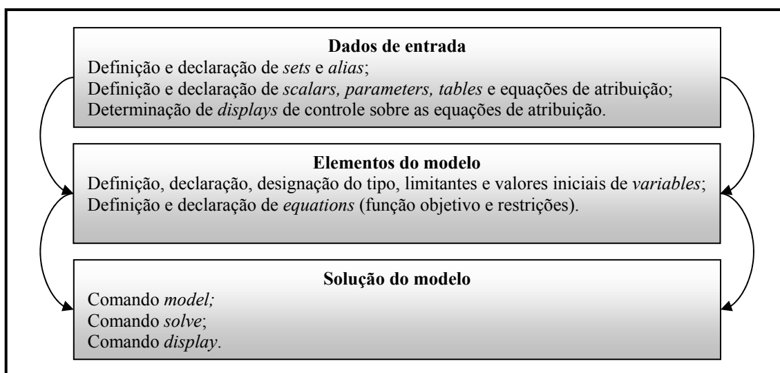
Figura 31. Estrutura geral do modelo GAMS (Fonte: adaptada de Brooke et al. , 1997)
