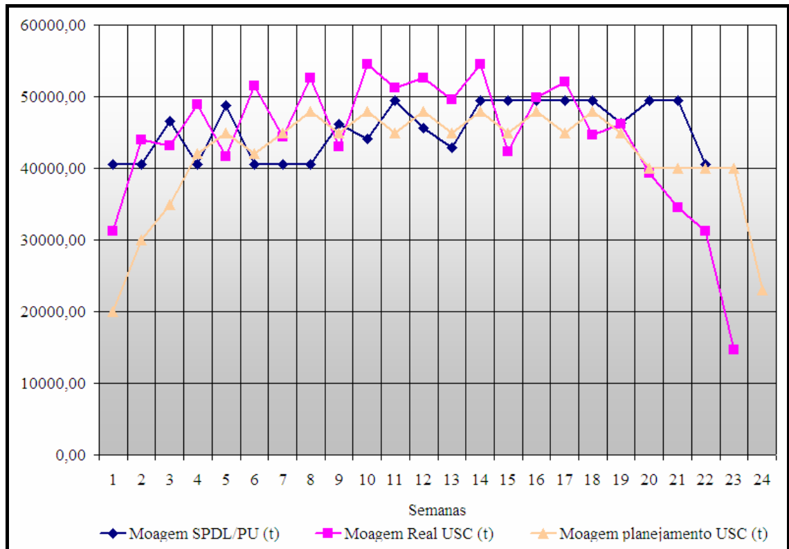
Figura 19. Evolução e comparação da moagem durante a safra (cenário preliminar)
