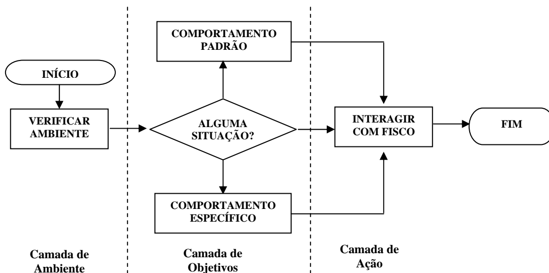
Figura 9 - Arquitetura detalhada utilizada para simulação
