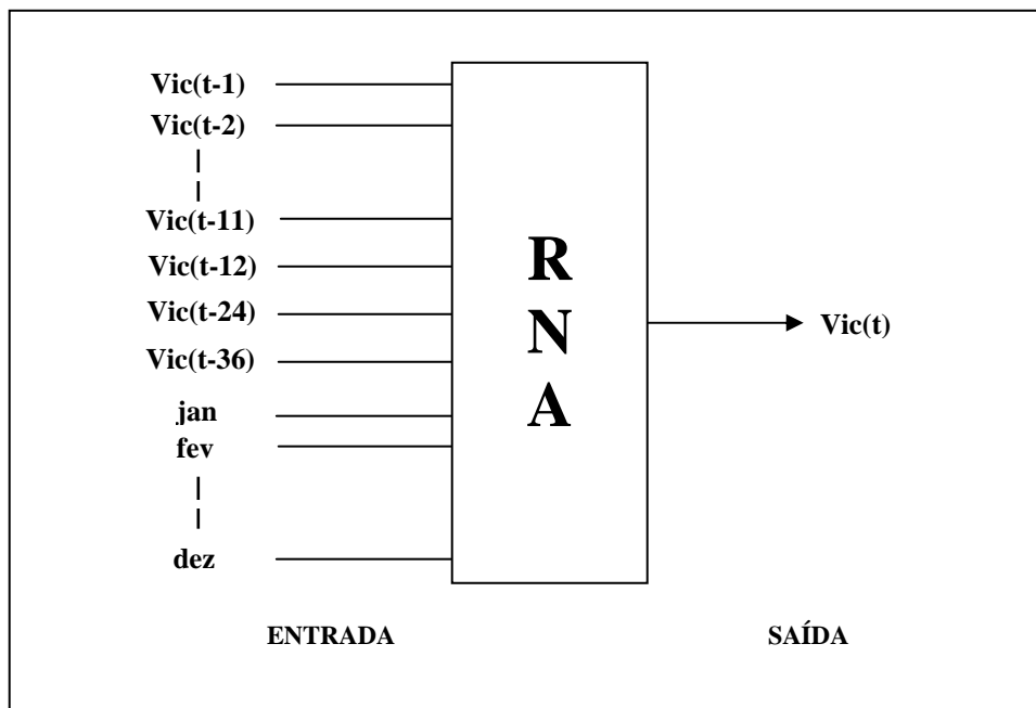
Figura 12 - RNA utilizada no módulo neural de previsão
