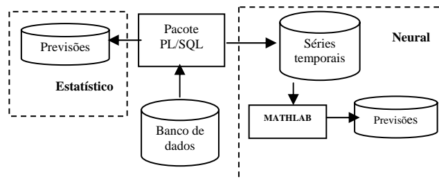
Figura 11 - Arquitetura de implementação do sistema de previsão comportamental
