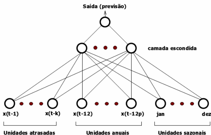
Figura 6 - Topologia de RNA para previsão segundo Varfis e Versino
