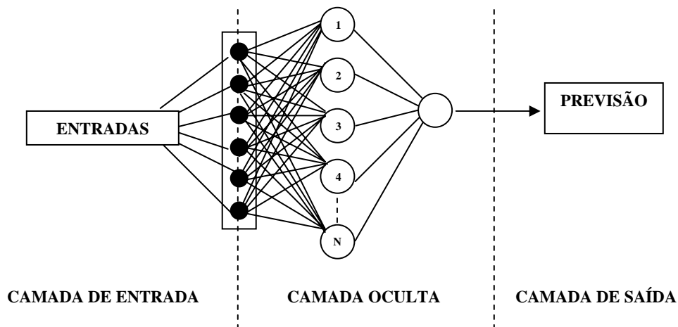
Figura 5 – Topologia genérica de RNA para previsão
