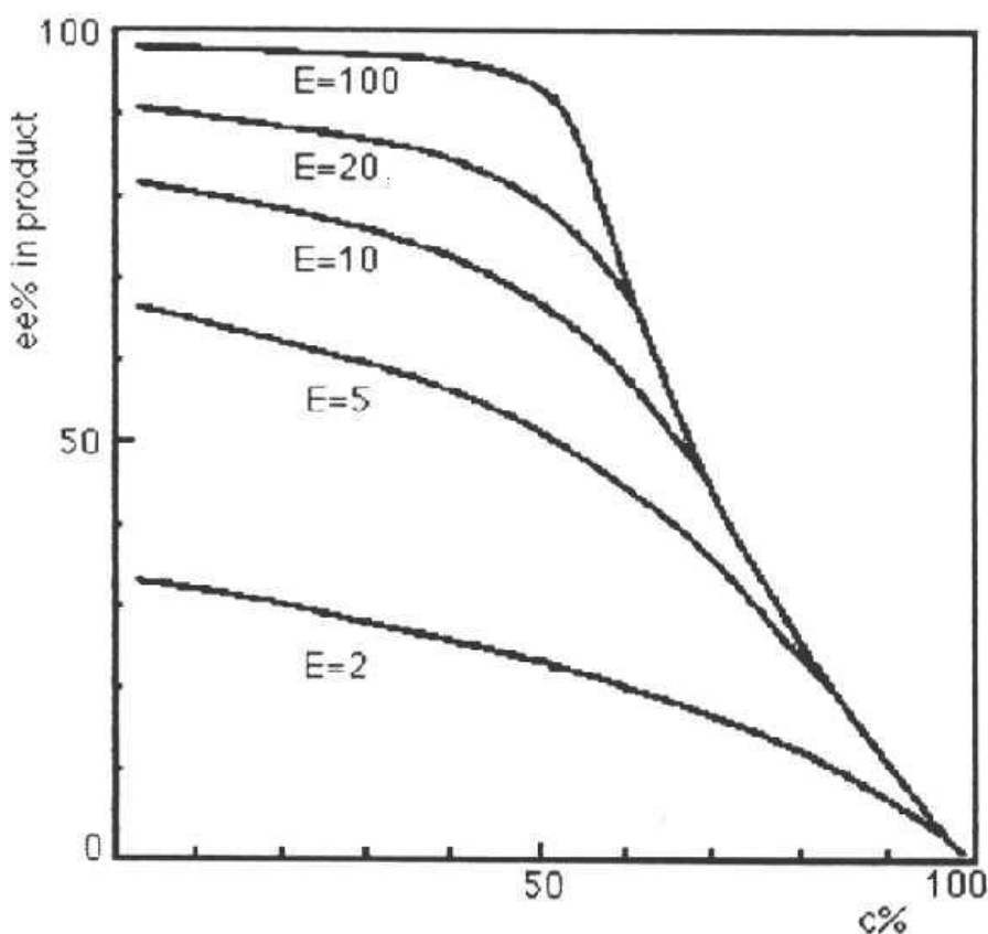
Figura 21. Superfície simulada do excesso enantiomérico versus grau de conversão em uma resolução cinética
