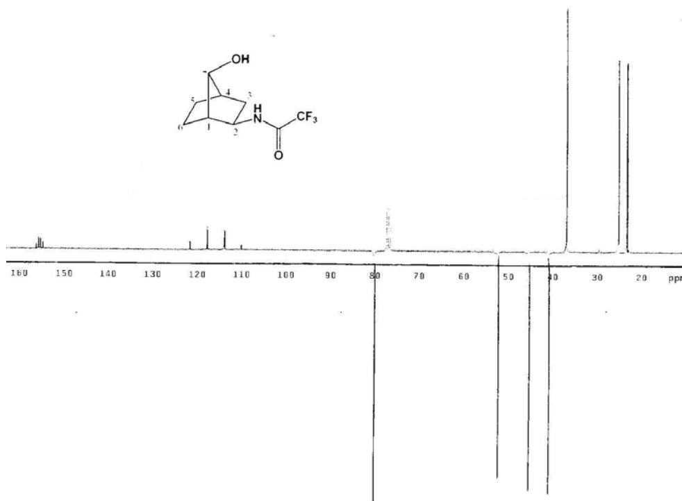
Figura 70. Espectro de RMN de ^{13}\text{C} (APT) do composto syn -( \pm )- 81 ( \text{CDCl}_3 , 75 MHz)
