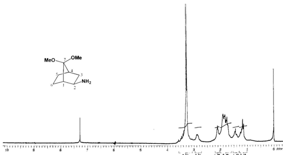
Figura 63. Espectro de RMN de ^1\text{H} da amina ( \pm )- 78 ( \text{CDCl}_3 , 300 MHz)
