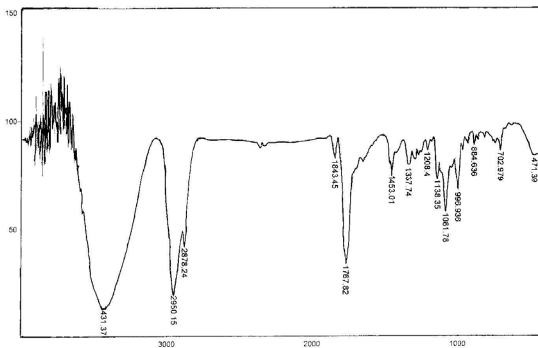
Espectro 6. Espectro de infra vermelho do ceto álcool 68
