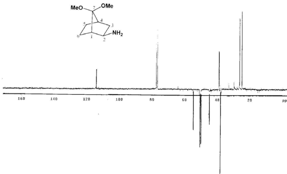
Figura 64. Espectro de RMN de ^{13}\text{C} (APT) da amina ( \pm )- 78 ( \text{CDCl}_3 , 75 MHz)
