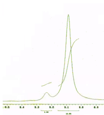
Figura 29 (b). Ampliação da região correspondente aos hidrogênios enantioméricos do composto (+)- 60 .
