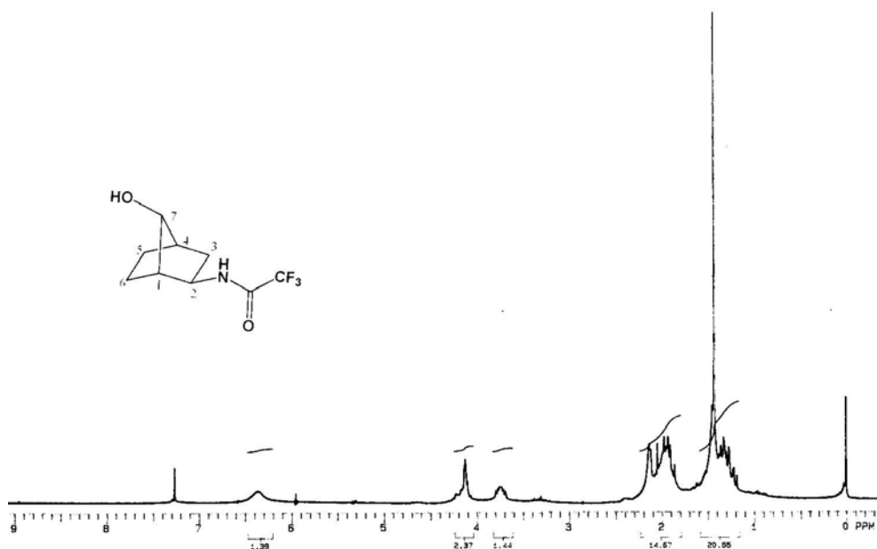
Figura 71. Espectro de RMN de ^1\text{H} do composto anti -( \pm )- 81 (CDCl 3 , 200 MHz)
