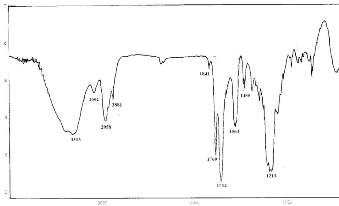
Espectro14. Espectro de infra vermelho da ceto trifluoroacetamida 80
