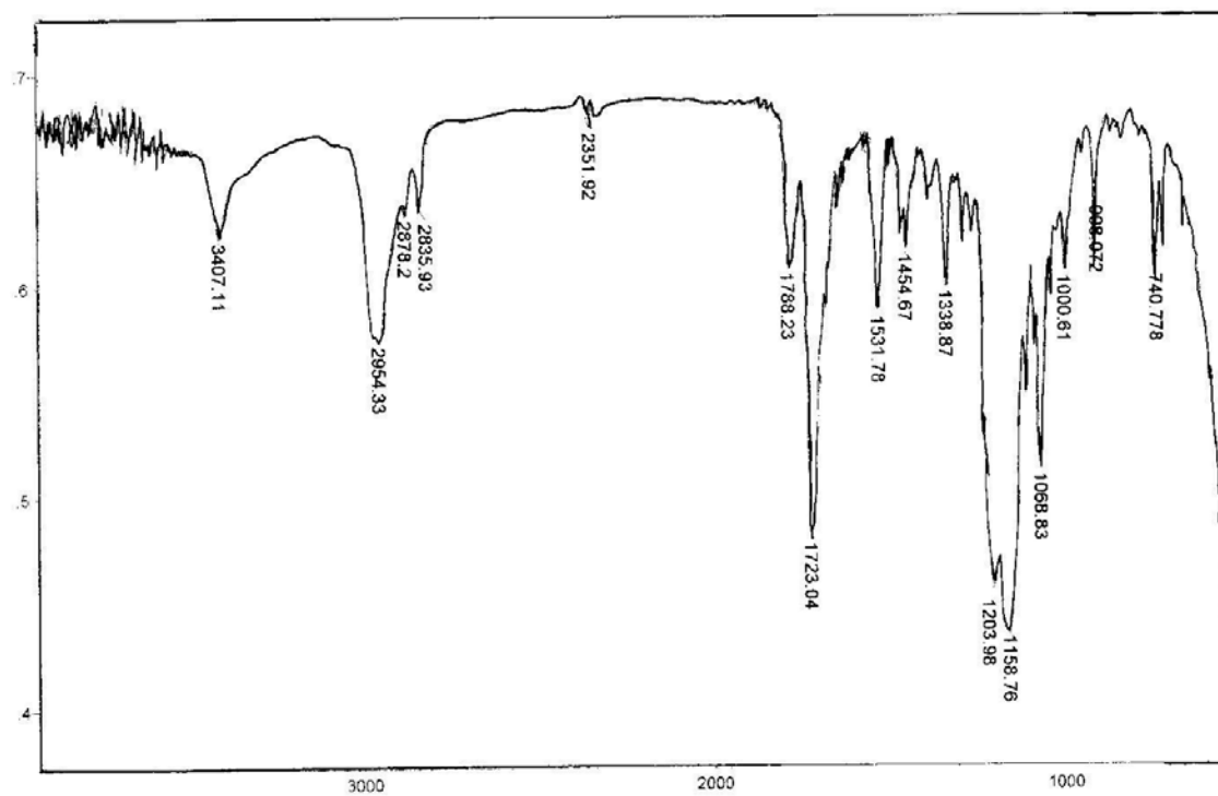
Espectro 13. Espectro de infra vermelho da trifluoroacetamida 79
