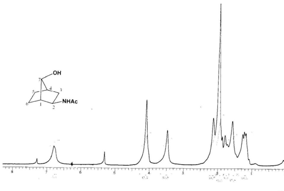
Figura 92. Espectro de RMN de ^1\text{H} do composto (+)- 90 ( \text{CDCl}_3 , 200 MHz)
