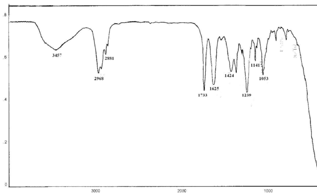
Espectro 21. Espectro de infra vermelho do composto (+)-85
