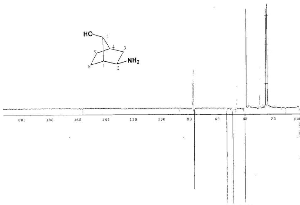
Figura 76. Espectro de RMN de 13 C (APT) do composto anti -(±)- 81 (CDCl 3 , 75 MHz)
