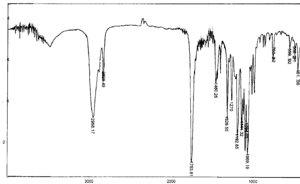
Espectro 4. Espectro de infra vermelho da cetona 66
