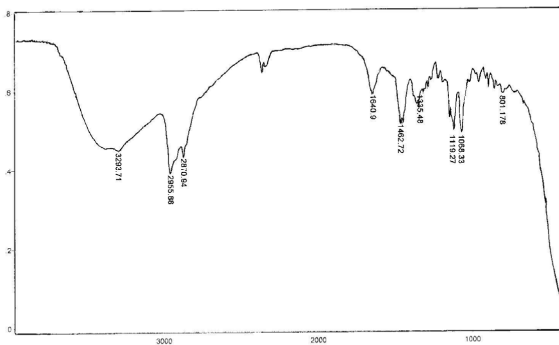
Espectro 20. Espectro de infra vermelho do composto (-)-84
