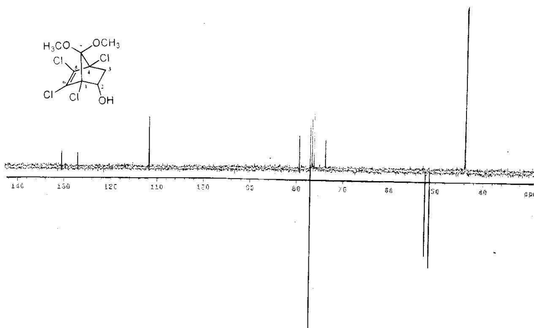
Figura 37. Espectro de RMN de ^{13}\text{C} (APT) do álcool ( \pm )-40 ( \text{CDCl}_3 , 50 MHz).
