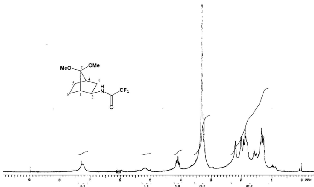
Figura 65. Espectro de RMN de ^1\text{H} da trifluoracetamida ( \pm )-79 ( \text{CDCl}_3 , 200 MHz)
