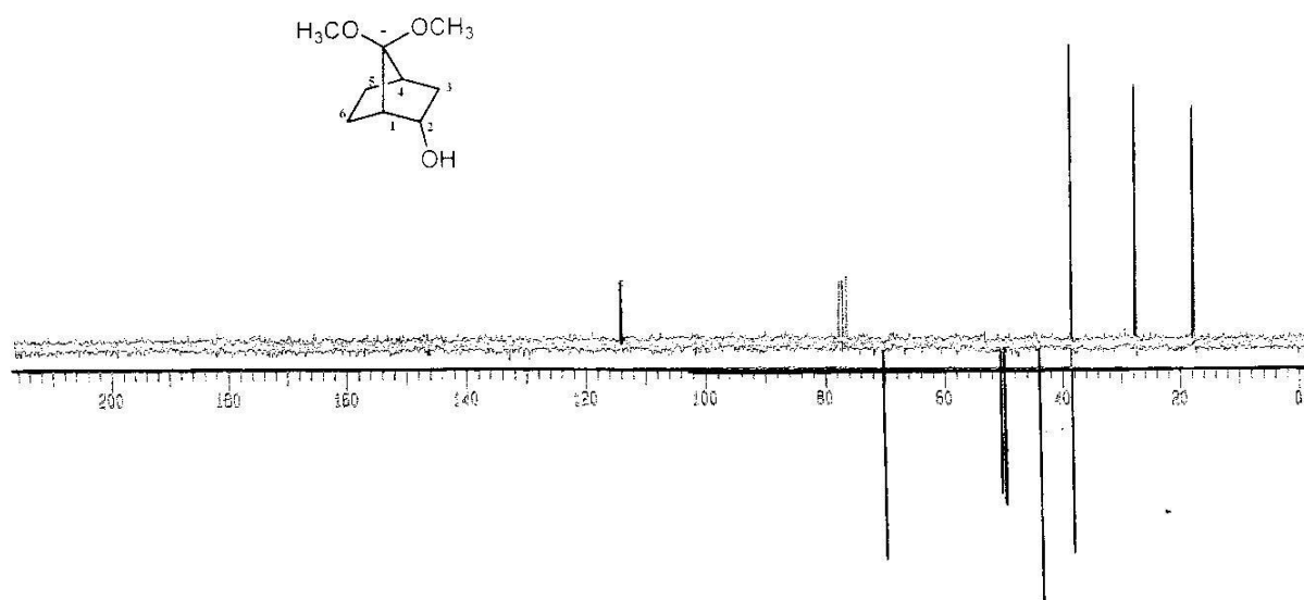
Figura 43. Espectro de RMN de ^{13}\text{C} (APT) do composto ( \pm )- 65 ( \text{CDCl}_3 , 50 MHz)
