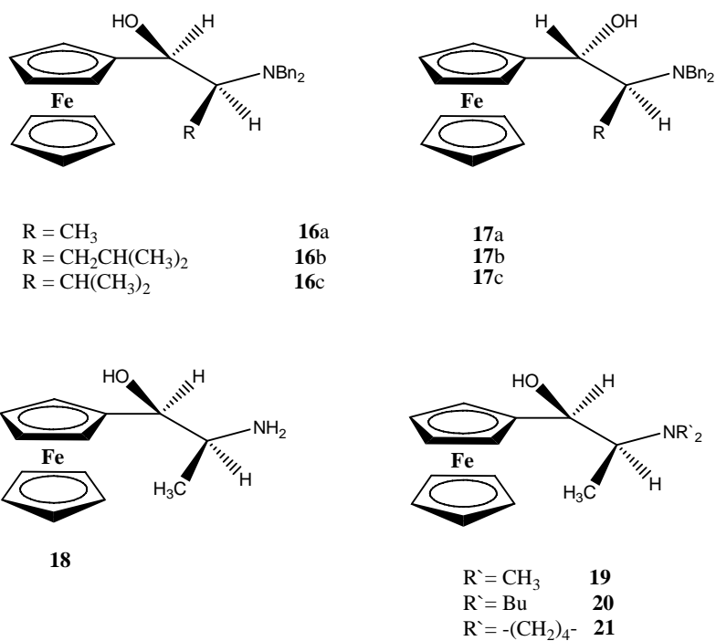
Figura 4. Aminoálcoois derivados do ferroceno
