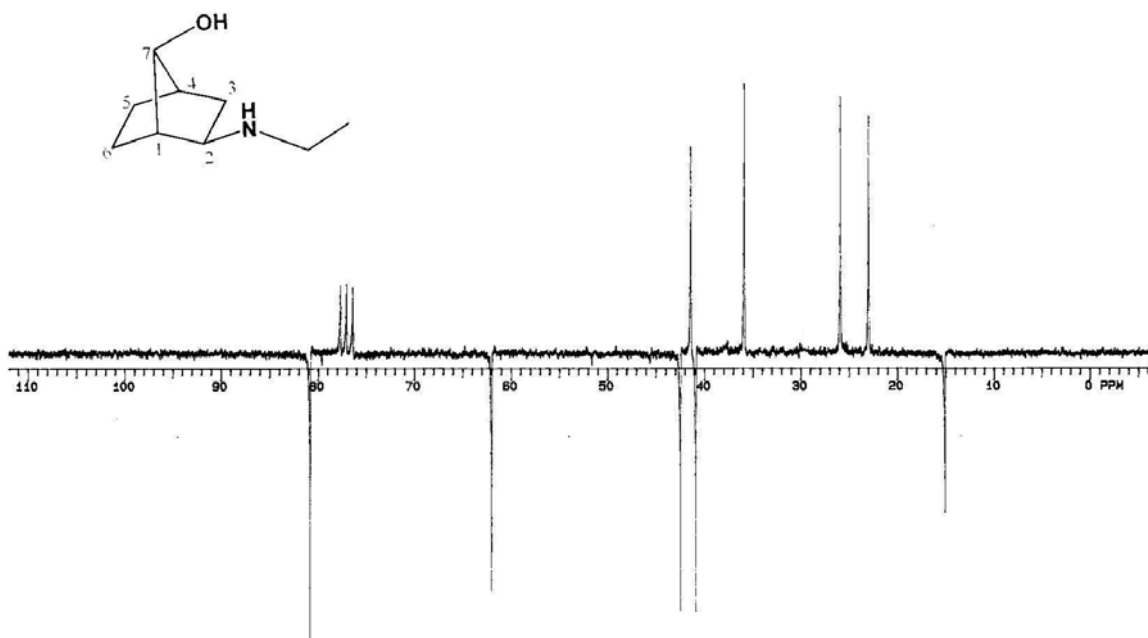
Figura 81. Espectro de RMN de ^{13}\text{C} (APT) do composto (-)- 84 ( \text{CDCl}_3 , 50 MHz)
