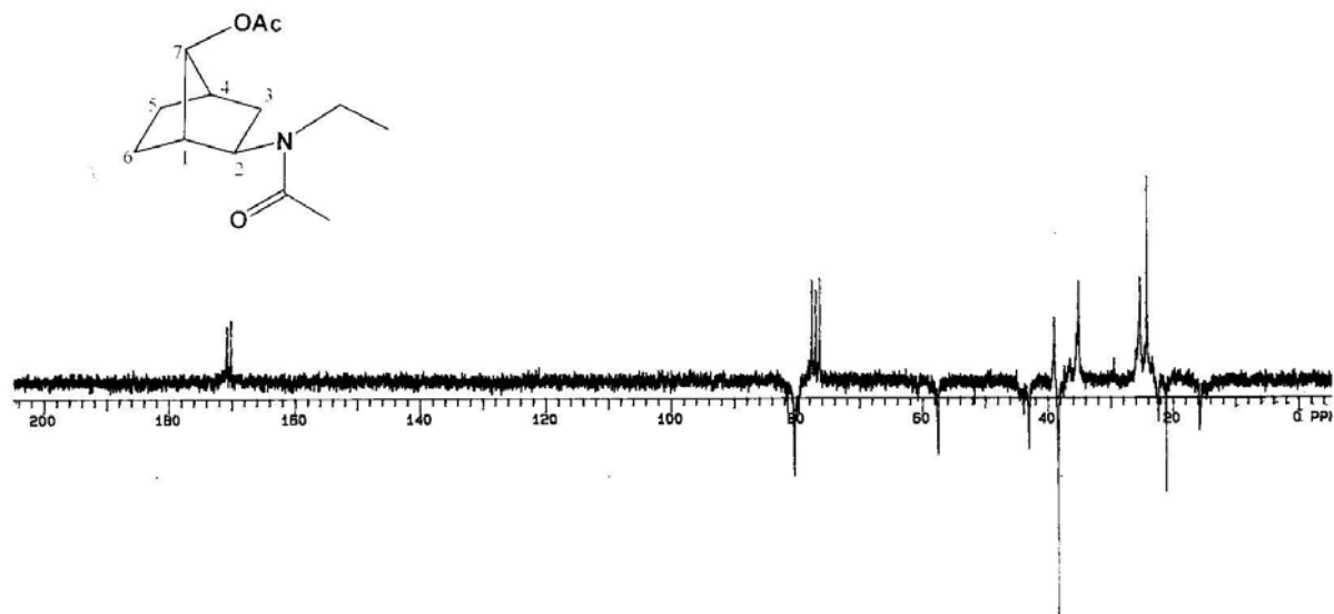
Figura 83. Espectro de RMN de ^{13}\text{C} (APT) do composto (+)- 85 ( \text{CDCl}_3 , 50 MHz)
