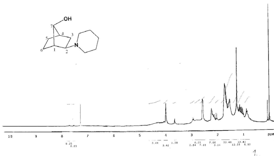
Figura 88. Espectro de RMN de ^1\text{H} do composto (-)- 89 ( \text{CDCl}_3 , 300 MHz)
