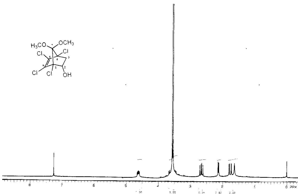
Figura 36. Espectro de RMN de ^1\text{H} do álcool ( \pm )-40 ( \text{CDCl}_3 , 200 MHz).
