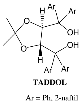
Figura 10. Estrutura básica do TADDOL
