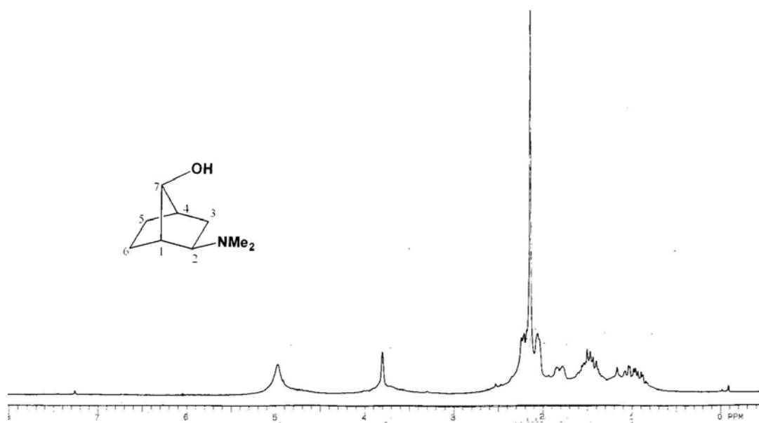
Figura 86. Espectro de RMN de 1 H do composto (-)- 87 (CDCl 3 , 200 MHz)
