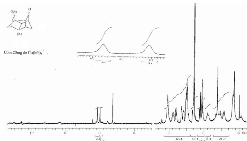
Figura 26. Espectro de RMN de ^1\text{H} do composto (\pm) - 60 com 20 mg de reagente de deslocamento químico quiral \text{Eu}(\text{hfc})_3 ( \text{CDCl}_3 , 300 MHz).
