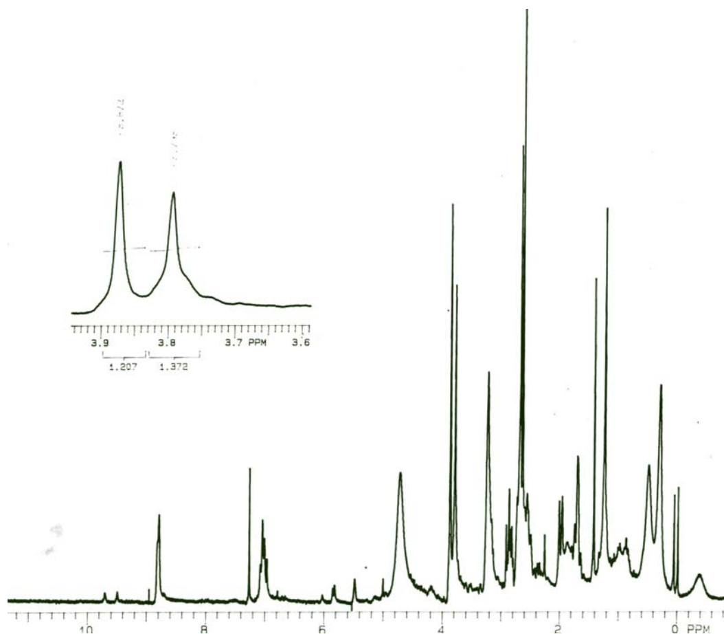
Figura 33. Espectro de RMN de ^1\text{H} do diacetato 61 , derivado do diol obtido com a redução de (-) - 60 , com 35 mg de reagente de deslocamento químico quiral \text{Eu}(\text{hfc})_3 ( \text{CDCl}_3 , 200 MHz).
