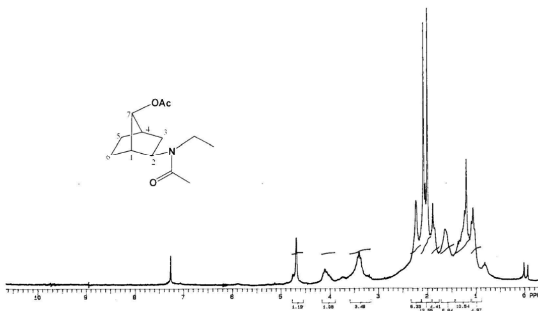
Figura 82. Espectro de RMN de 1 H do composto (+)- 85 (CDCl 3 , 200 MHz)
