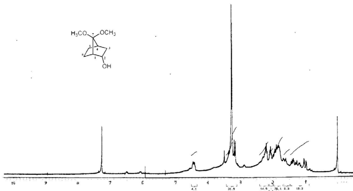
Figura 42. Espectro de RMN de ^1\text{H} do composto ( \pm )- 65 ( \text{CDCl}_3 , 200 MHz)
