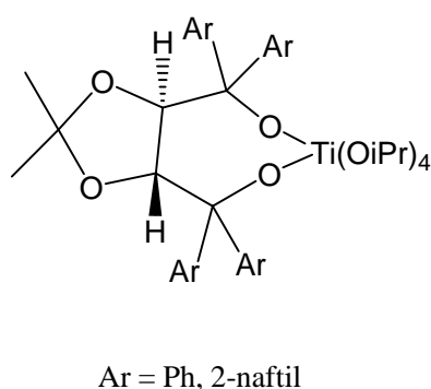
Figura 11. Complexo de titânio derivado do TADDOL
