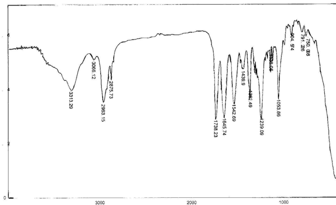
Espectro 19. Espectro de infra vermelho do composto (+)-83
