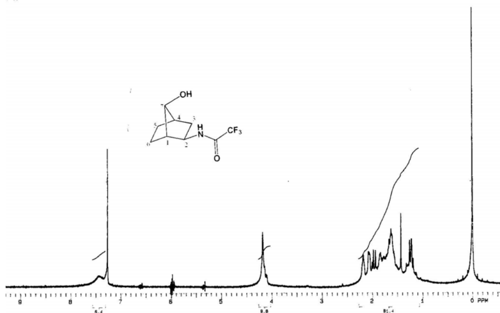
Figura 69. Espectro de RMN de ^1\text{H} do composto syn -( \pm )- 81 ( \text{CDCl}_3 , 200 MHz)
