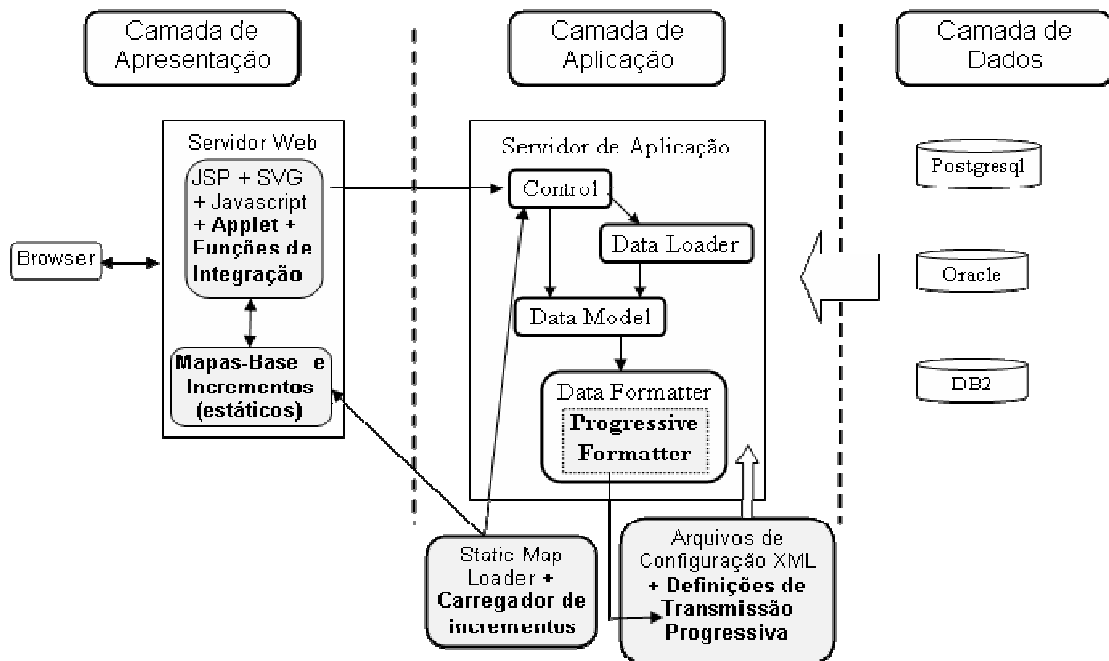
Figura 5.16. Arquitetura do iGIS com módulo de Transmissão Progressiva.
