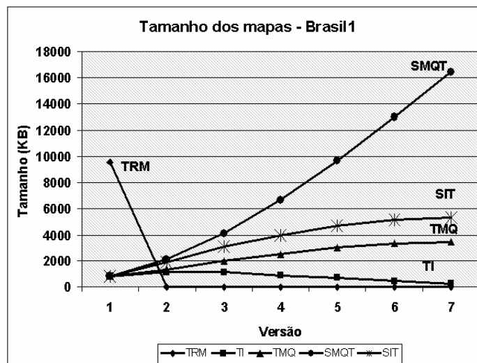
Figura 6.2. Gráfico comparativo para o mapa Brasil1
