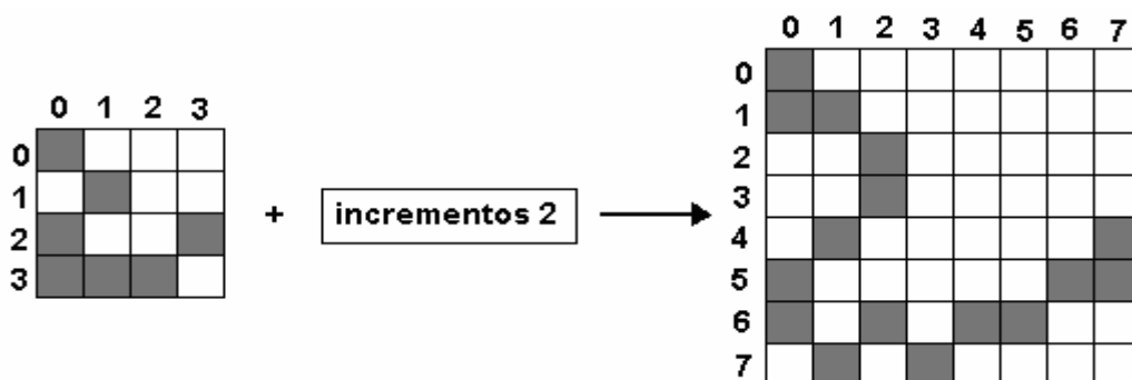
Figura 5.5. Reconstituição da Versão 3 do mapa.
