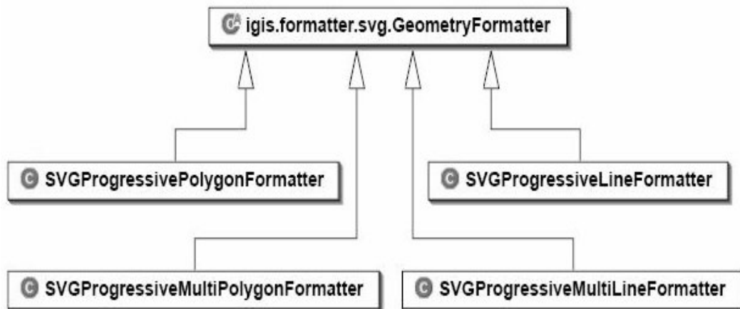
Figura 5.12. Classes formatadoras de geometrias.
