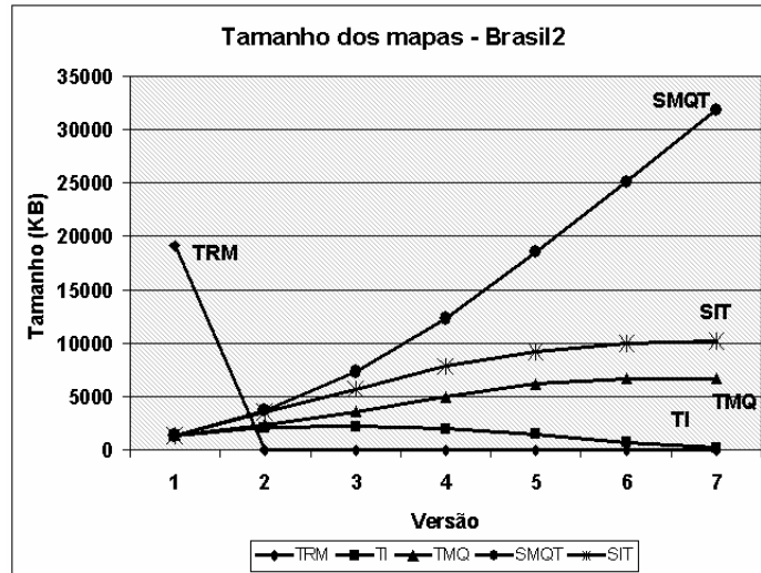
Figura 6.3. Gráfico comparativo para o mapa Brasil2
