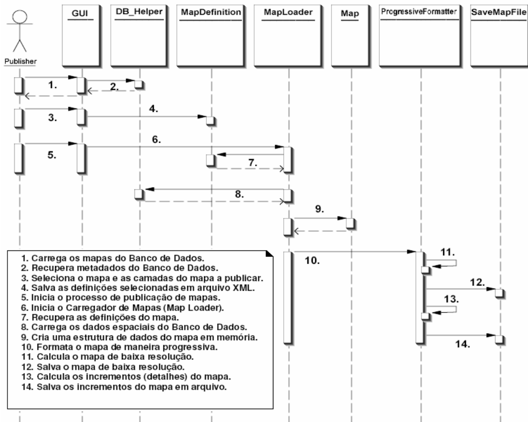
Figura 5.14. Cenário de geração de mapas progressivos.
