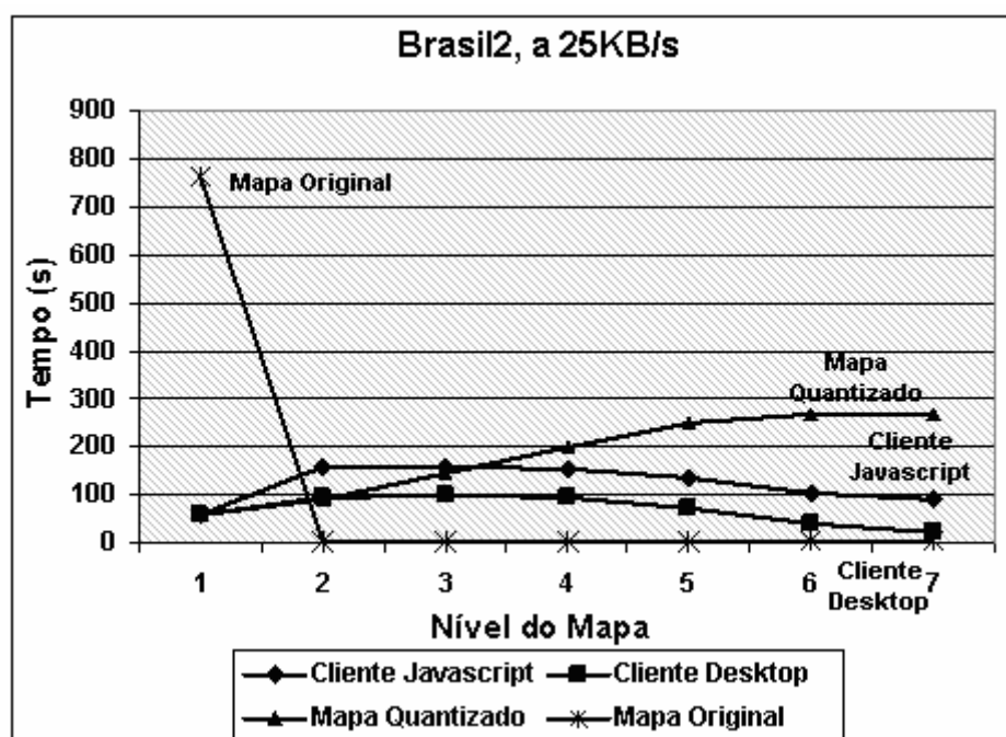
Figura 6.6. Tempo de transmissão para o mapa Brasil2, a 25KB/s.
