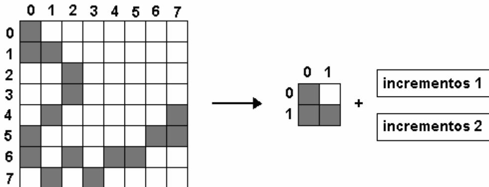
Figura 5.3. Decomposição em mapa base e incrementos.
