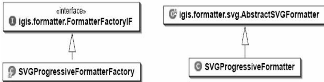
Figura 5.11. Extensão de Classes Progressivas a partir das classes iGIS.
