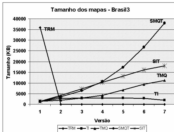
Figura 6.4. Gráfico comparativo para o mapa Brasil3
