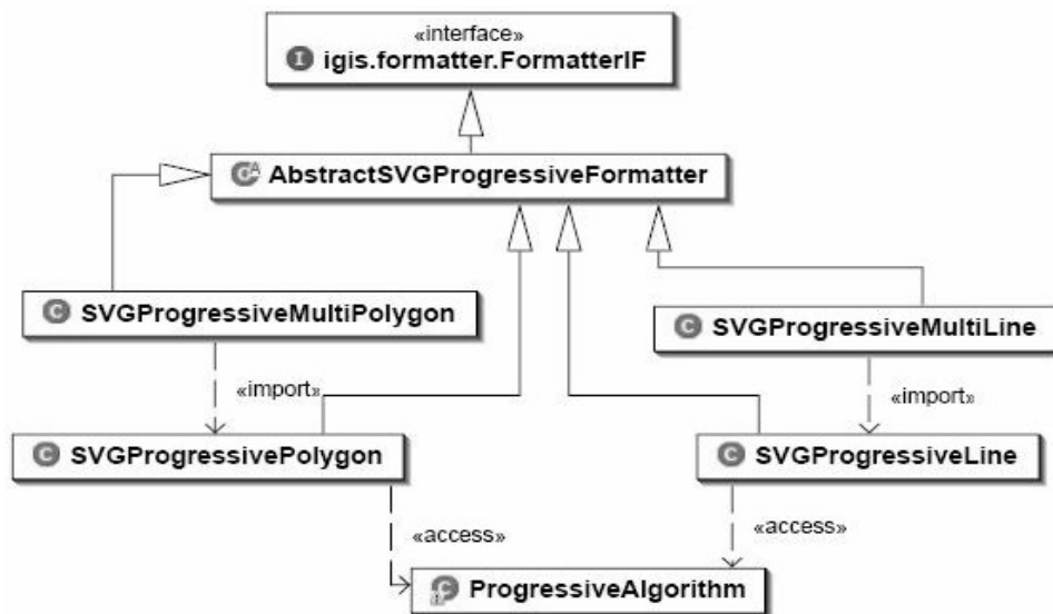
Figura 5.13. Classes que processam as geometrias progressivamente.
