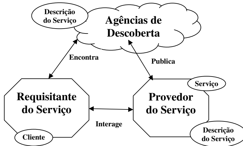
Figura 4.2. Arquitetura geral da tecnologia de Web Services.
