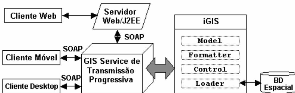
Figura 5.18. Arquitetura de GIS Services Proposta.
