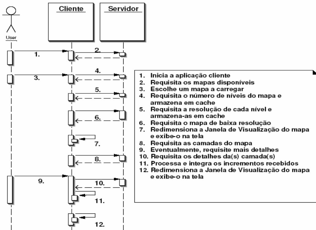
Figura 5.15. Cenário de utilização dos mapas progressivos
