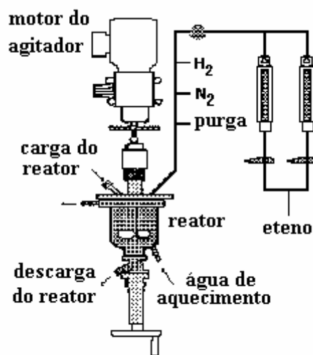
Figura 8 - Reator metálico (utilizado nas reações de polimerização na IPQ)
