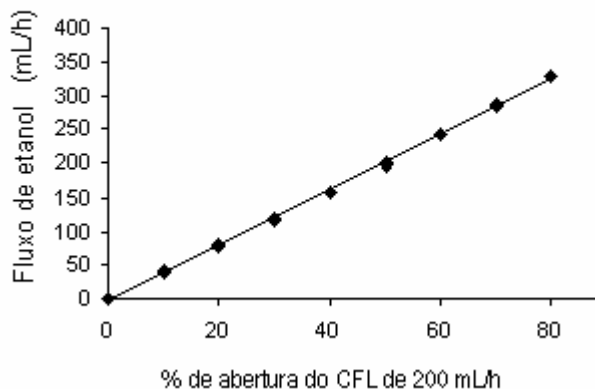
Figura 9. Curva de calibração para o fluxo de etanol com CFL 200 mL/h
