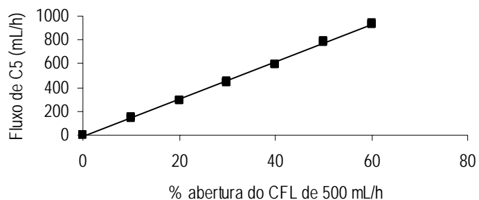
Figura 8: Curva de calibração para o fluxo de C 5 com CFL 500 mL/h
