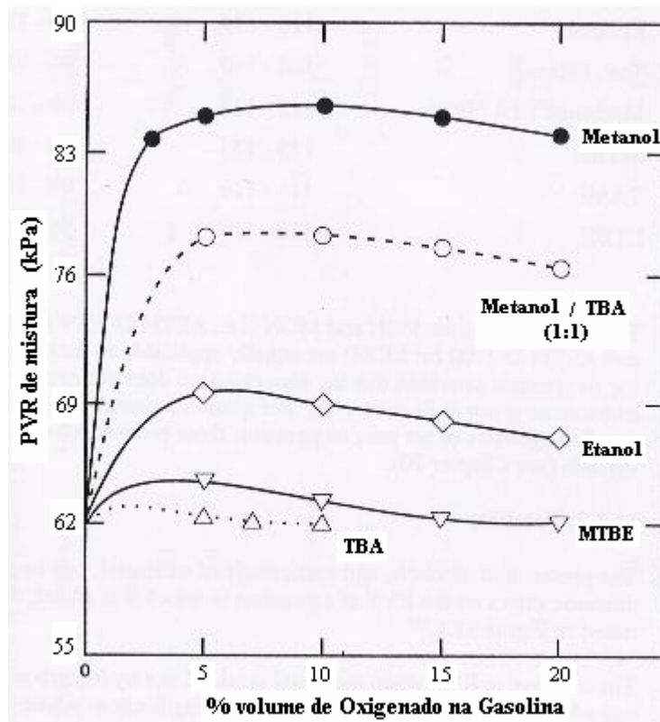
Figura 6: Efeito da concentração de oxigenados no PVR das misturas de gasolina. (Gasolina base: Indoleno HO III) 8
