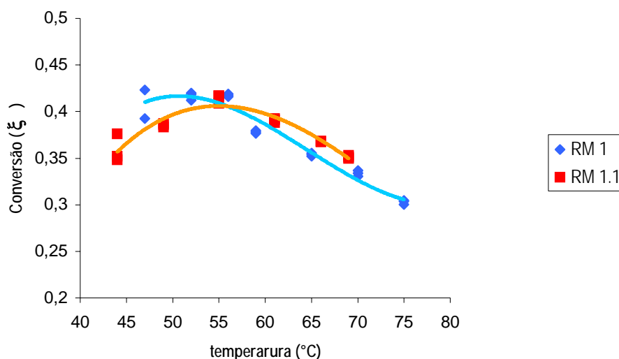
Figura 10. Gráfico da conversão de 2M1B e 2M2B em TAEE em função da temperatura no 1.º Passe pelo reator.
