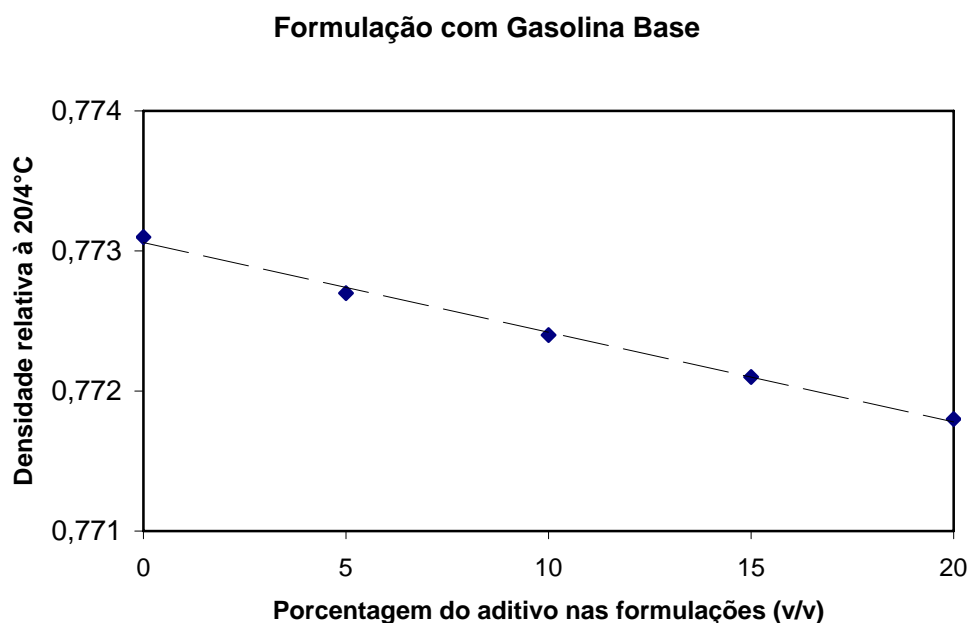
Figura 19: Densidade relativa à 20/4°C da formulação da gasolina base com TAEE nas proporções (v/v) de 5, 10, 15 e 20%.
