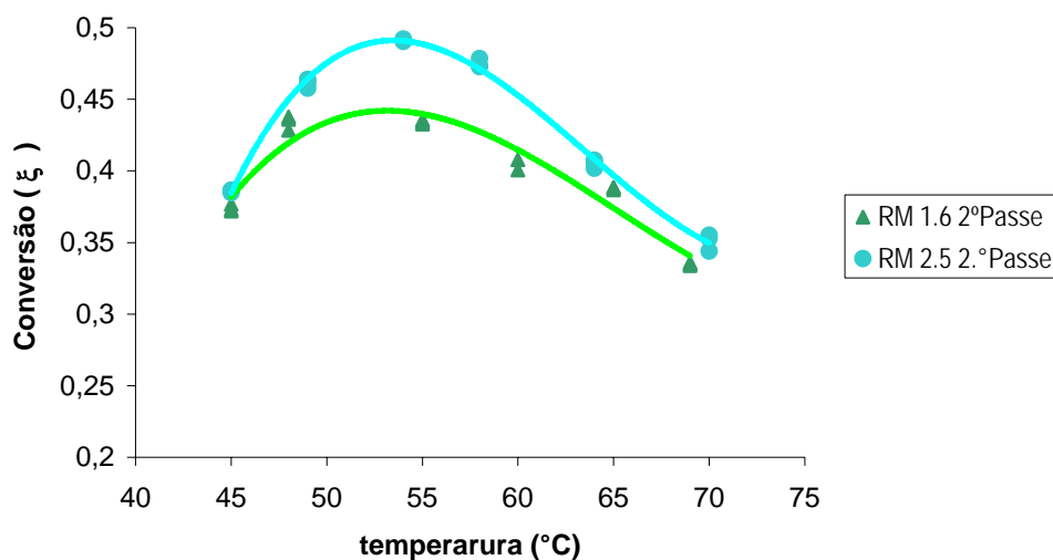
Figura 11. Gráfico da conversão de 2M1B e 2M2B em TAEE em função da temperatura no 2.º Passe pelo reator.
