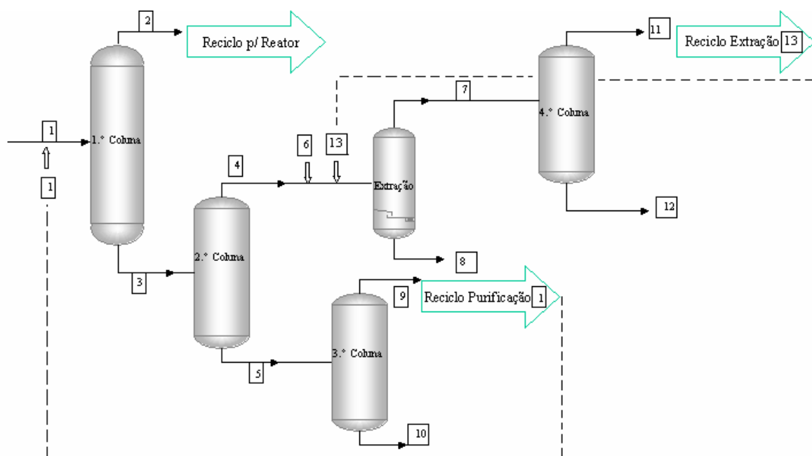
Figura 17. Diagrama de fluxo da unidade de purificação do TAEE.
