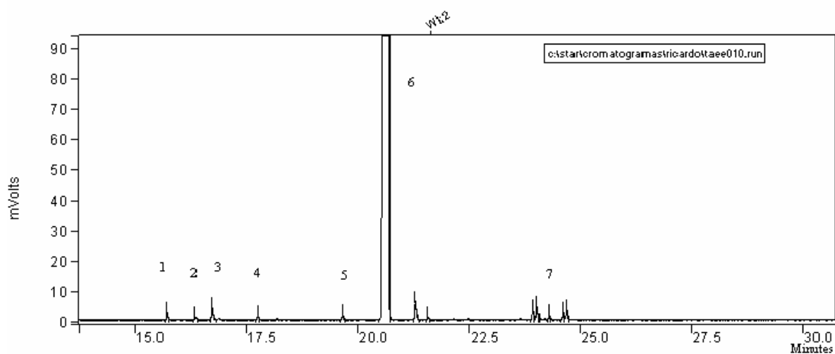
Figura 18: Cromatograma em detalhe do TAE com 99,5% molar (GC-FID).
