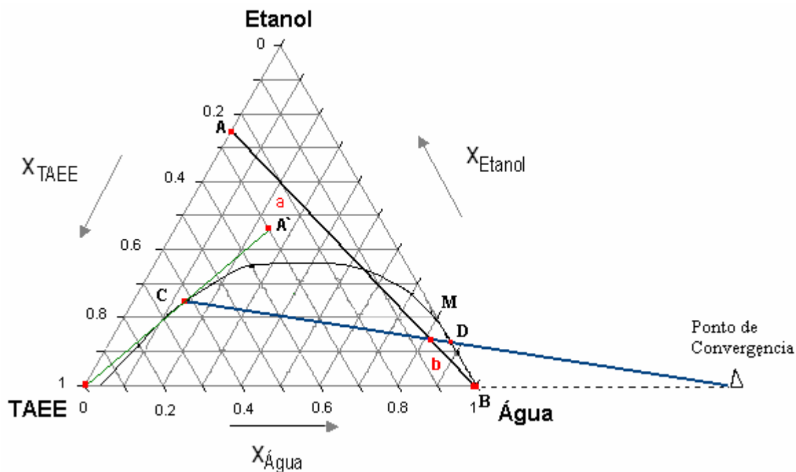
Figura 16: Diagrama ternário para análise da extração líquido-líquido do sistema (água/etanol/TAEE).
