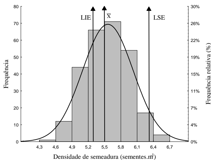
Figura 9 - Histograma de distribuição e curva normal dos dados do indicador de densidade de semeadura
