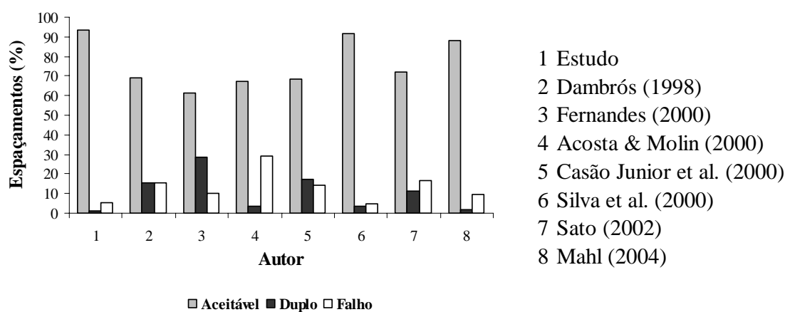
Figura 15 - Comparação entre os valores obtidos na bibliografia e no estudo para o indicador de distancia entre sementes no sulco
