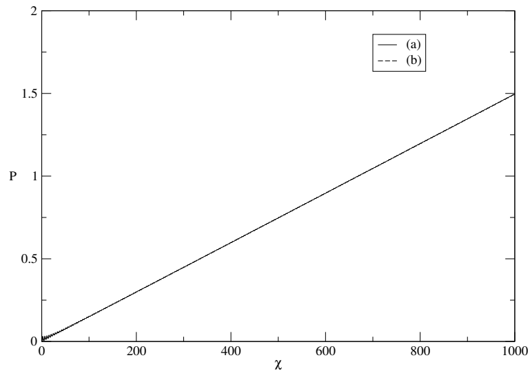
Figura 3.2: Momento normalizado do plasma P versus distância normalizada (fase) \chi para \Omega_c = 0.1 e S_\nu = 0.03 (a) Elétrons, (b) Pósitrons.
