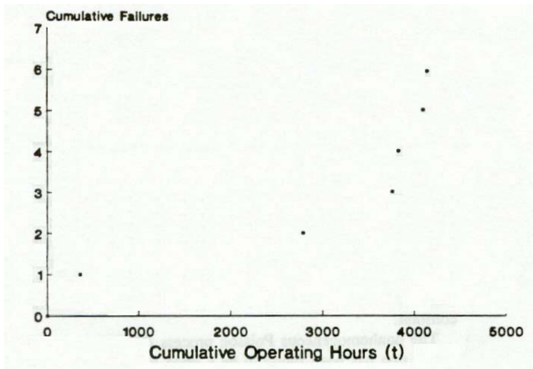
FIGURA 19 - Análise gráfica da tendência do sistema
