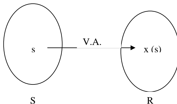
FIGURA 1 - Representação da variável aleatória
