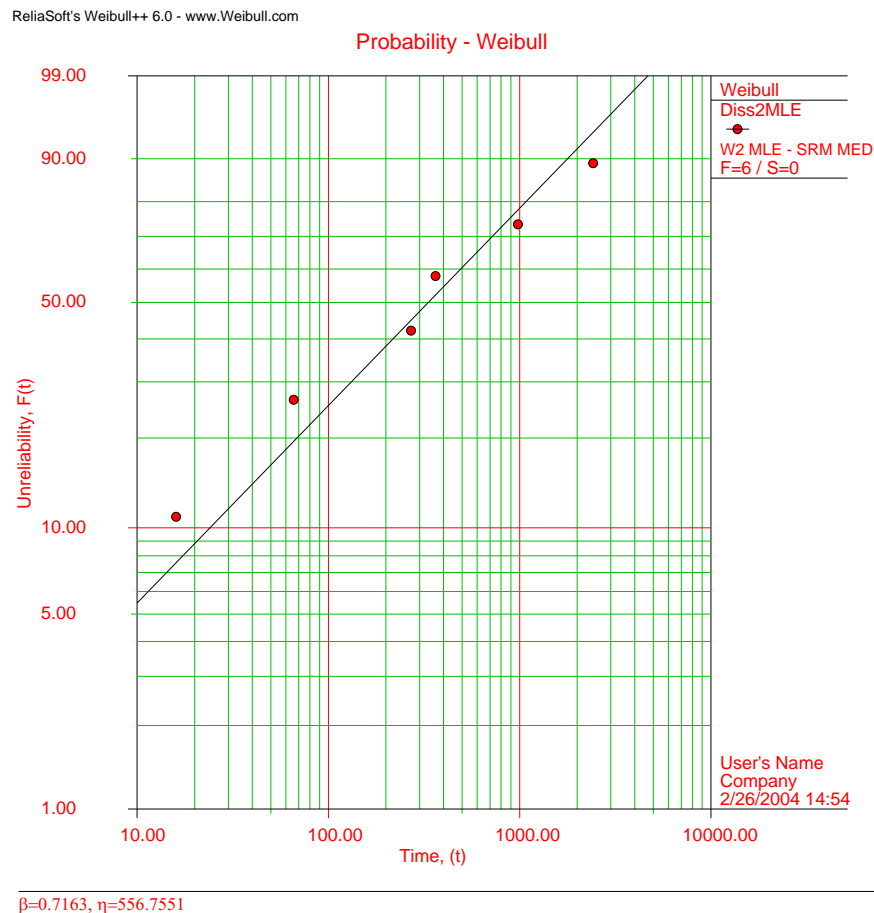
FIGURA 18 - Gráfico Weibull dos dados da tabela tempo de operação do sistema
