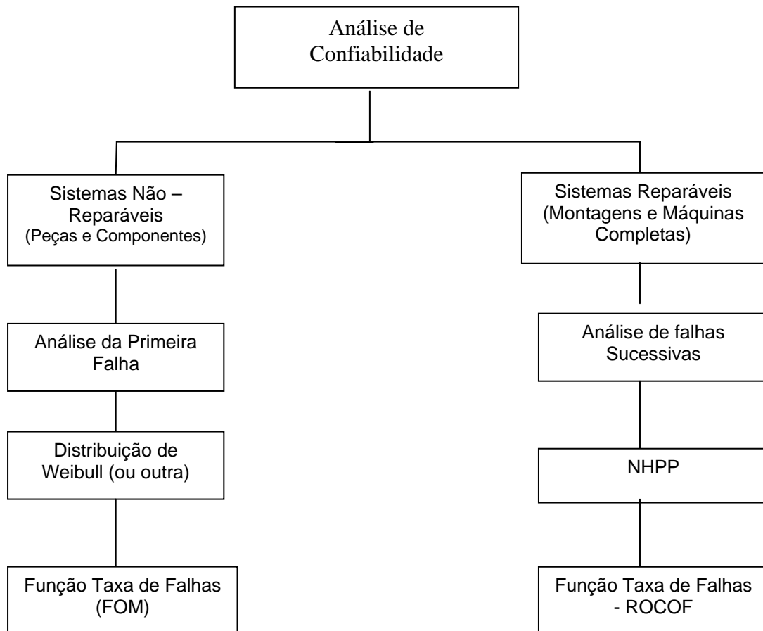
FIGURA 25 - Modelo para análise de falhas de máquinas
