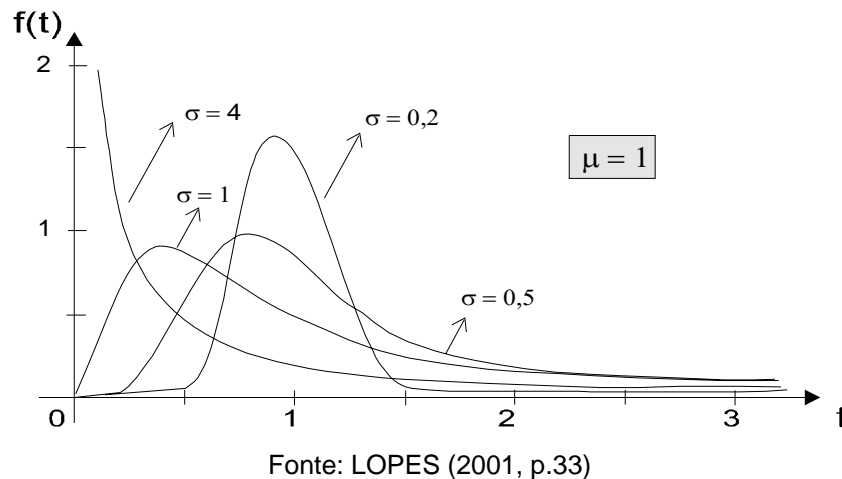
FIGURA 5 - Função densidade de probabilidade log-normal para \mu = 1 e alguns valores de \sigma
