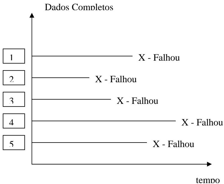
FIGURA 8 - Representação de dados completos
