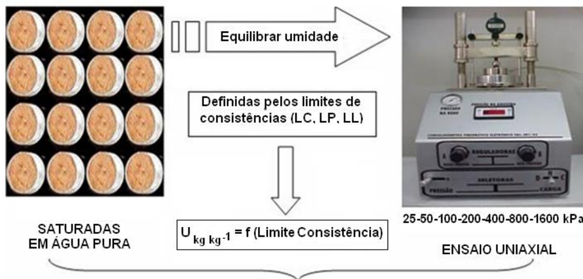
Figura 4. Procedimentos laboratoriais para realização dos ensaios de compressibilidade e obtenção da pressão de preconsolidação ( \sigma_p ). LC (Limite de Contração), LL (Limite de Liquidez) e LP (Limite de Plasticidade). Consolidômetro desenvolvido por Silva et al. (2005a).
