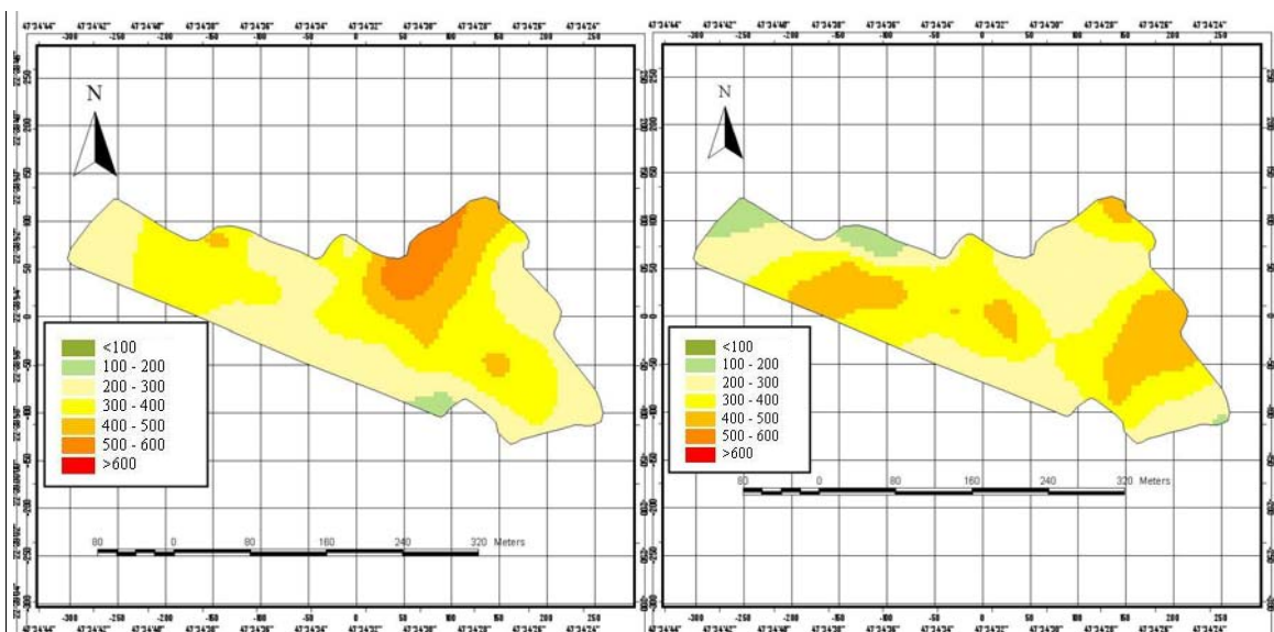
Figura 21. Variabilidade espacial da pressão de preconsolidação ( \sigma_p - kPa) do Talhão III LV , na região de consistência de friabilidade em função das duas profundidades avaliadas.
