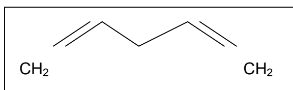
FIGURA 1 - Isopreno – Unidade estrutural dos compostos isoprenóides.
