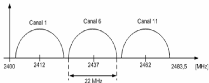
Figura 2.3 - Atribuição de canais no padrão IEEE 802.11b.
