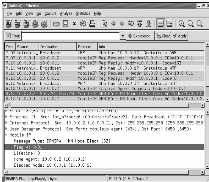
Figura A.7 - Visualização do MNnodelect Advertisement no Ethereal.
