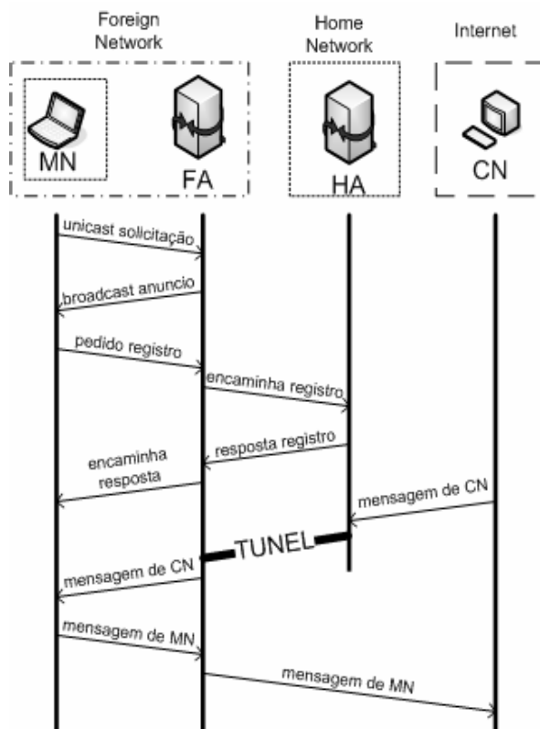
Figura 2.5 - Processo de sinalização entre MN, FA e HA.
