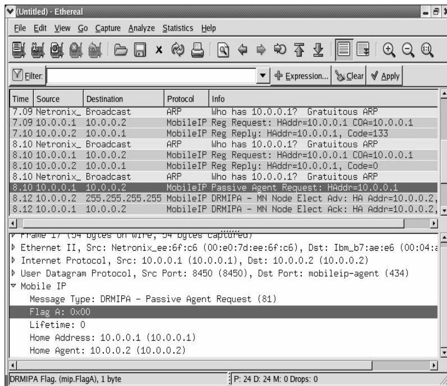
Figura A.5 - Visualização do Passive Agent Request no Ethereal.
