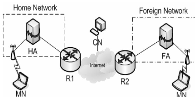
Figura 2.1 - Topologia básica do MIP.
