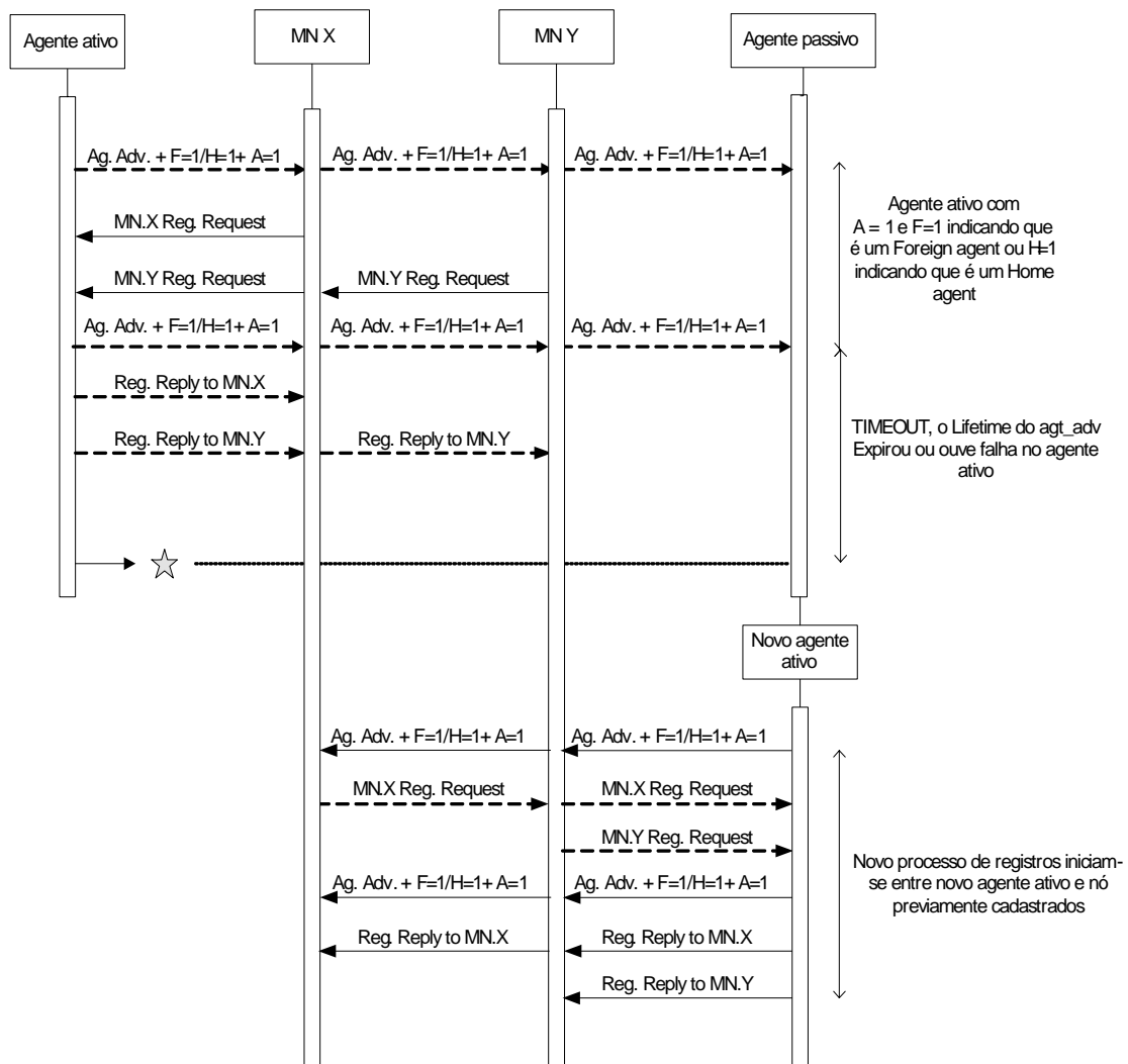
Figura 4.9 - Sinalização da mudança do agente ativo para agente passivo.
