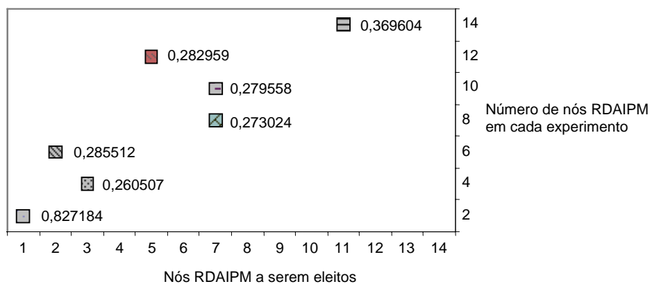
Figura 6.1 - Tempo para eleição do agente passivo RDAIPM (em segundos).
