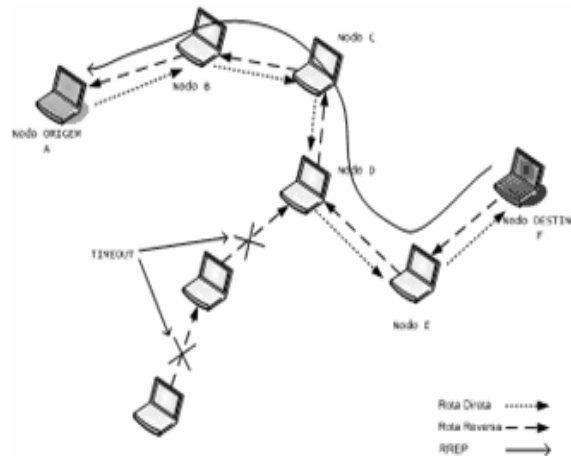
Figura 3.2 - Propagação dos RREPs e estabelecimento da rota direta entre os nós de origem e destino, A e F respectivamente.
