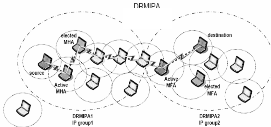
Figura 4.20 - Novo MIPv4 em MANET.
