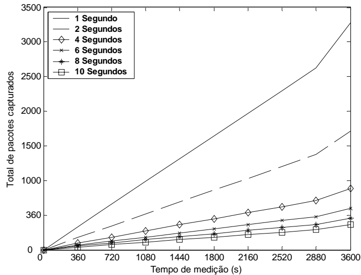
Figura 6.17 - Total Pacotes ADV&SOL gerados em 1 salto.
