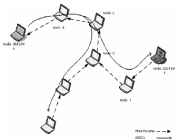
Figura 3.1 - Propagação dos RREQs e estabelecimento da rota reversa entre os nós de origem e destino A e F respectivamente.
