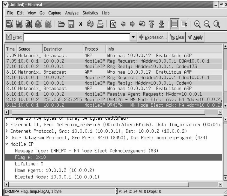
Figura A.9 - Visualização do MNnodelect Acknowledgement no Ethereal
