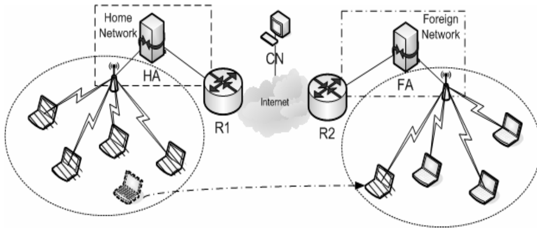
Figura 4.3 - Estrutura MIPv4 atual.
