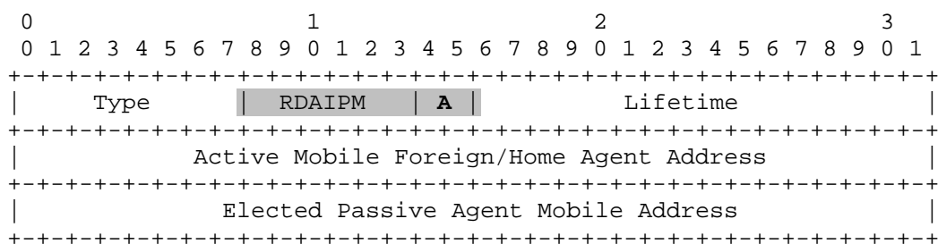
Figura A.6 - Estrutura do MNnodelect Advertisement.
