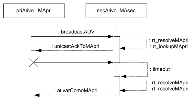
Figura 4.8 - Diagrama de seqüência para detecção da queda do agente ativo e atualização da lista de visitantes.
