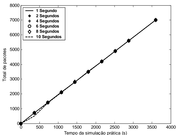
Figura 6.16 - Total Pacotes AODV gerados em 1 salto.
