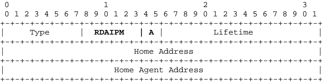
Figura 4.15 - Mensagem Passive Agent Request (Type=81, A=00).
