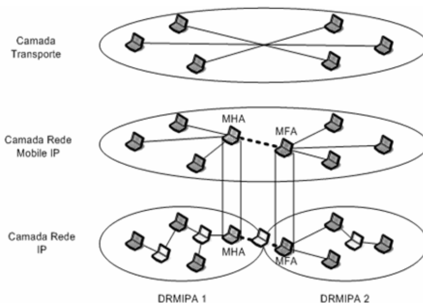
Figura 4.19 - Visão conceitual do RDAIPM.
