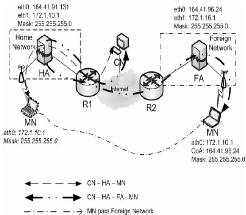
Figura 2.4 - Roteamento de datagramas para e de um nó móvel numa rede estrangeira.
