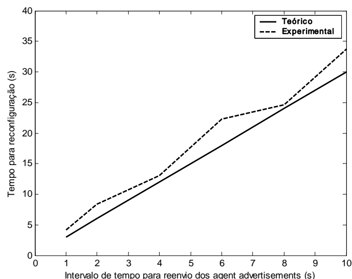
Figura 6.10 - Comparativo entre os tempos de reconfiguração esperados teóricos e práticos em 1 salto.
