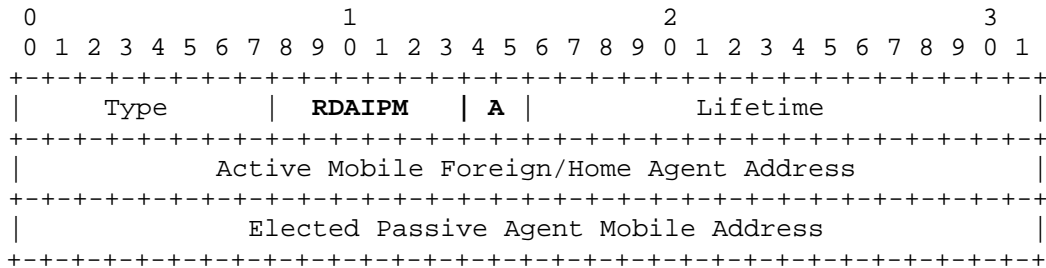
Figura 4.16 - Mensagem MNnodelect Advertisement do MA ativo para nós da rede (Type=82, A=01).
