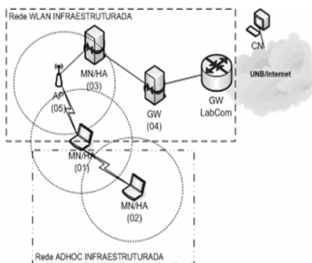
Figura 6.14 - Cenário MANET e WLAN.
