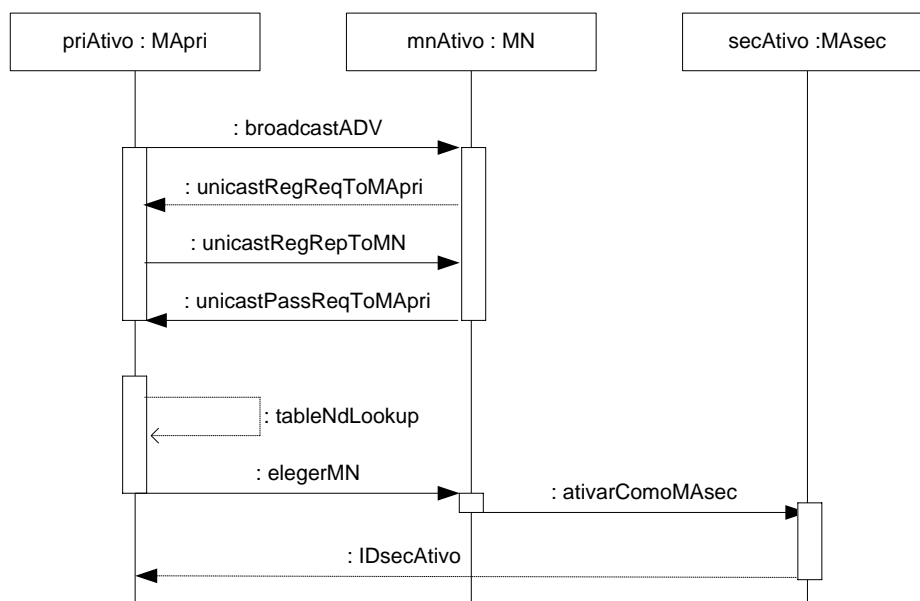
Figura 4.7 - Diagrama de seqüência para eleger um agente passivo.
