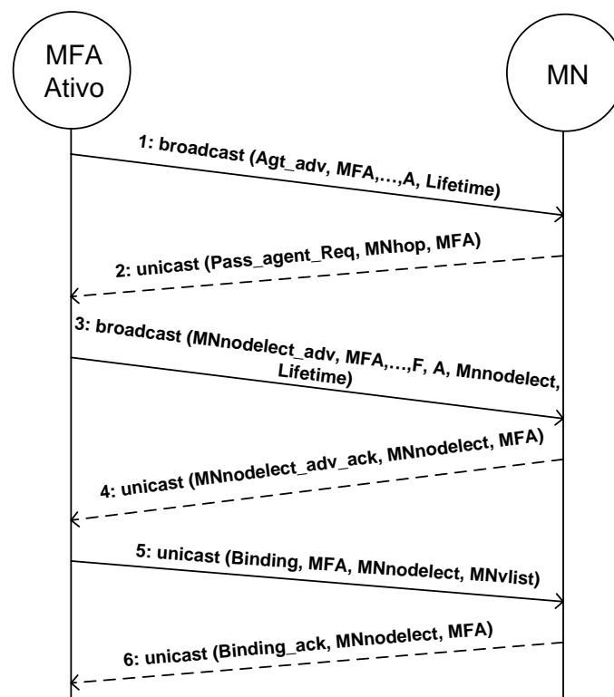
Figura 4.10 - Sinalização da eleição do agente passivo.
