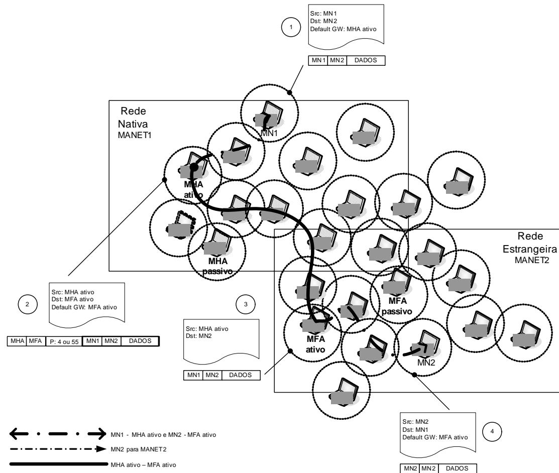
Figura 5.1 - Exemplificação do Tunelamento na rede RDAIPM.
