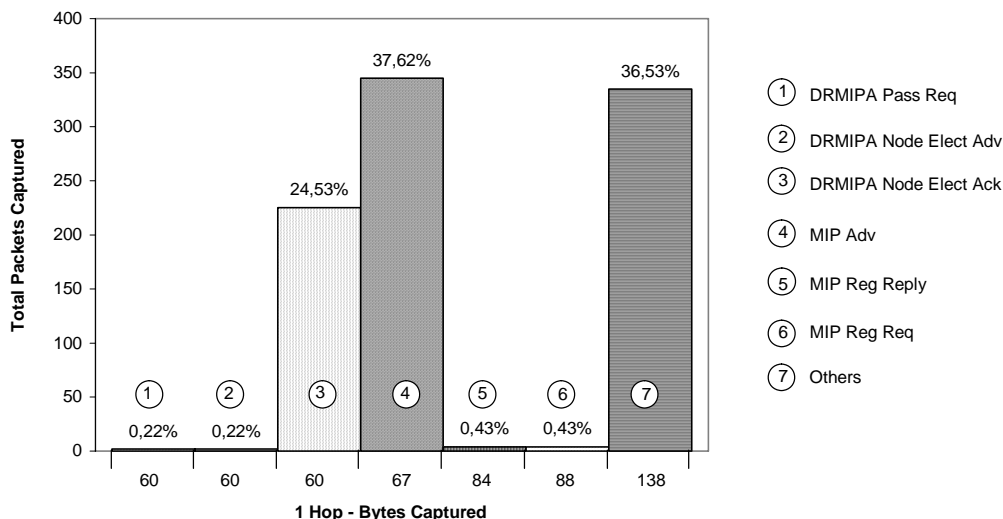
Figura 6.11 - Total Pacotes capturados na WLAN em 1 salto.
