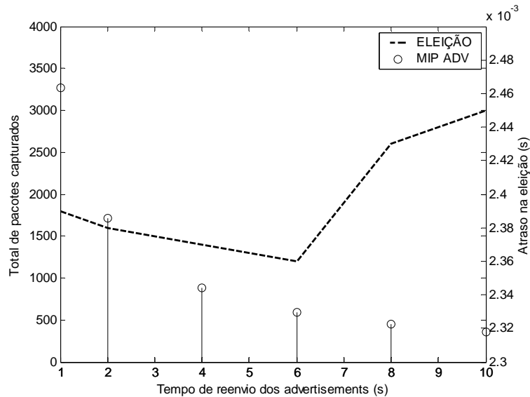
Figura 6.15 - Tempo de eleição de agente passivo versus intervalo de tempo para anúncio de agente ativo.
