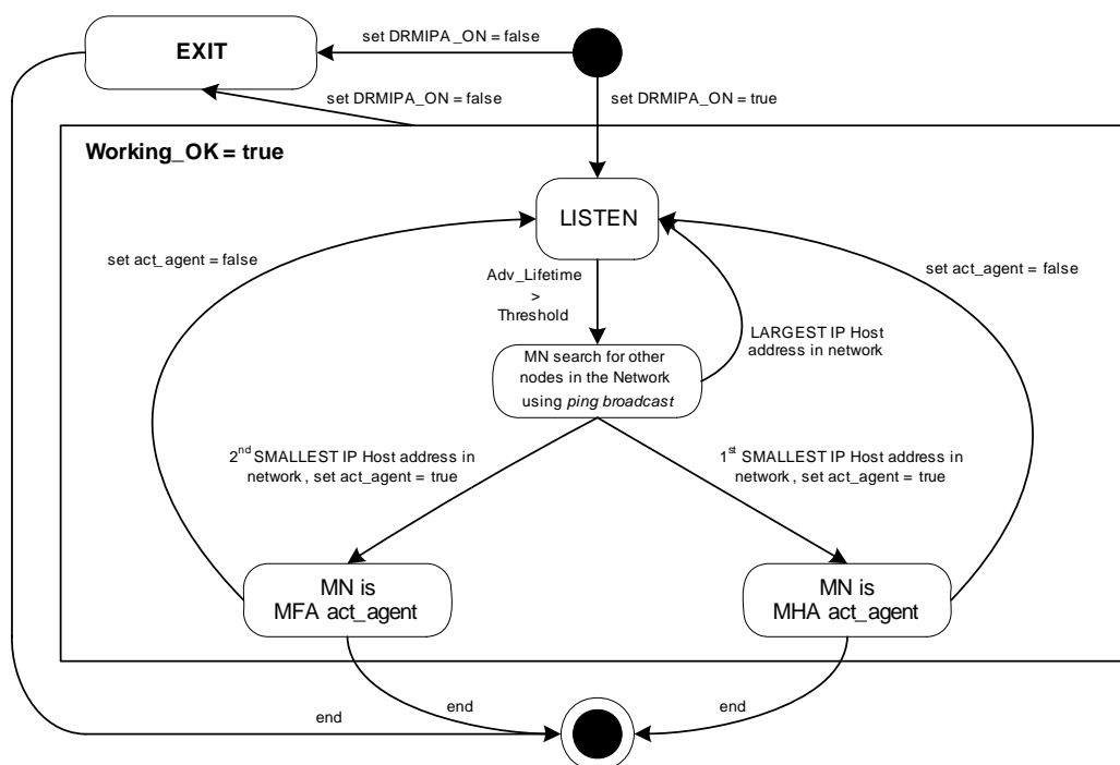
Figura 4.17 - Diagrama de estados básico para autoconfiguração de um MN.
