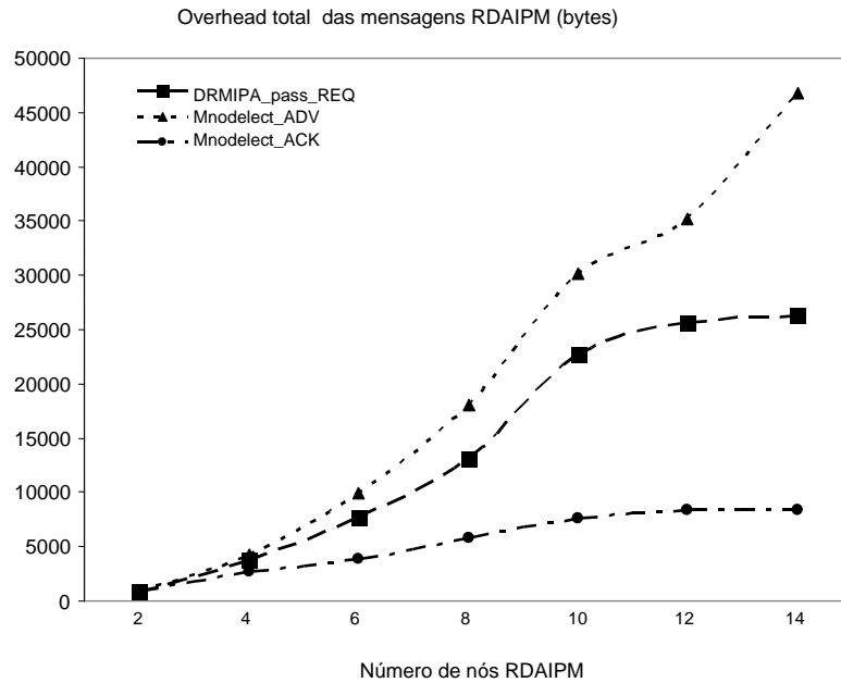
Figura 6.1 - Overhead das mensagens principais do RDAIPM em bytes.
