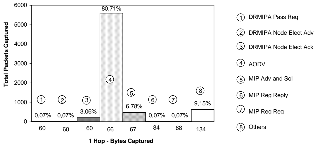
Figura 6.122 - Total Pacotes capturados na MANET em 1 salto.
