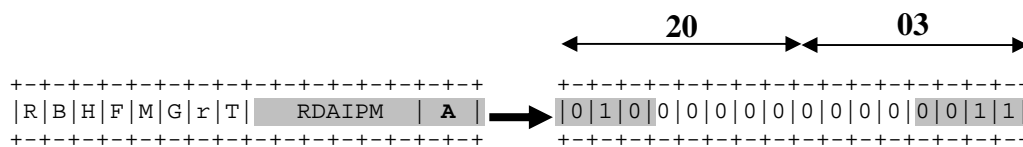
Figura A.2 - Valores dos octetos FLAGS e RESERVED.
