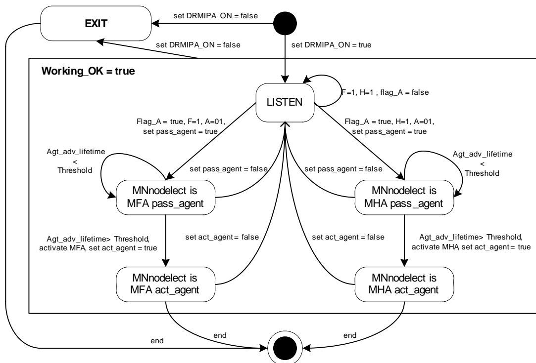
Figura 4.11 - Diagrama de estados básico para um Mnodelect.
