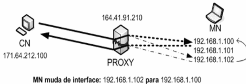
Figura 2.6 - Mobilidade na Camada de Transporte.
