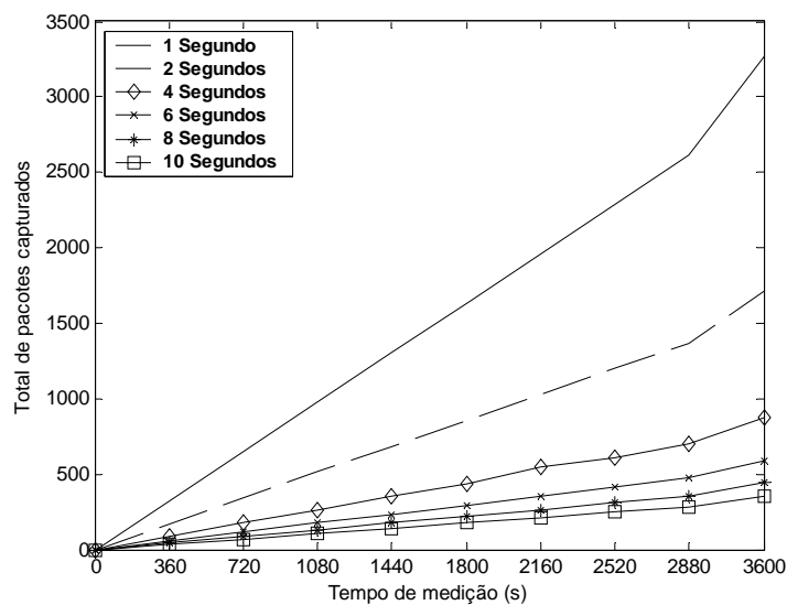
Figura 6.18 - Total Pacotes MN_NodeElect_Ack gerados em 1 salto.
