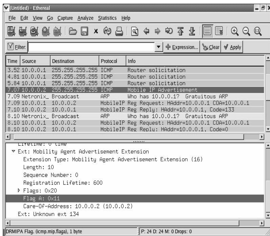
Figura A.3 - Visualização do RDAIPM Agent Advertisement no Ethereal
