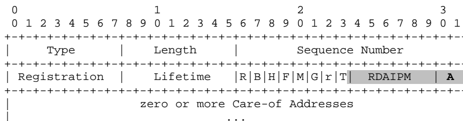
Figura A.1 - Estrutura do RDAIPM Agent Advertisement
