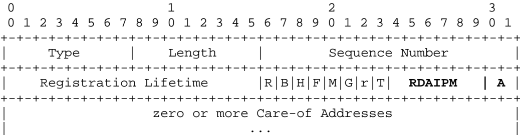
Figura 4.14 - Mensagem MIP de agent advertisement modificada (Type=16, A=11).
