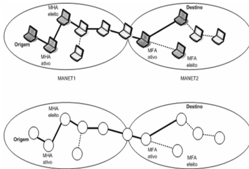
Figura 4.5 - Eleição de um agente móvel na rede MANET.
