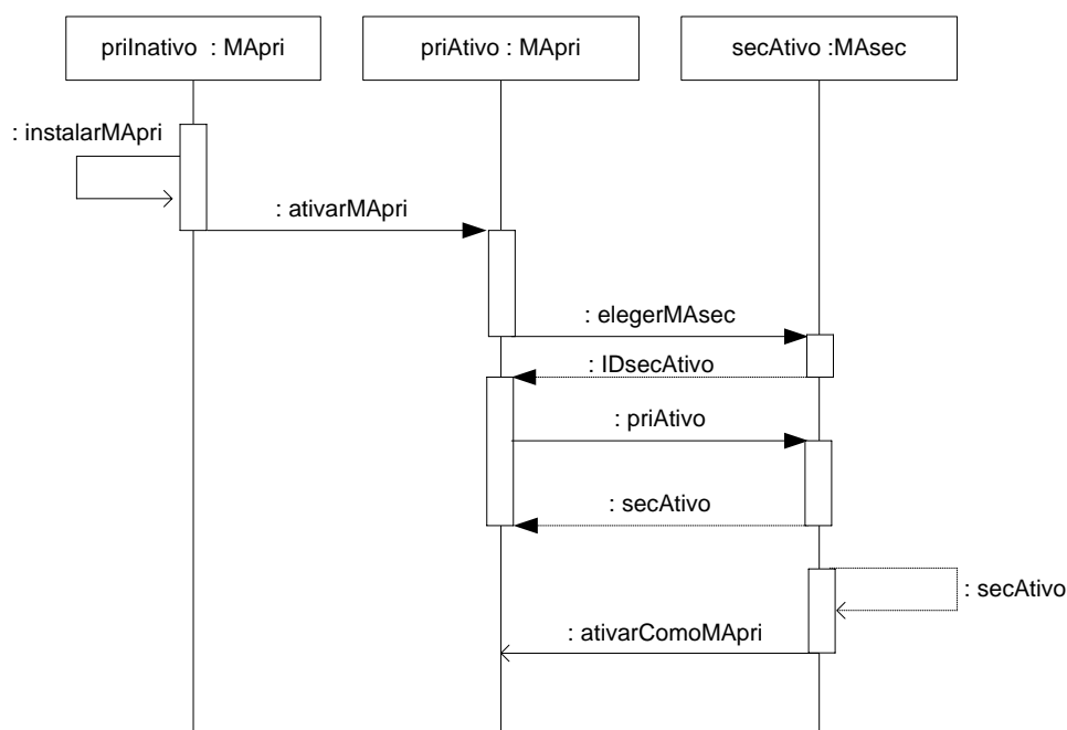
Figura 4.6 - Diagrama de seqüência para configurar os agentes móveis ativos ( MApri ) e passivo ( MAsec ).
