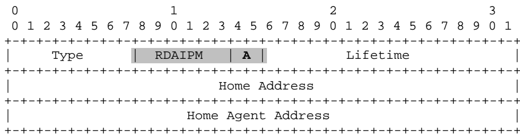
Figura A.4 - Estrutura do Passive Agent Request.
