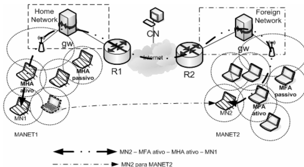
Figura 4.4 - Novo MIPv4 em MANET com acesso a gateways.
