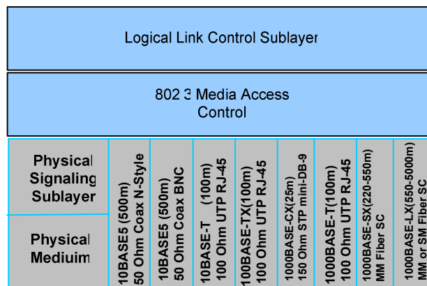
Figura 4.16 - Subcamada MAC – OSI
