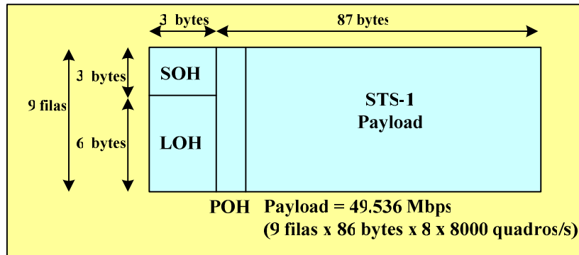
Figura 4.26 - Malha básica STS-1 (SONET)
