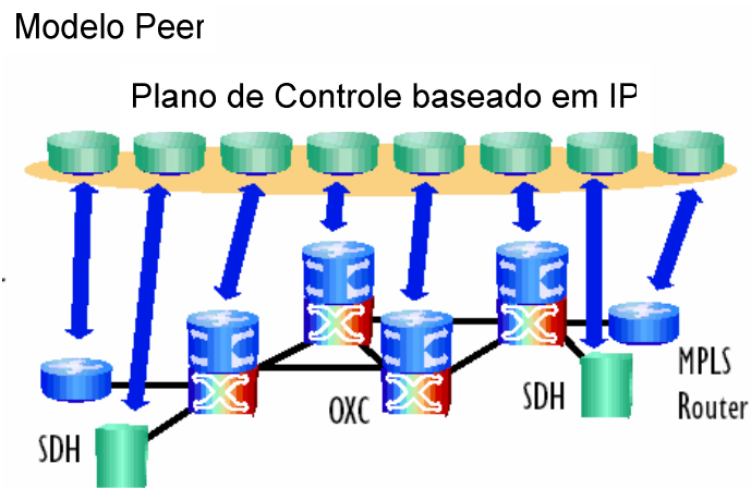
Figura 4.10 - Arquitetura do modelo Peer com controle distribuído
