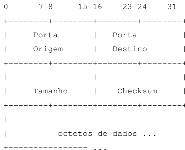
Figura 7.1 – Formato de um datagrama UDP
