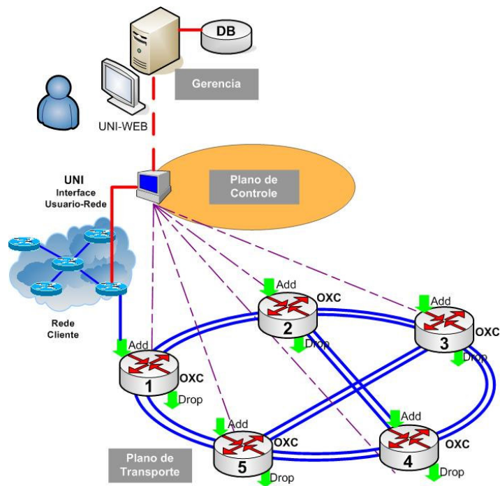
Figura 6.2 - Visão completa da arquitetura proposta.
