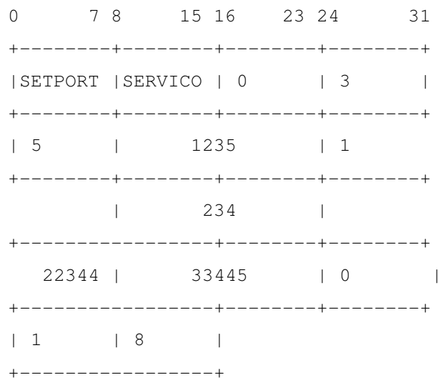
Figura 7.2 – Configuração de um pacote Set da requisição 234
