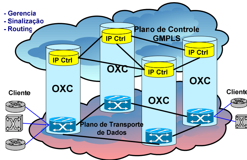
Figura 4.13 - Plano de controle e plano de transporte de dados
