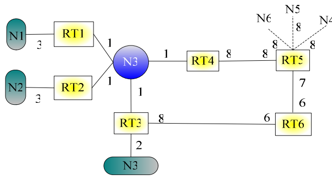
Figura 6.10 - Topologia física de uma rede
