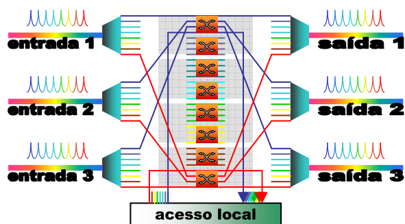
Figura 5.4 - Elementos de um nó e suas conexões
