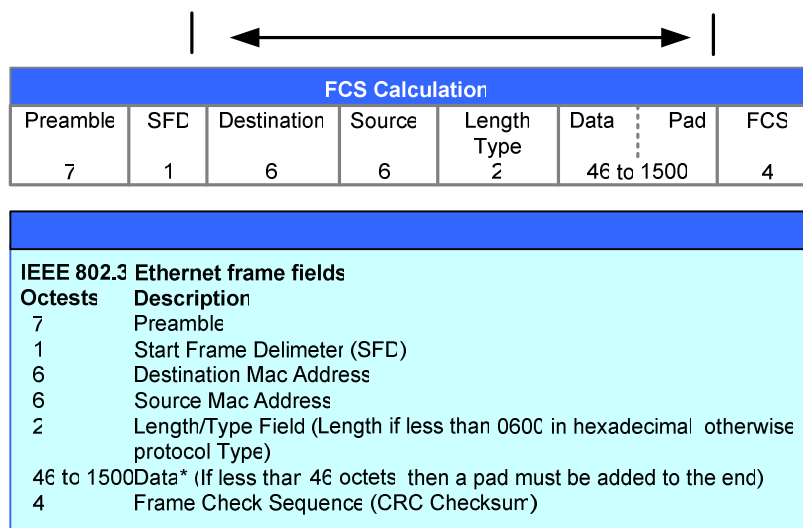
Figura 4.18 - Frame 802.3 Ethernet
