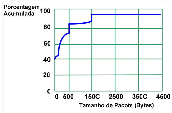
Figura 4.23 - Tamanho de pacotes num enlace doméstico [THOMPSON, 1997]
