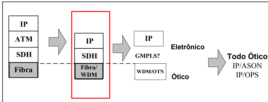
Figura 4.24 - Eliminação da camada ATM e propostas para IP diretamente sobre fibra
