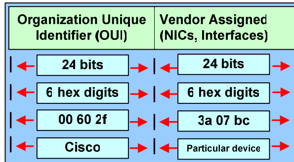
Figura 4.17 - Formato do endereço MAC
