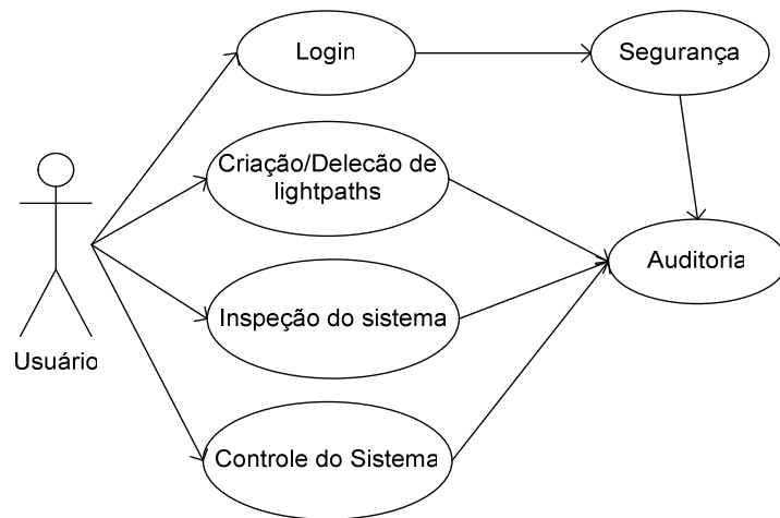
Figura 6.4 - Caso de Uso da Gerência
