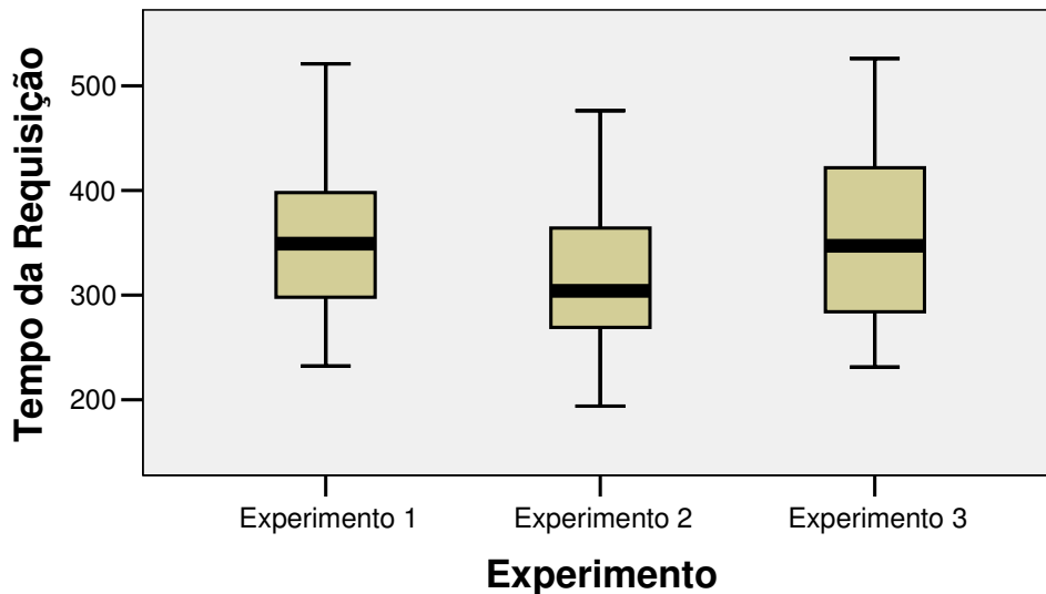
Figura 7.7 – Gráfico de caixas
