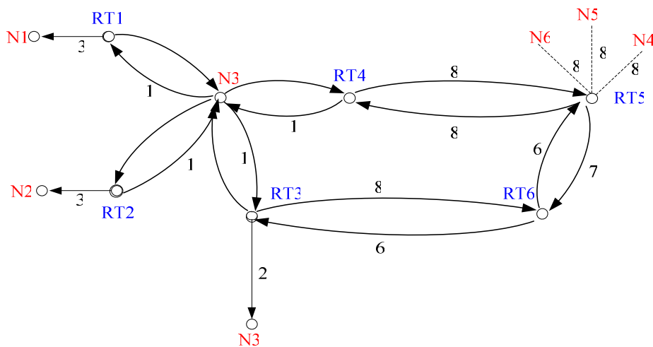
Figura 6.11 - Grafo resultante
