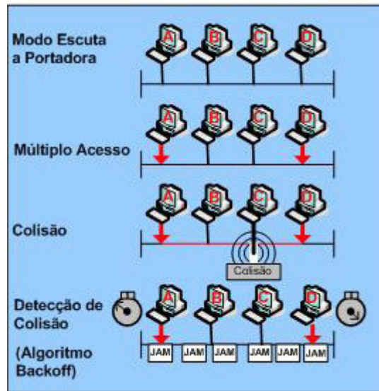
Figura 4.20 - Método de acesso CSMA/CD
