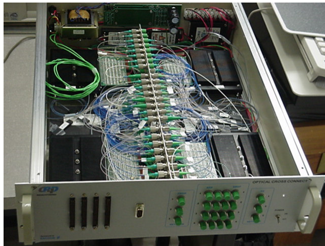
Figura 5.5 - Optical cross-connect (OXC) da rede OMEGA.
