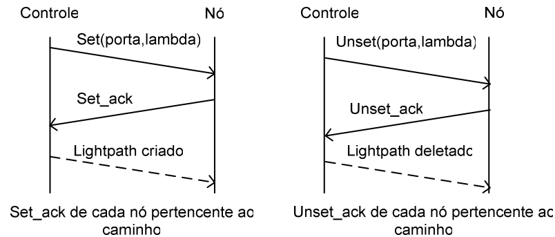
Figura 6.12 - Sequência de eventos
