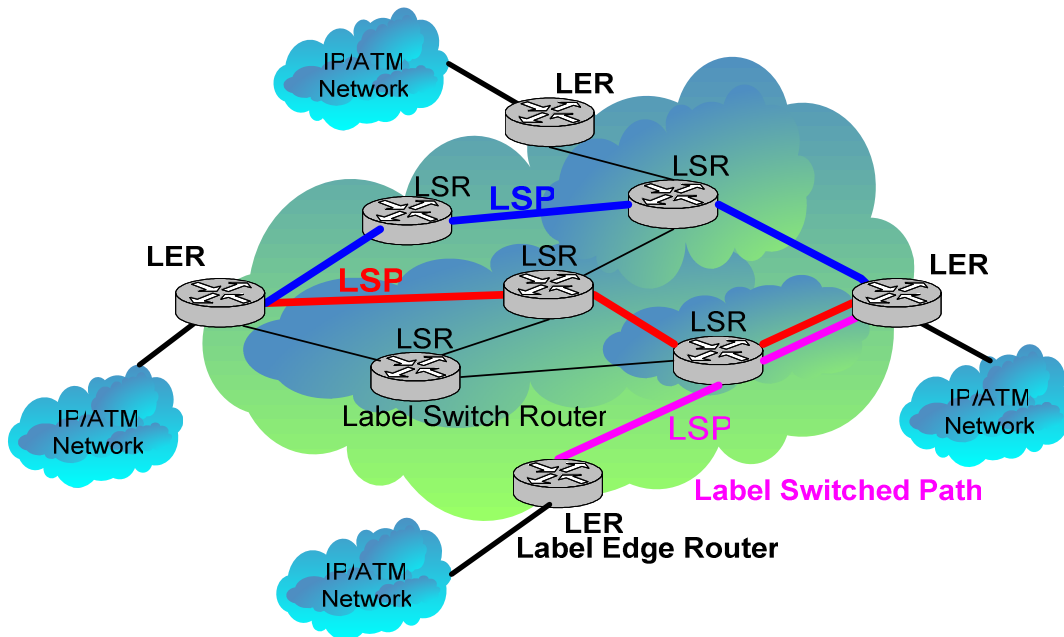
Figura 4.3 - Componentes LER, LSR e LSP de um domínio MPLS.
