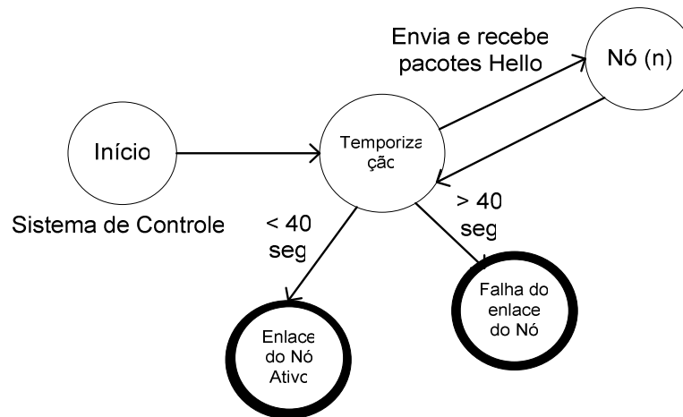
Figura 6.13 - Diagrama de estado do protocolo Hello
