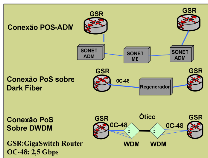
Figura 4.28 - Configurações de Rede IP sobre SDH
