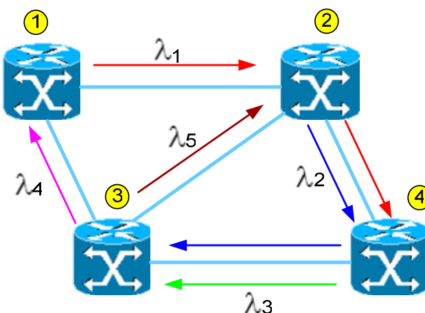
Figura 2.6 - Topologia de uma rede WDM com 5 comprimentos de onda
