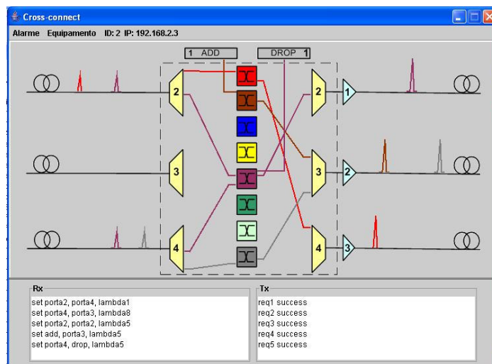
Figura 6.16 – OXC simulado
