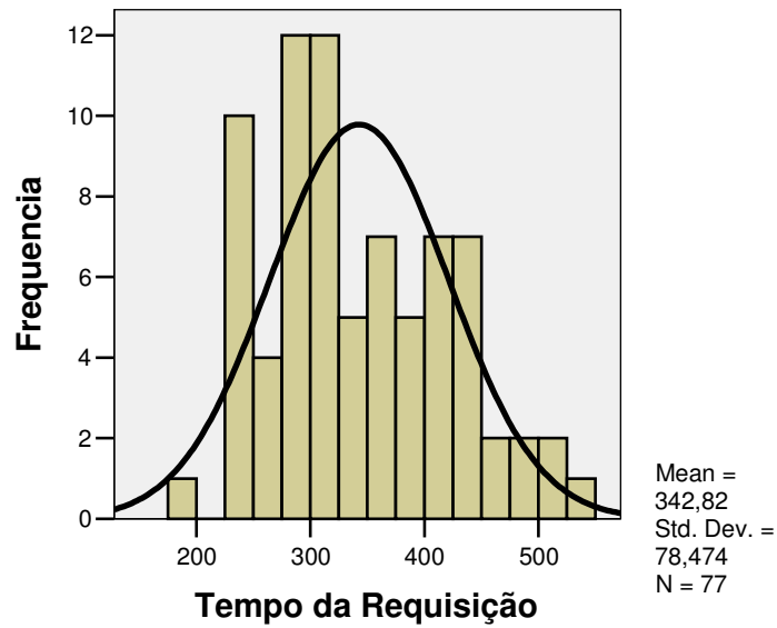
Figura 7.5 – Histograma do tempo da requisição para todos os experimentos
