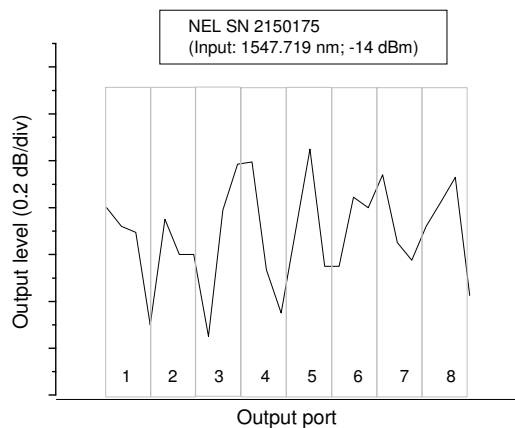
Figura 5.7 - Flutuação do nível de potência da porta de saída do switch
