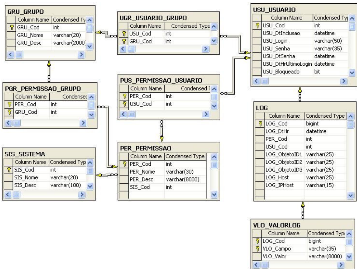
Figura 6.9 - Modelo Entidade Relacionamento
