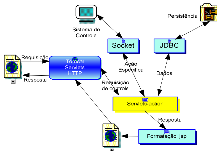
Figura 6.5 - Diagrama da arquitetura da camada de gerência
