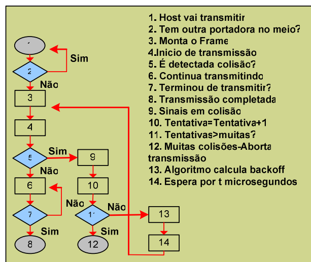
Figura 4.21 - Fluxograma da operação do CSMA/CD
