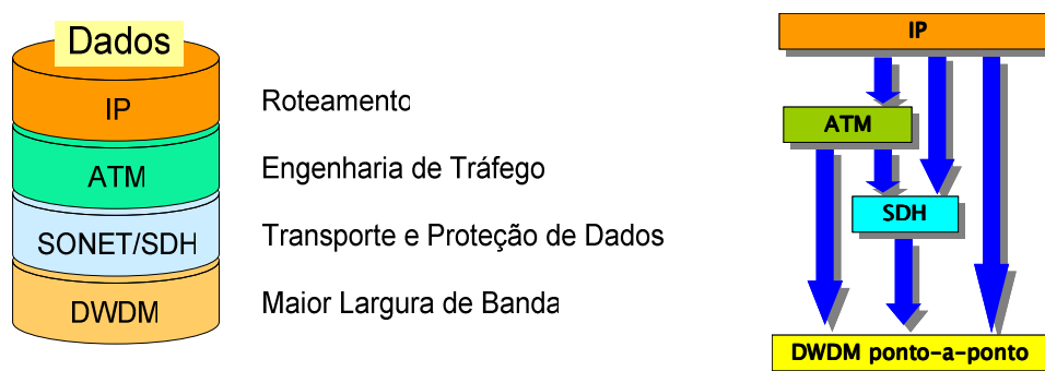
Figura 4.1 - Camadas da Rede de Transporte
