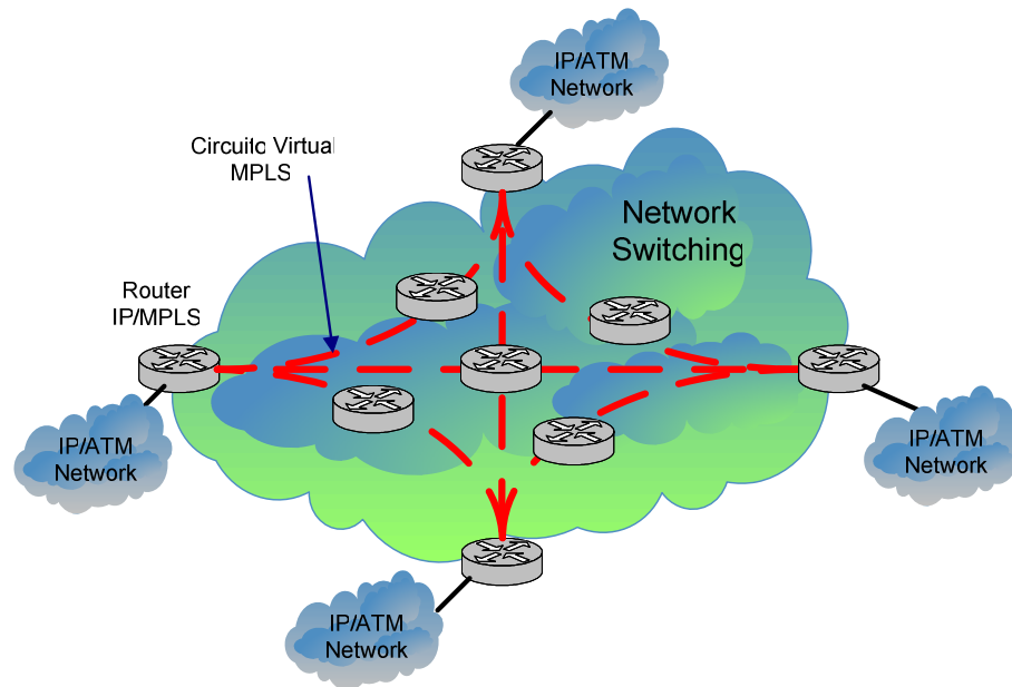
Figura 4.2 - Exemplo de uma rede de comutação IP/MPLS.
