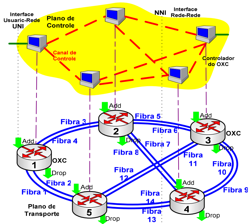
Figura 5.1 - Plano de Transporte e Plano de Controle da Rede OMEGA
