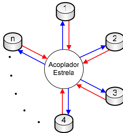
Figura 2.1 - Rede óptica com topologia estrela.
