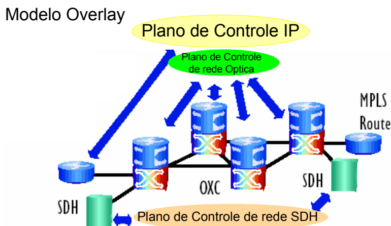
Figura 4.12 - Modelo Overlay com plano de controle centralizado
