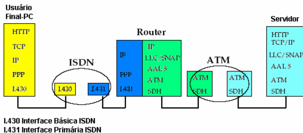
Figura 4.22 - Exemplo de uma rede IP/ATM usando encapsulamento LLC
