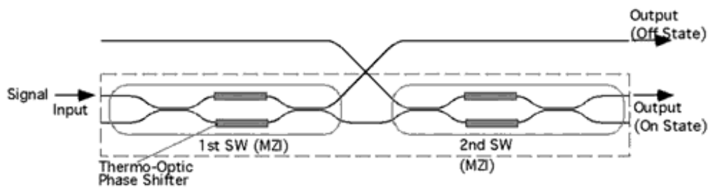
Figura 3.1 - Configuração da unidade de chaveamento da chave termo-óptica 8 x 8
