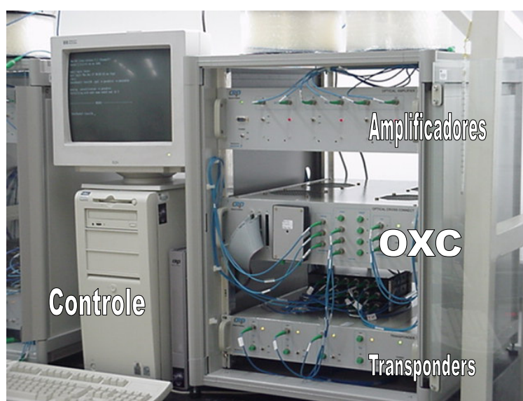
Figura 5.3 - Estrutura física de um nó da rede OMEGA
