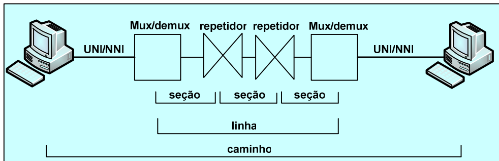
Figura 4.25 - Níveis de overhead em SDH/SONET
