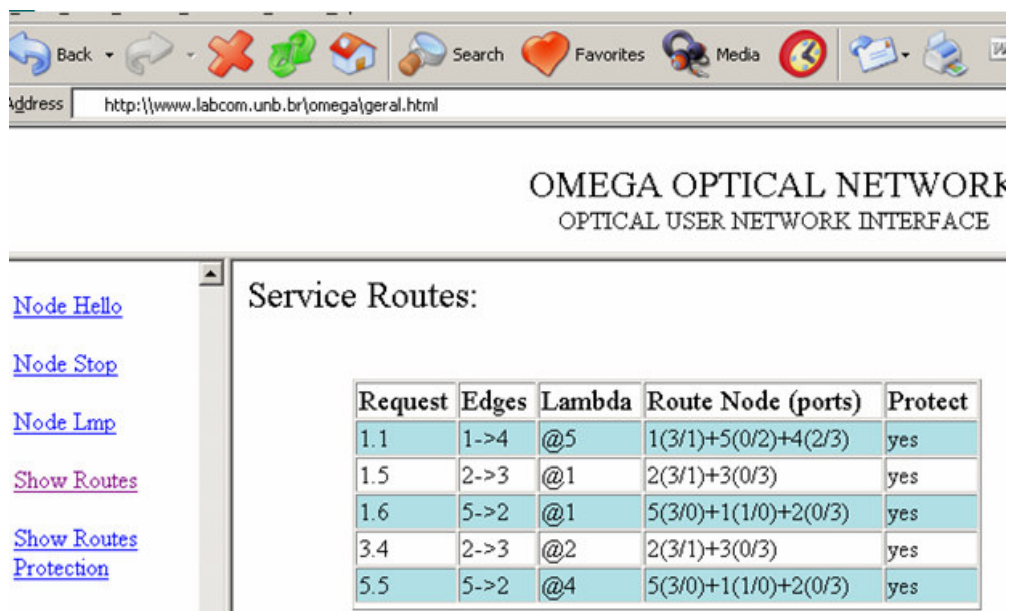
Figura 6.8 - Administração de um nó óptico
