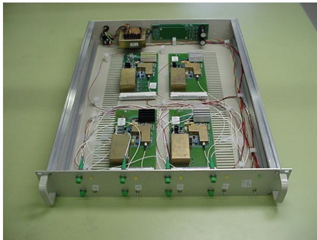
Figura 5.6 - Módulo Transponder (Quatro pares TX/RX).
