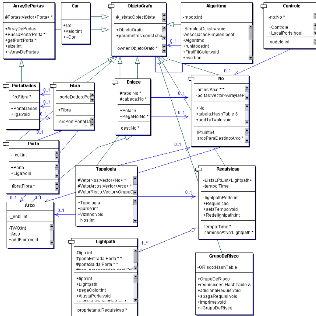
Figura 6.15 – Diagrama de Classes
