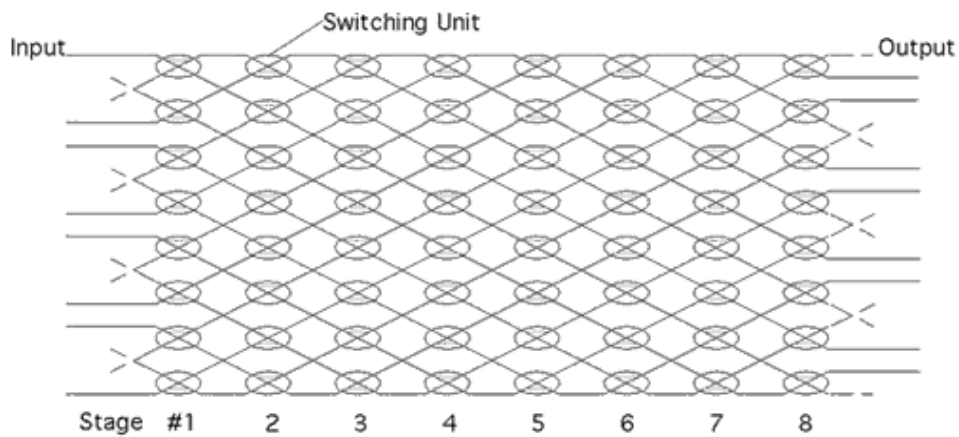
Figura 3.2 - Arranjo local de uma chave termo-óptica 8 x 8
