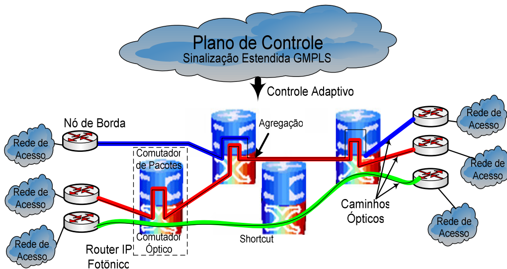
Figura A. 1 - Rede Fotônica IP
