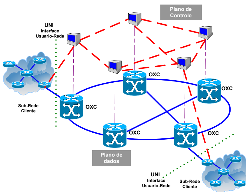
Figura 2.9 - Arquitetura de rede óptica
