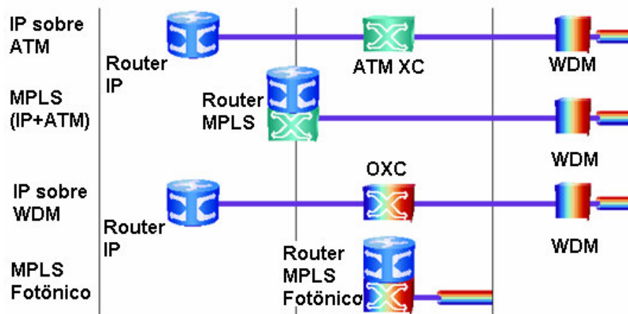
Figura 4.5 - Evolução das Configurações da Rede de Transporte baseadas em IP
