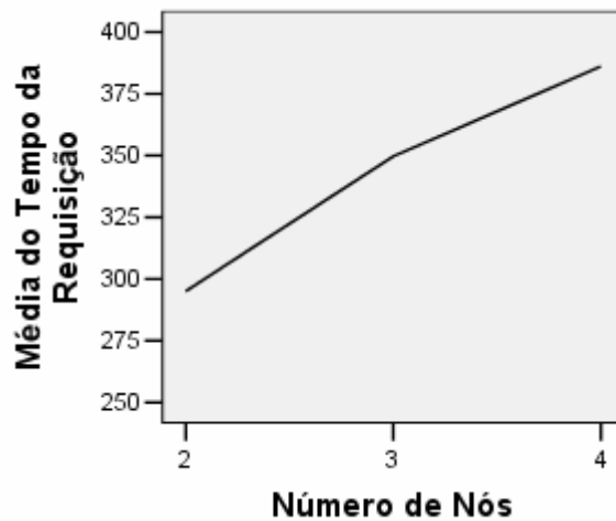
Figura 7.6 – Correlação entre número de nós e tempo da requisição em ms
