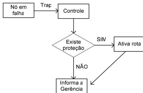
Figura 6.14 – Lógica de proteção
