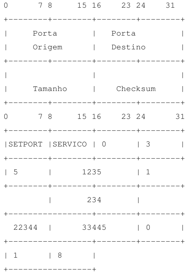
Figura 7.3 – Configuração de um pacote UDP para um Set
