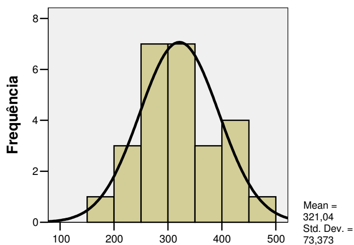
Figura 7.4 – Histograma do tempo da requisição para o experimento dois
