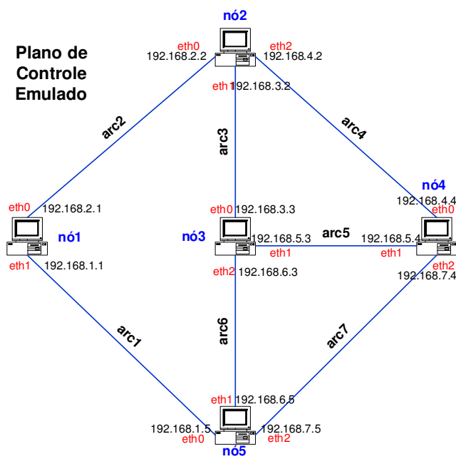
Figura 5.8 - Plano de controle emulado no Laboratório da UnB
