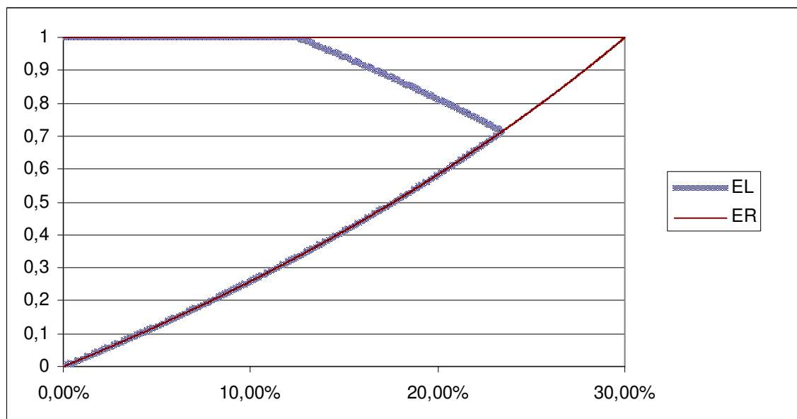
Figura 2.14 – Comportamento do erro de linearização de Chiu e Park (1994).
