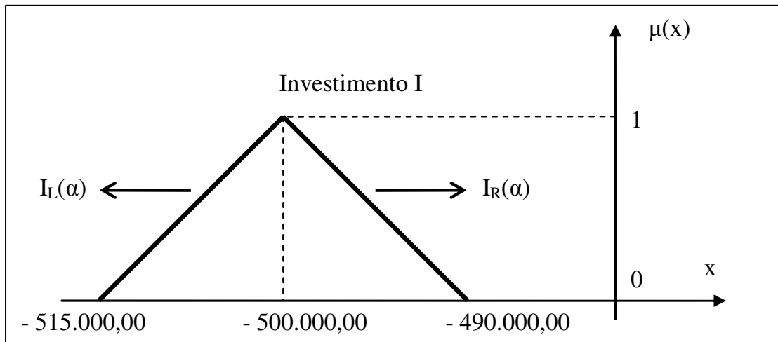
Figura 2.5 – Representação fuzzy do investimento I
