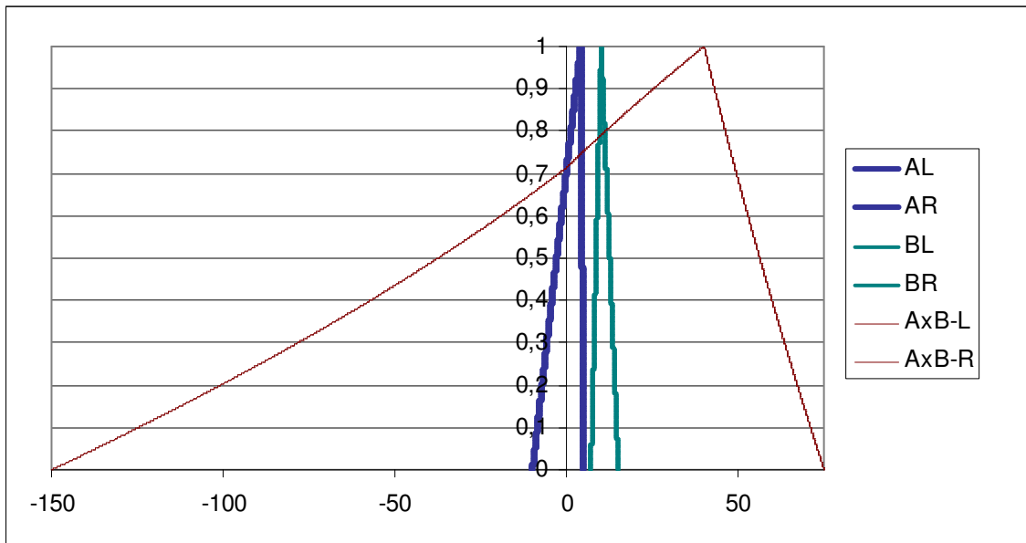
Figura 2.8 – Multiplicação de dois números fuzzy A e B.
