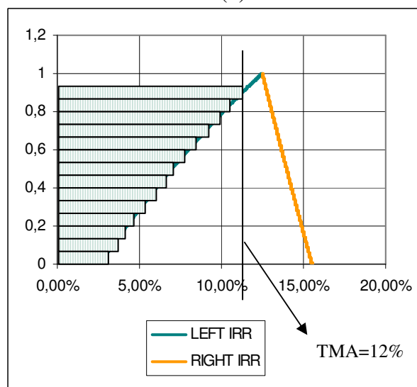
Figura 3.8 – TIRF exata para o fluxo de caixa da tabela 3.1, integrada pelo método de Riemann.
