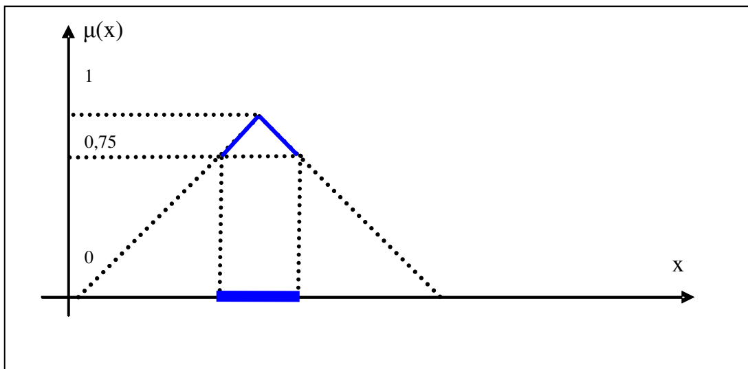
Figura 2.4 – Exemplo de um \alpha -cut, com A(\alpha) = A(0,75)
