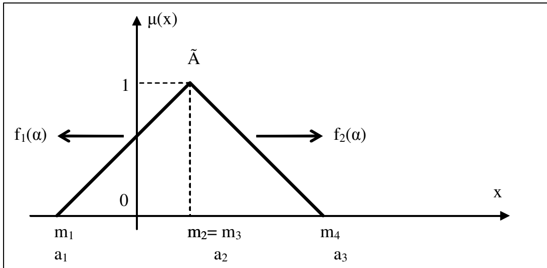
Figura 2.2 – Número fuzzy triangular (TFN)
