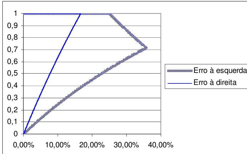
Figura 2.12 – Comportamento do erro de linearização com relação ao valor exato.
