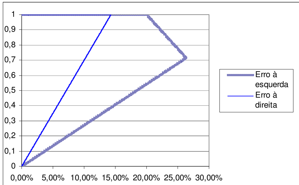
Figura 2.11 – Comportamento do erro de linearização de Chiu e Park (1994).
