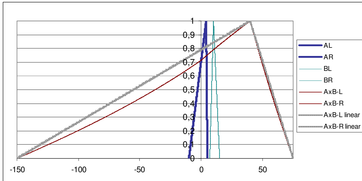
Figura 2.10 – Multiplicação com resultado linearizado.
