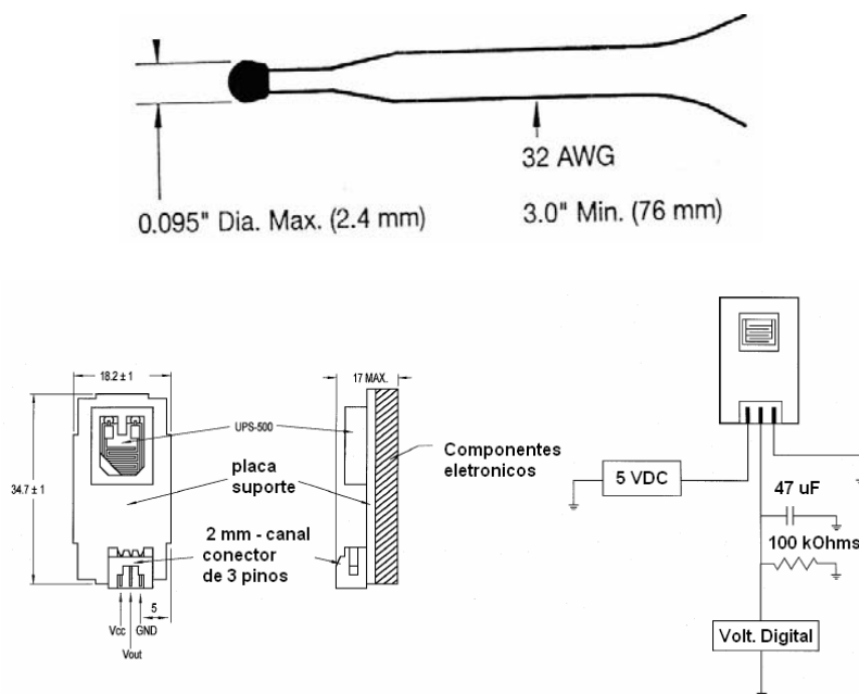
FIGURA 15 TERMISTORES E SENSORES DE UMIDADE RELATIVA
