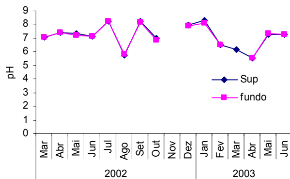
Fig 17. Variação de pH ( superfície e fundo) durante o período de março/2002 a junho/2003, nos pontos R3,R5 e R1 ( canal da represa) e em L14, L22, L9 e L19 que correspondem respectivamente à desembocadura de Ribeirão de Água Fria, Córrego São João, Ribeirão do Lajeado e Ribeirão do São João.
