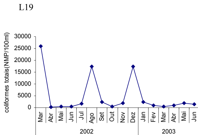
Fig 24. Variação da concentração de coliformes totais ( superfície e fundo) durante o período e março/2002 a junho/2003, nos pontos R3,R5 e R1 ( canal da represa) e em L14, L22, L9 e L19 que correspondem respectivamente à desembocadura de Ribeirão de Água Fria, Córrego São João, Ribeirão do Lajeado e Ribeirão do São João
