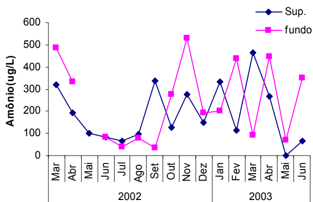
Fig 21. Variação da concentração de amônio ( superfície e fundo) durante o período de março/2002 a junho/2003, nos pontos R3,R5 e R1 ( canal da represa) e em L14, L22, L9 e L19 que correspondem respectivamente à desembocadura de Ribeirão de Água Fria, Córrego São João, Ribeirão do Lajeado e Ribeirão do São João
