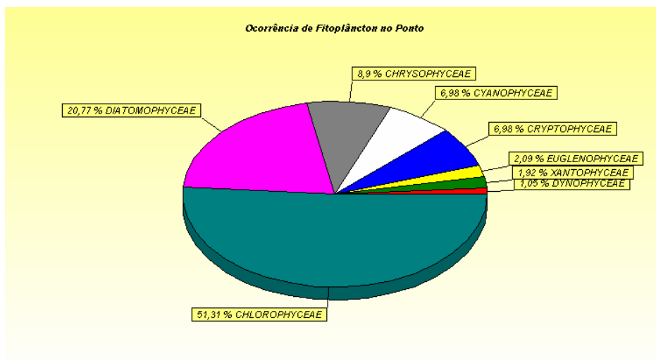
Fig 28. Abundância relativa dos principais grupos fitoplantônicos no ponto R1 (canal da represa sob a influência do Ribeirão do Lajeado), na Represa do Lajeado, TO, em junho de 2003.
