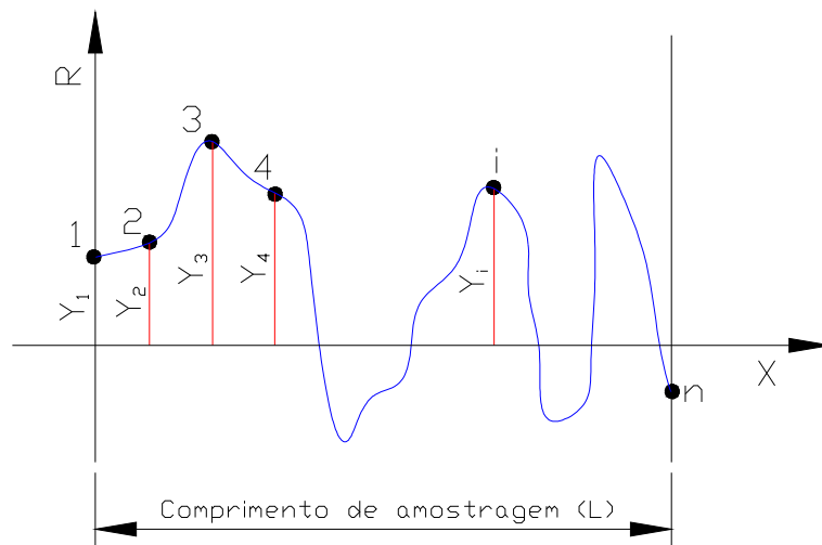
Figura 2.6 - Desvio médio aritmético R_a . Fonte: Agostinho, et al. (1990)
