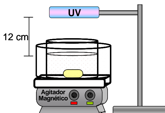
Figura 3.2 – Esquema do sistema reacional 1 usado nos experimentos para foto-Fenton
