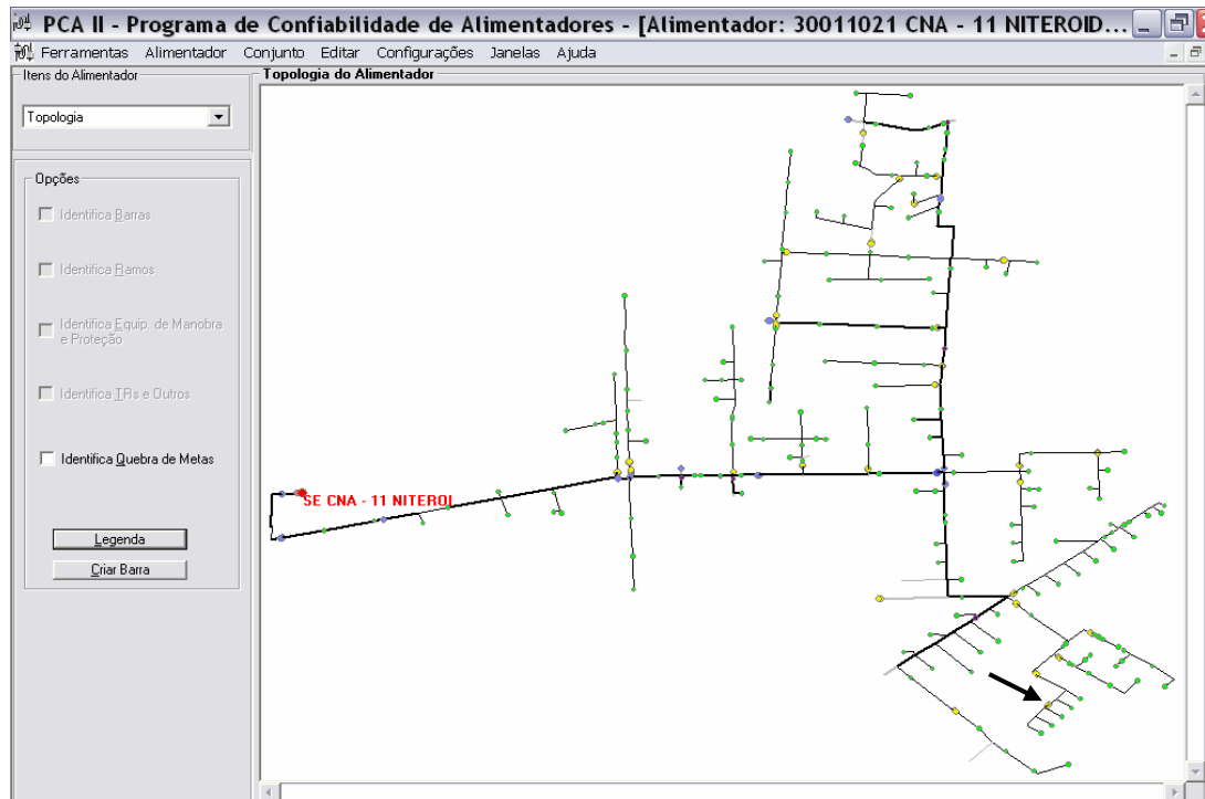
Figura 36 - Tela de apresentação da topologia normal do Alimentador.
