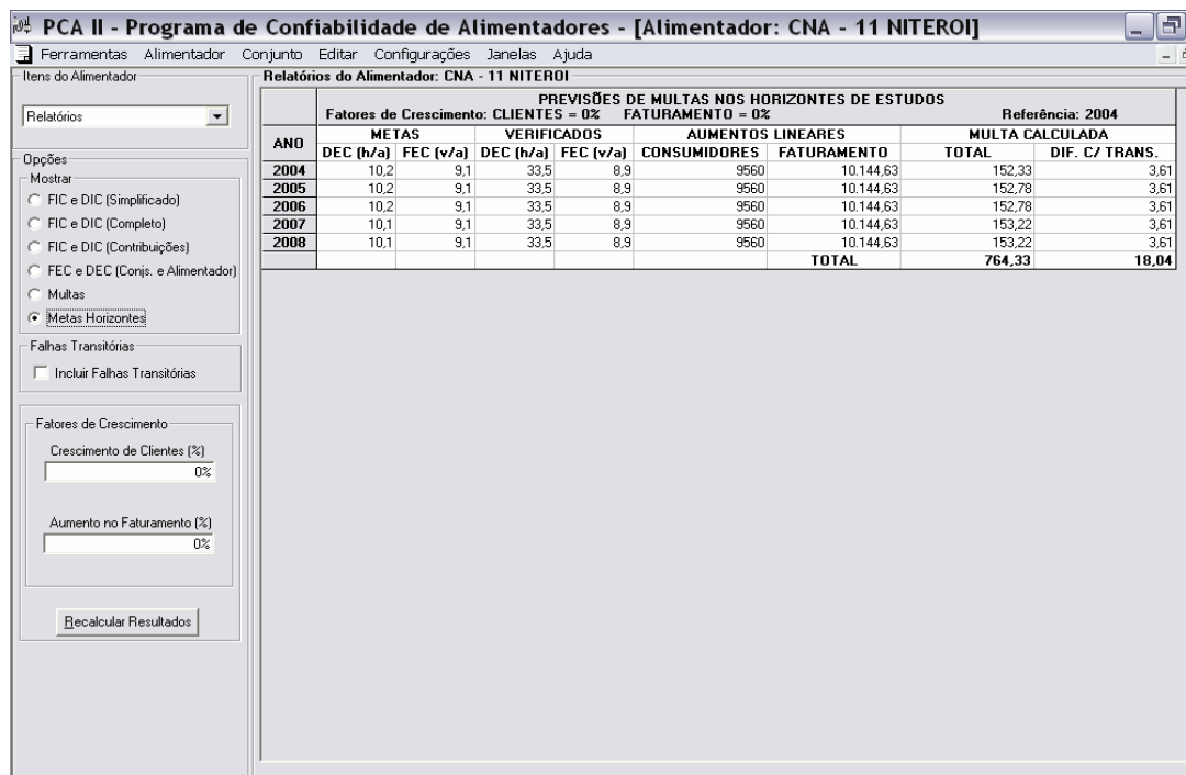
Figura 32 – Tela de apresentação do relatório. Opção selecionada: Metas Horizontes.
