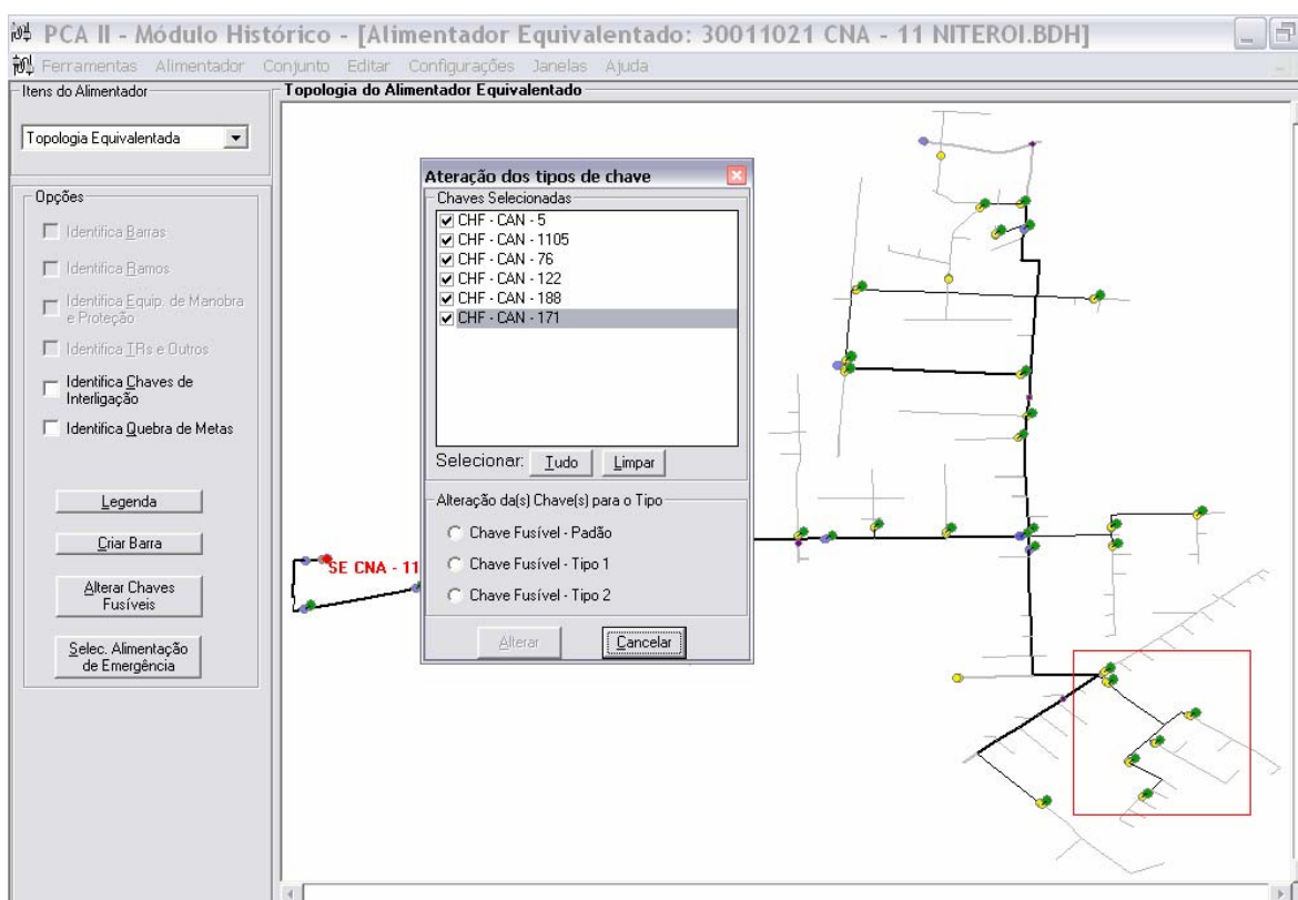
Figura 59 – Tela do Assistente para alteração de tipo de chave.
