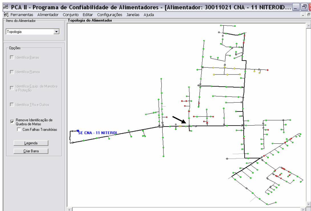
Figura 37 - Tela de apresentação da topologia do Alimentador com indicativos de quebra de metas dos pontos de carga (transformador).
