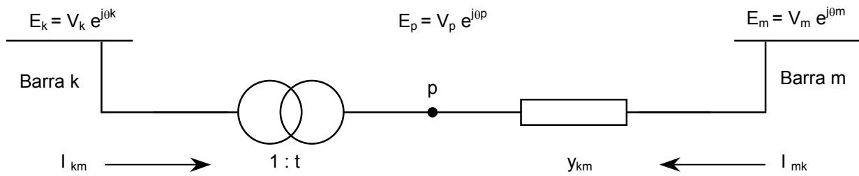
Fig. 3.2 Transformador em fase
