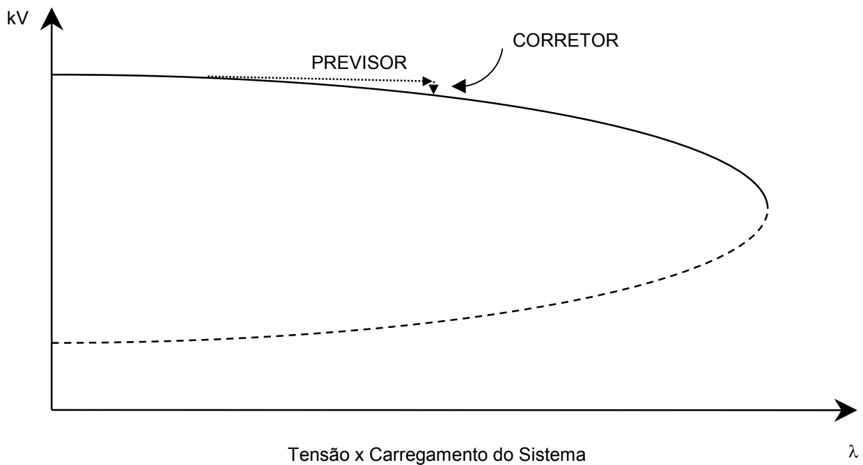
Fig. 4.1 – Método da Continuação
