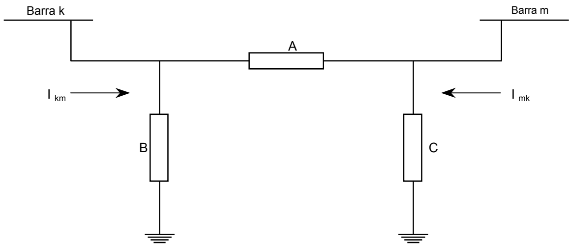
Fig. 3.3 – Modelo Pi do Transformador
