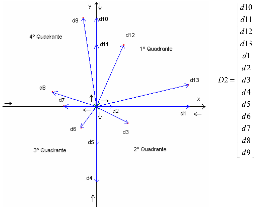
Figura 5.6: Geração do Vetor Distância das coordenadas rotacionadas de um ângulo \theta=90^\circ
