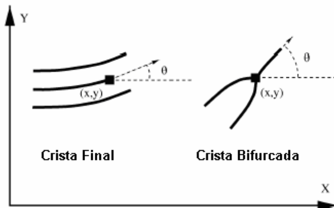
Figura 3.4: Componentes das minúcias (HONG et al , 1998b)
