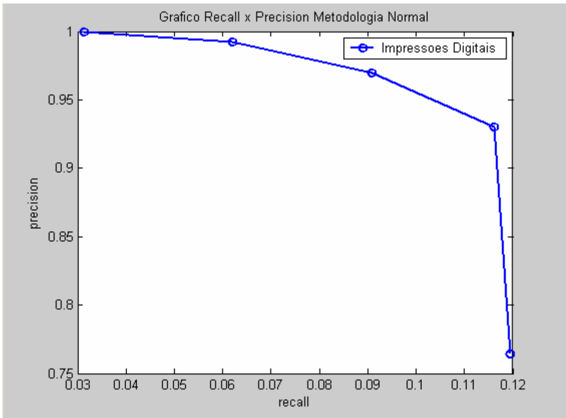
Figura 6.8: Gráfico Recall x Precision do Método Normal
