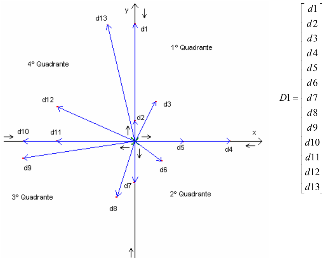
Figura 5.5: Geração do Vetor Distância ordenado do primeiro ao quarto quadrante
