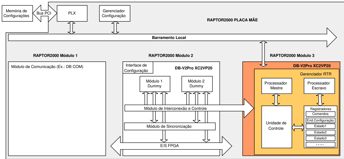
Figura 3.13: Diagrama de blocos da plataforma proposta por Griesel[14].
