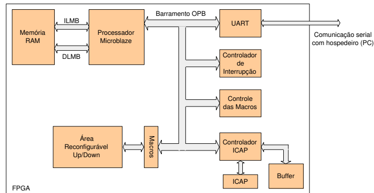
Figura 6.5: Diagrama em blocos do projeto Contador Up-Down.
