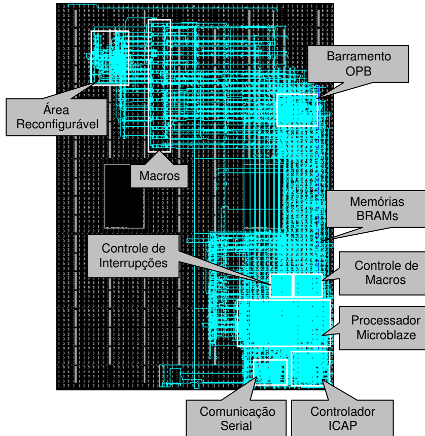
Figura 6.6: Leiaute resultante da síntese do projeto Contador Up-Down, conforme visualizado com a ferramenta FPGA Editor.
