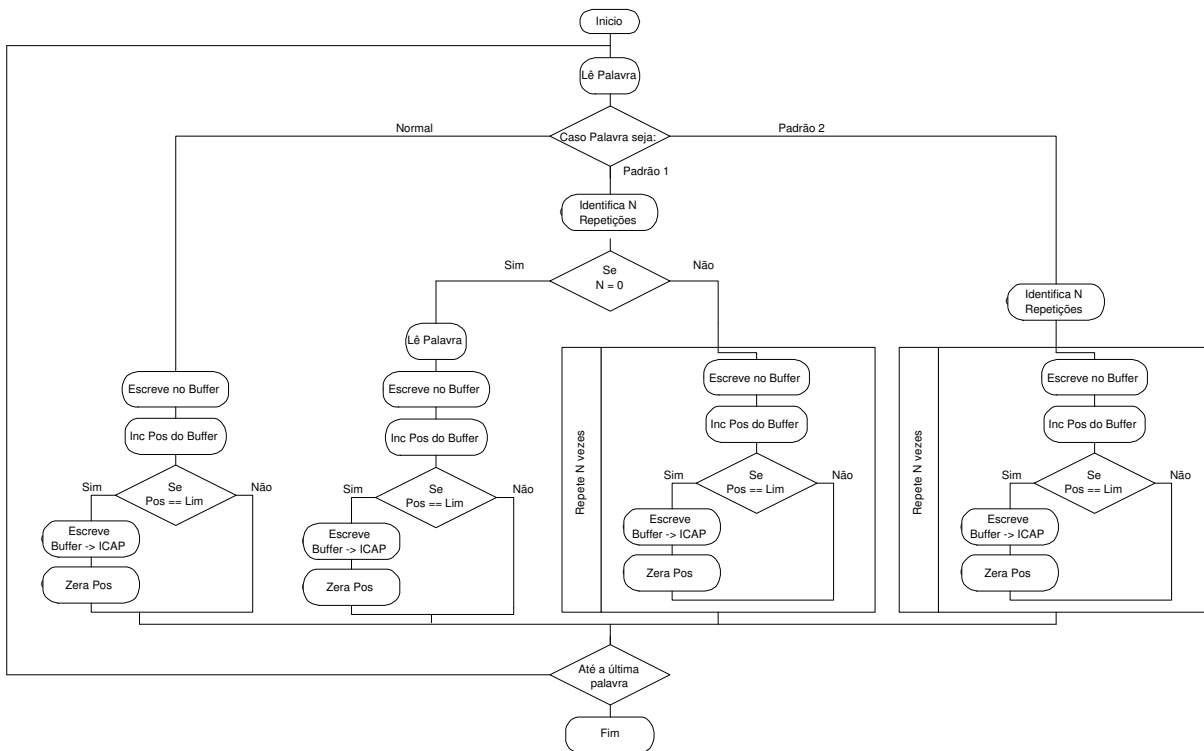
Figura 5.4: Fluxograma do algoritmo de descompactação de bitstreams utilizado no módulo Autoconfigurador do RSCM-S.
