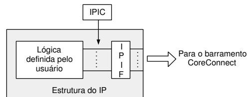
Figura 4.3: Estrutura do template de hardware gerado através do fluxo de criação de IPs do EDK.
