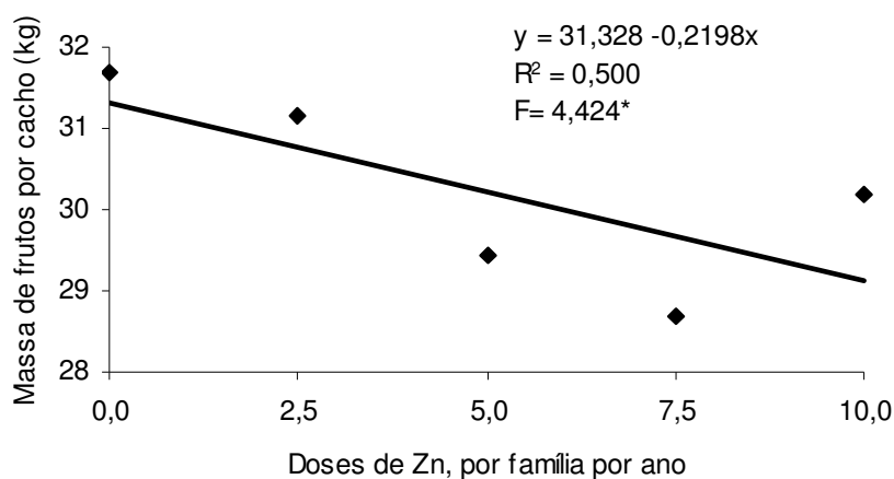
Figura 10. Massa de frutos do cacho de bananeira 'Prata-Anã', em resposta à aplicação de zinco, no terceiro ciclo de avaliação. Epamig/CTNM, Jaíba – 2006.
