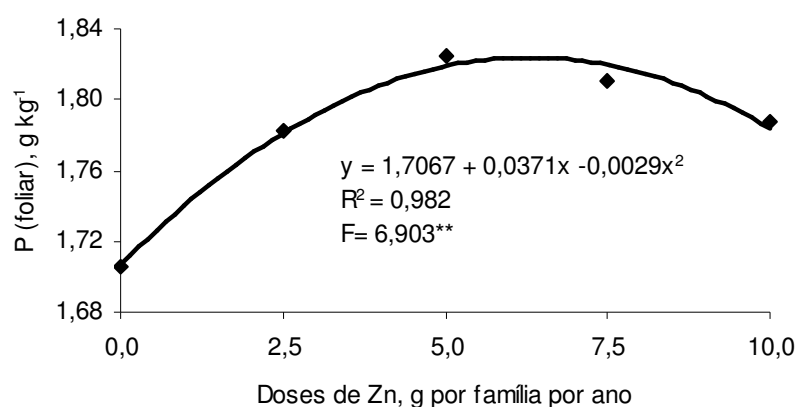
Figura 3. Teores foliares de fósforo em bananeira 'Prata-Anã', em resposta à aplicação de zinco, no primeiro ciclo de avaliação. Epamig/CTNM, Jaíba – 2006.
