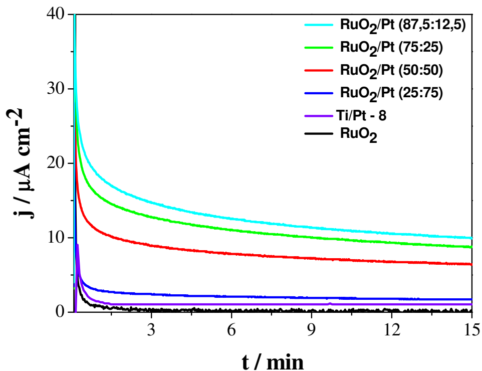
Figura 4.34 - Cronoamperometria de oxidação de metanol 0,5M em HClO 4 0,1M. E ox = 0,5 V. Eletrodos de Ti/RuO 2(x) Pt (1-x) e Ti/Pt - 8.
