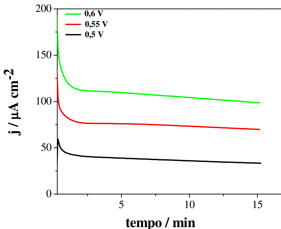
Figura 4.28 – Perfil cronoamperométrico da oxidação eletroquímica em diferentes potenciais. Ti/Pt - 8. E_{ox} = 0,5, 0,55 e 0,6\text{V} . t = 15\text{min} . Etanol 0,5\text{M} em \text{HClO}_4 0,1\text{M} . T = 25^\circ\text{C} .
