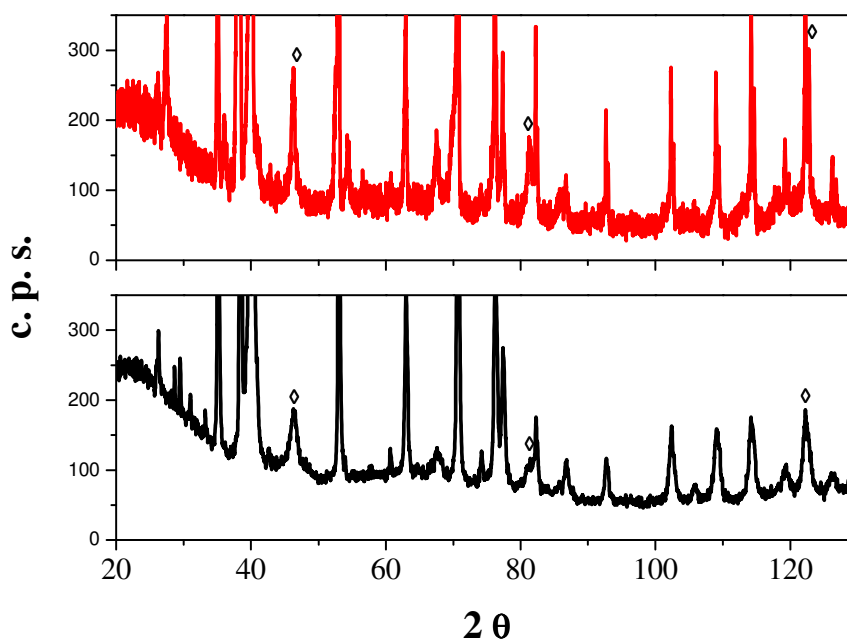
Figura 4.7 – Difrátogramas dos eletrodos de Ti/Pt preparados por 3 camadas das resinas: (3) 1:8:64. ◊ Pt. ___ 300 °C e ___ 600 °C.
