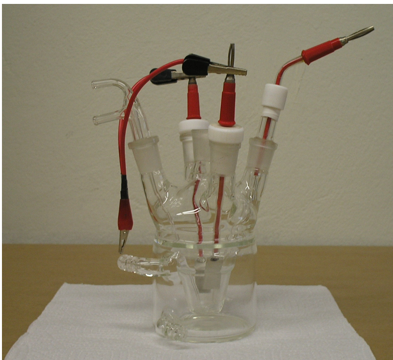
Figura 3.3 – Célula eletroquímica convencional de três eletrodos.
