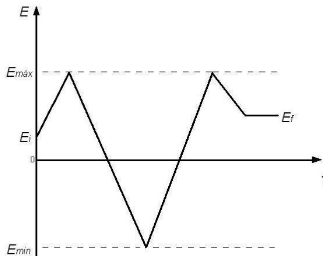
Figura 3.6 – Variação do potencial aplicado com o tempo em voltametria cíclica, mostrando o potencial inicial, E_i , o potencial final, E_f , os potenciais máximos, E_{\max} , e mínimo, E_{\min} . A velocidade de varredura |dE / dt| = v .
