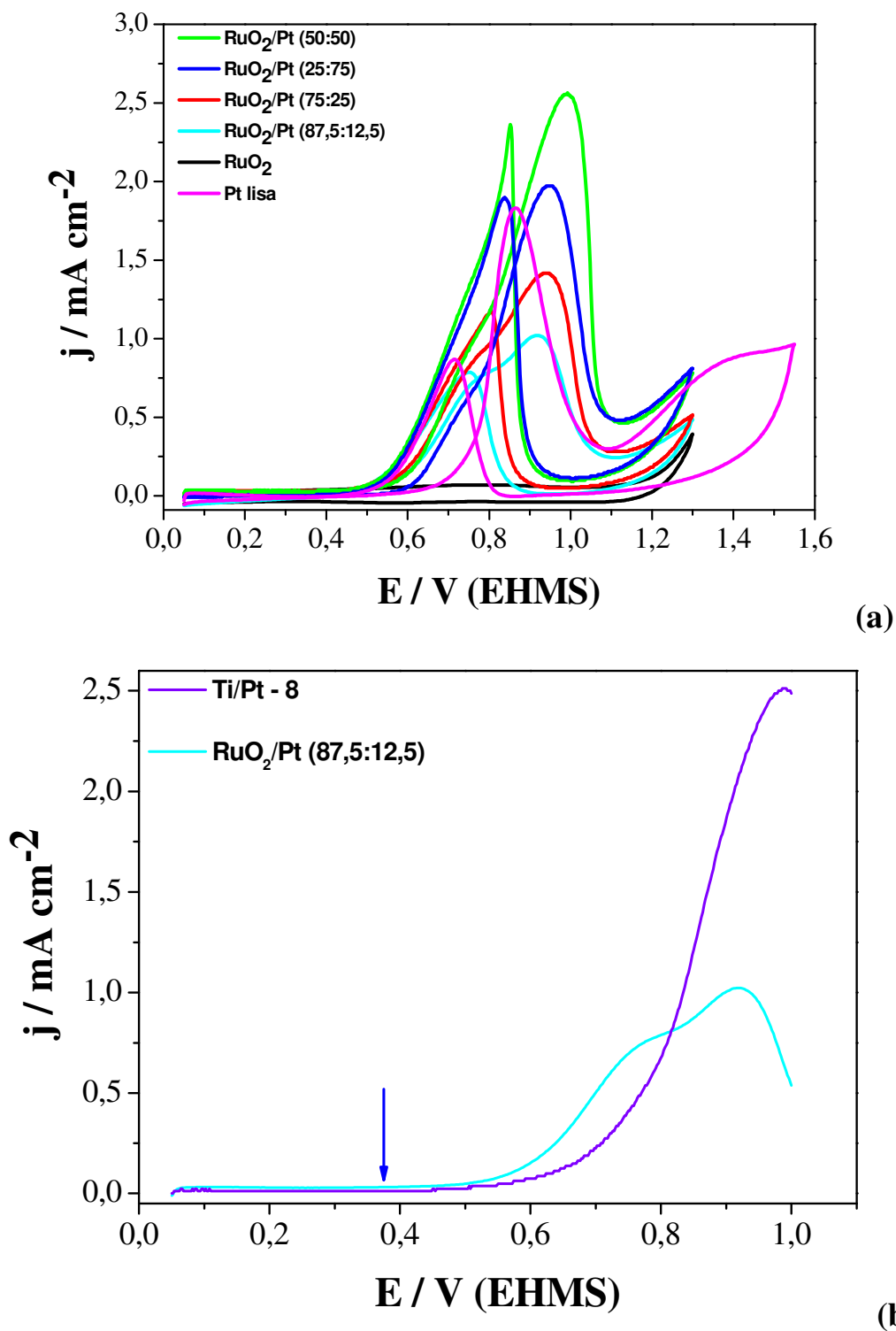
Figura 4.33 - Voltamograma cíclico de oxidação metanol 0,5M em \text{HClO}_4 0,1M à 50 \text{ mV s}^{-1} . a) \text{Ti/RuO}_2_{(x)}\text{Pt}_{(1-x)} e b) \text{Ti/Pt} - 8 e \text{Ti/RuO}_2_{(x)}\text{Pt}_{(1-x)} (87,5:12,5).
