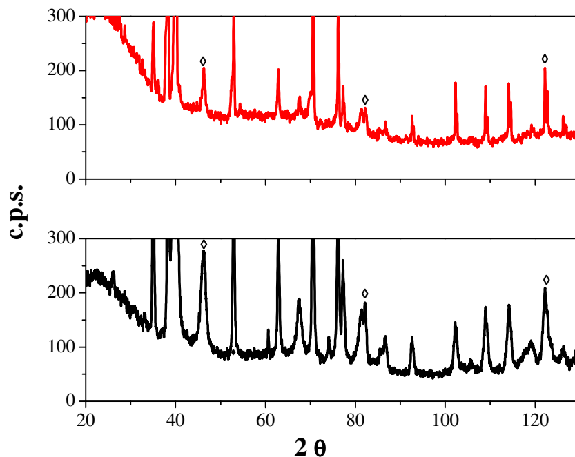
Figura 4.6 – Difrátogramas dos eletrodos de Ti/Pt preparados por 3 camadas das resinas: (2) 1:12:48. ◊ Pt. ___ 300 °C e ___ 600 °C.
