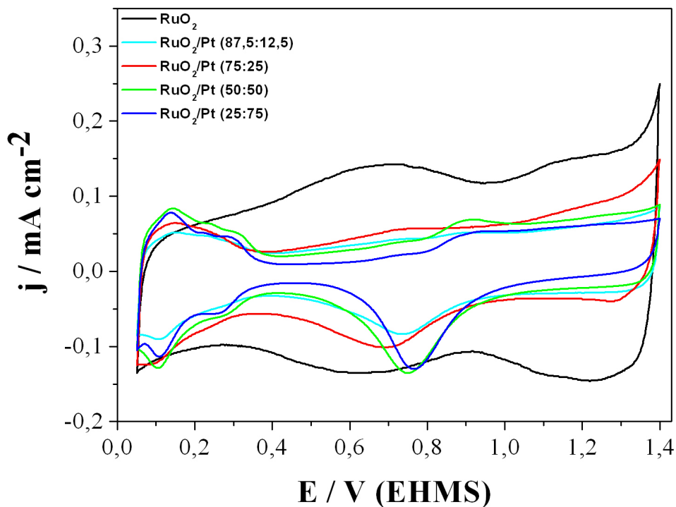
Figura 4.32 - Voltamogramas cíclicos de caracterização dos eletrodos \text{Ti/RuO}_{2(x)}\text{Pt}_{(1-x)} em \text{HClO}_4 0,1M. v = 50 \text{ mV s}^{-1} . T = 25 \text{ }^\circ\text{C} .
