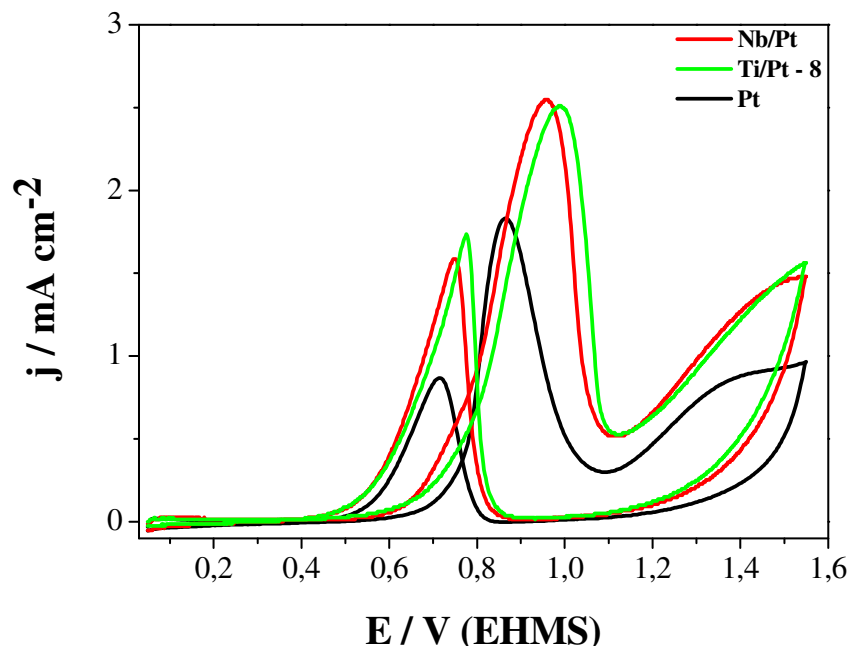
Figura 4.23 - Perfil voltamétrico da oxidação eletroquímica de metanol 0,5M à v=50 \text{ mV s}^{-1} em meio de \text{HClO}_4 0,1M sobre Pt, Ti/Pt - 8 e Nb/Pt. T = 25 \text{ }^\circ\text{C} .
