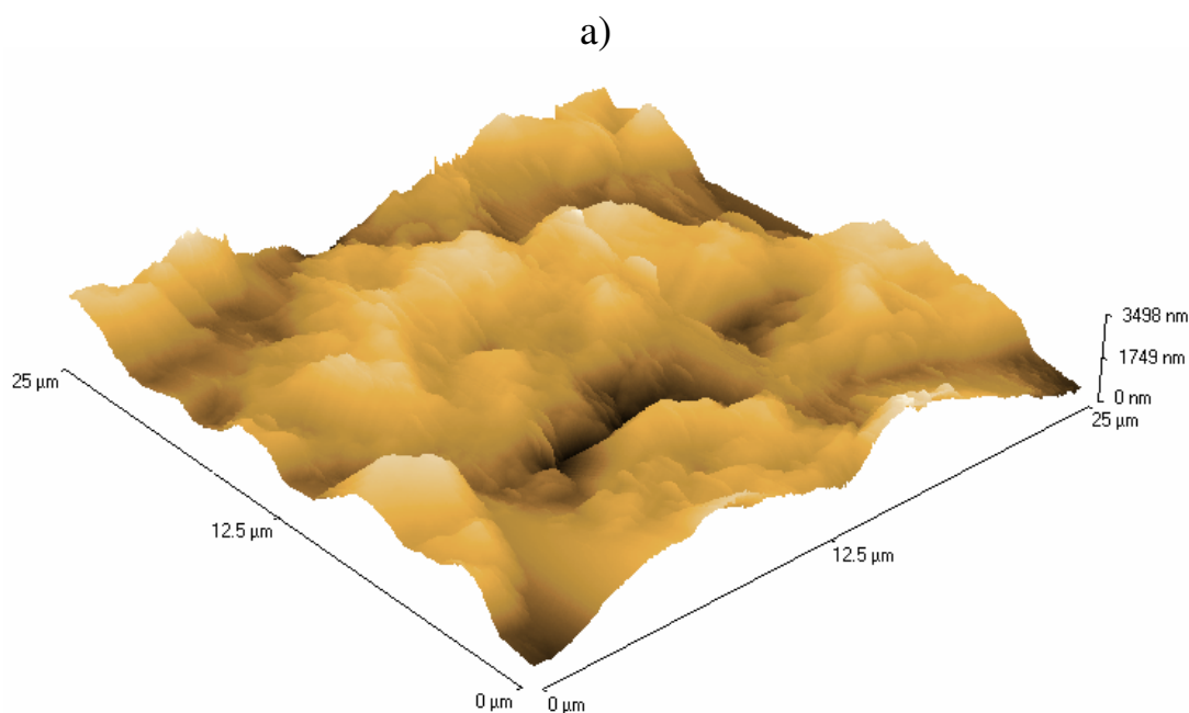
Figura 4.16 – Imagens tridimensionais de microscopia de força atômica. a) Ti jateado b) Ti/Pt, 3 camadas, solução precursora 1:12:96 (Pt:AC:EG), tratados termicamente a 600 °C.
