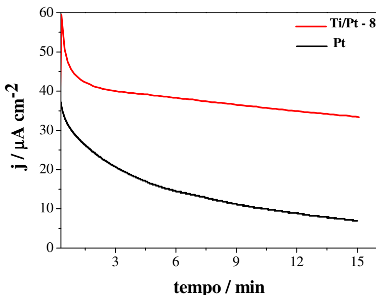
Figura 4.27 - Perfil cronoamperométrico da oxidação eletroquímica de etanol 0,5M em HClO 4 0,1M em Pt e Ti/Pt - 8. E_{ox} = 0,5V . t = 15min .
