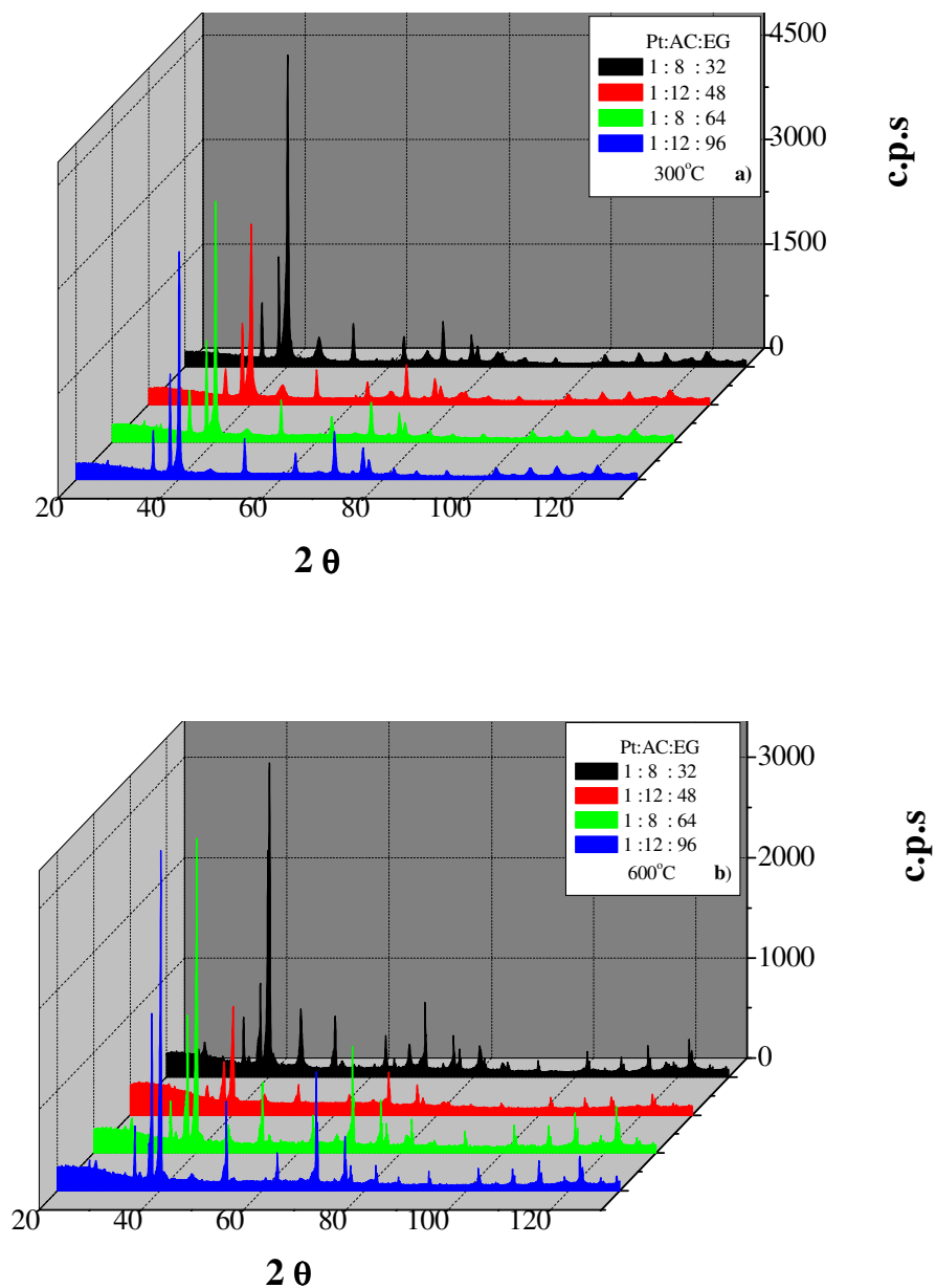
Figura 4.9 - Difractogramas dos eletrodos de Ti/Pt tratados termicamente a 300 (a) e 600 °C (b) preparados por 3 camadas.
