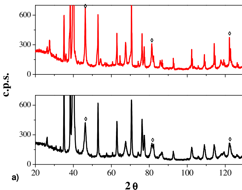
Figura 4.5 – Difratogramas dos eletrodos de Ti/Pt preparados por 3 camadas das resinas: (1) 1:8:32. \diamond Pt. ___ 300 °C e ___ 600 °C.
