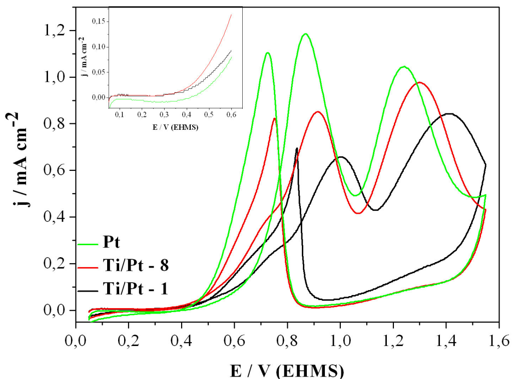
Figura 4.26 – Perfil voltamétrico da oxidação eletroquímica de etanol 0,5M em meio de HClO 4 0,1M sobre Pt e Ti/Pt. v = 20 \text{ mV s}^{-1} e T = 25 \text{ }^\circ\text{C} .
