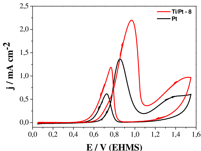
Figura 4.19 – Perfil voltamétrico da oxidação eletroquímica de metanol 0,5M em meio de \text{HClO}_4 0,1M sobre Pt e Ti/Pt - 8. v = 20 \text{ mV s}^{-1} e T = 25 \text{ }^\circ\text{C} .
