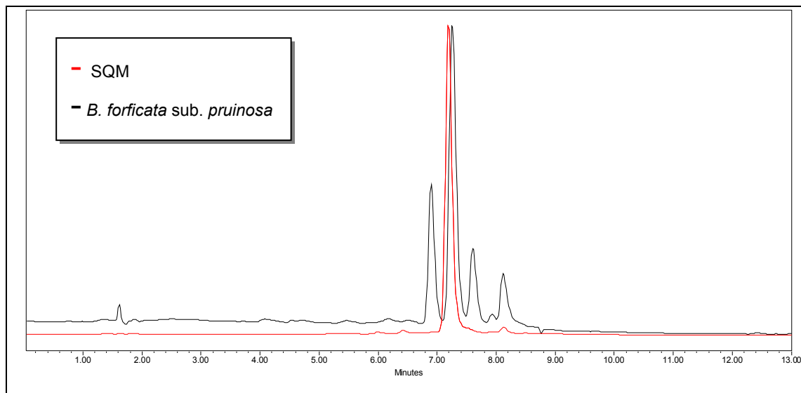
Figura 4.2. Cromatograma de Bauhinia forficata subespécie pruinosa , sobreposto com a substância química majoritária (SQM) isolada a partir de extrato butanólico de suas folhas, a 348 nm.
