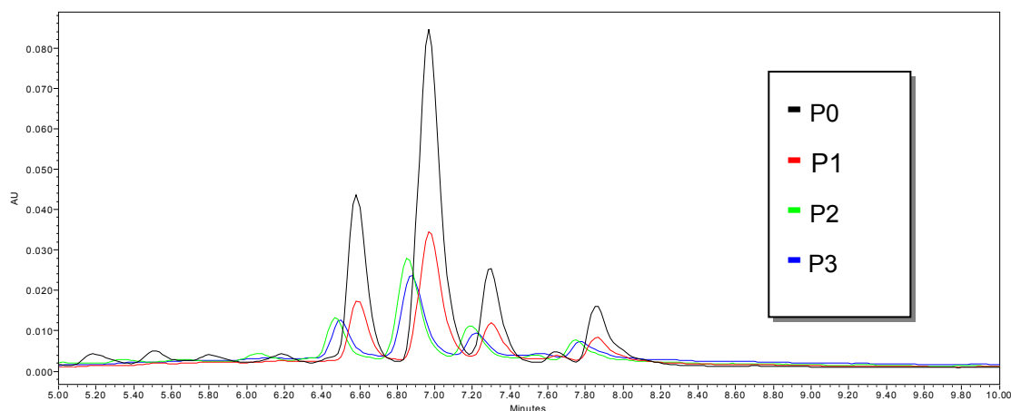
Figura 6.2. Cromatograma demonstrando o decaimento sistemático dos compostos presentes em Bauhinia forficata subespécie pruinosa no decorrer da análise de estabilidade.
