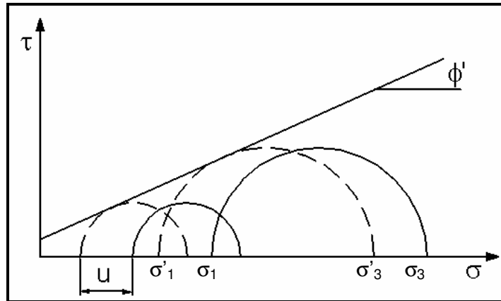
Figura 3.10 – Envoltória de resistência
