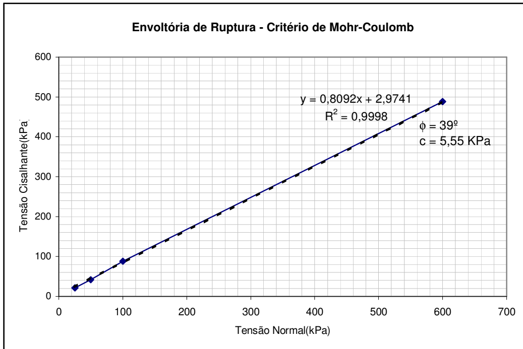
Figura 5.14 – Tensão Cisalhante x Tensão Normal – amostra acinzentada.
