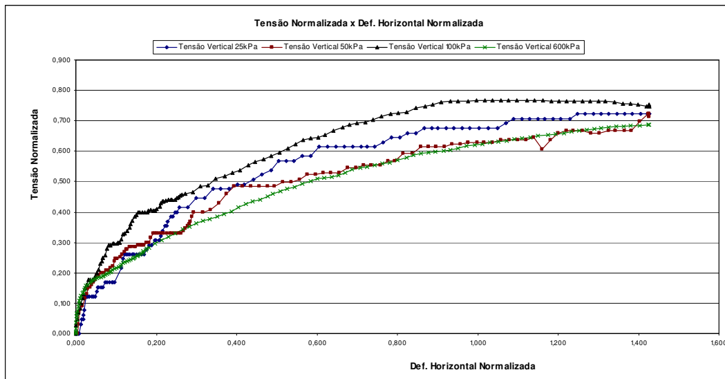
Figura 5.12 – Tensão Cisalhante Normalizada x Deslocamento Horizontal Normalizado – amostra acinzentada.
