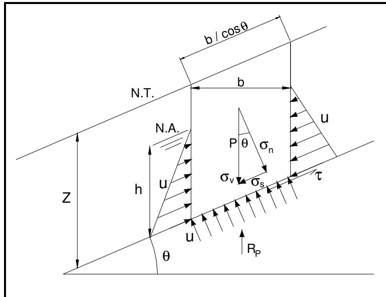
Figura 3.12 – Forças atuantes em um talude de terra com percolação de água.
