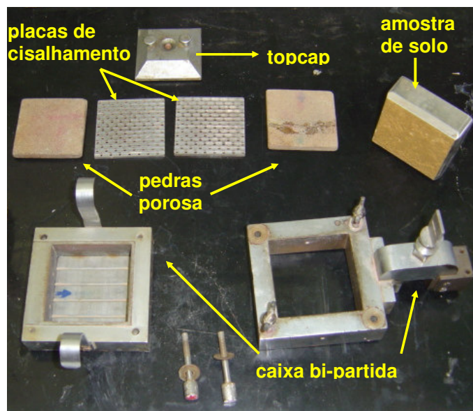
Figura 5.4 - Caixa de cisalhamento direto.
