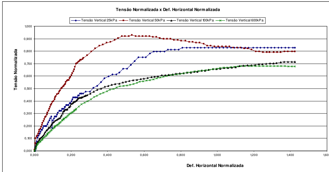
Figura 5.9 – Tensão Cisalhante Normalizada x Deslocamento Horizontal Normalizado – amostra amarelada.
