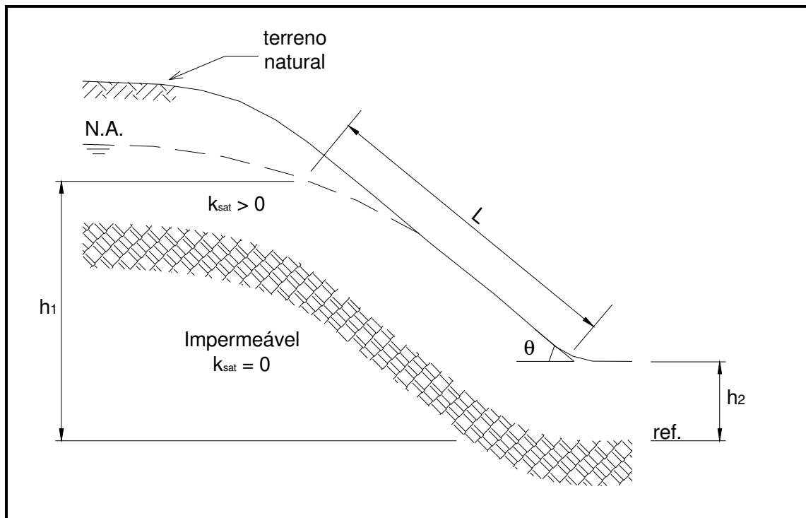
Figura 3.16 – Esquema representativo do regime permanente ao longo de uma encosta.
