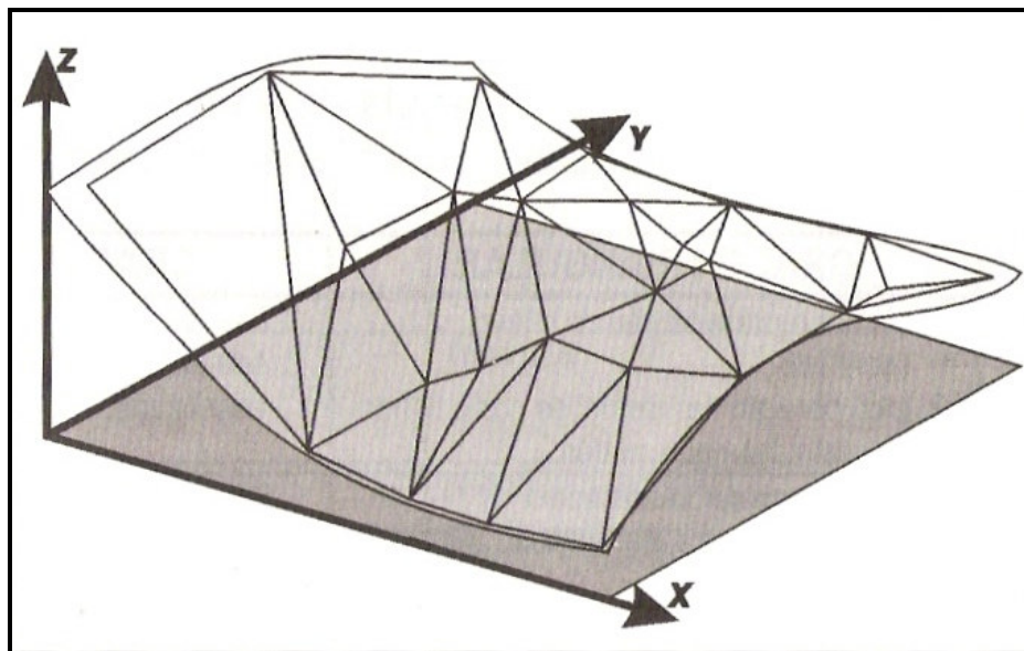
Figura 3.9 – Superfície e malha triangular correspondente (NAMIKAWA, 1995 apud ROCHA, 2002).
