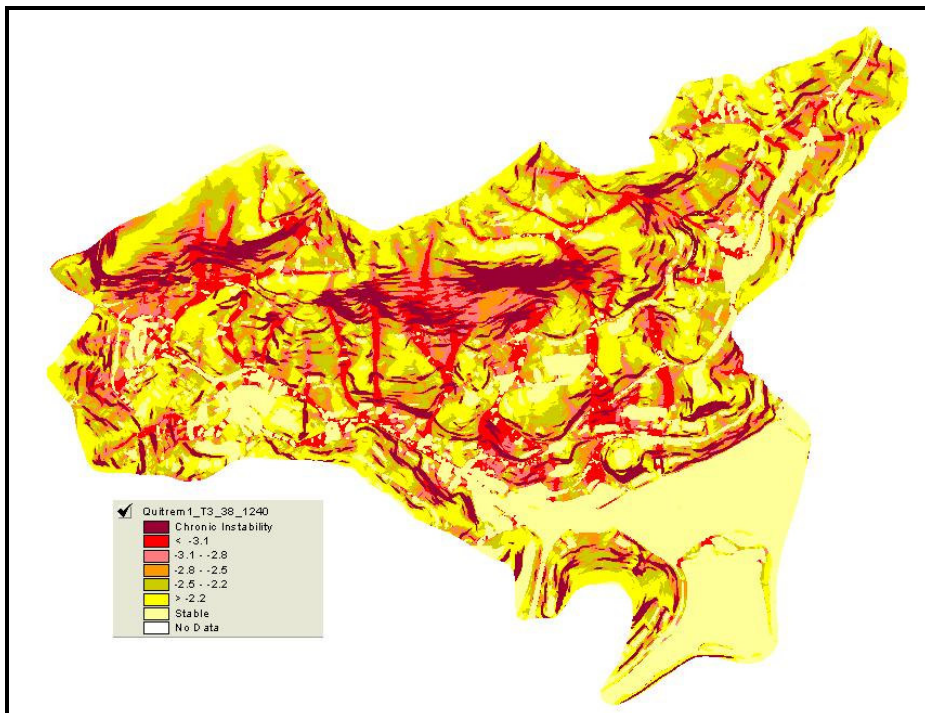
Figura 6.3 – Mapa resultante do modelo Shalstab considerando-se a Situação 03.
