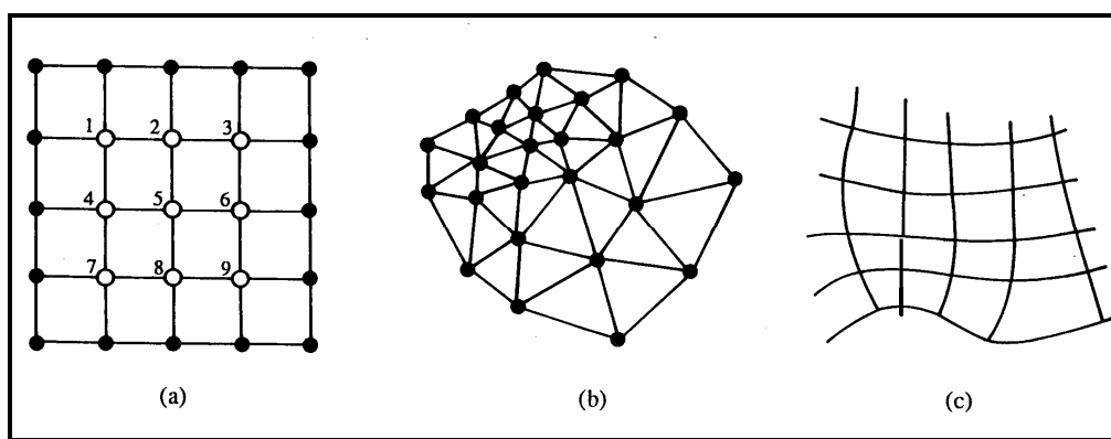
Figura 3.7 – Métodos de geração do MDE (MOORE et al. , 1993).
