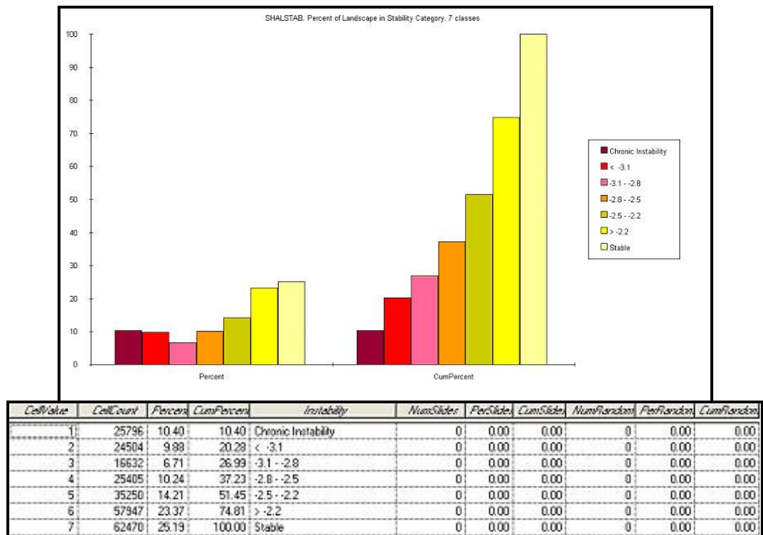
Figura 6.9 – Resultado do modelo SHALSTAB para a Situação 03.
