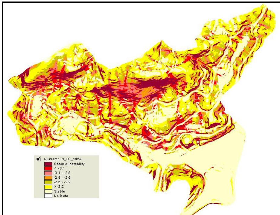
Figura 6.1 – Mapa resultante do modelo Shalstab considerando-se a Situação 01.
