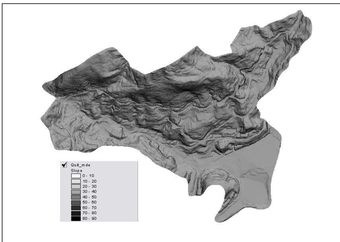
Figura 5.20 – Modelo Digital de Declividade (MDD).
