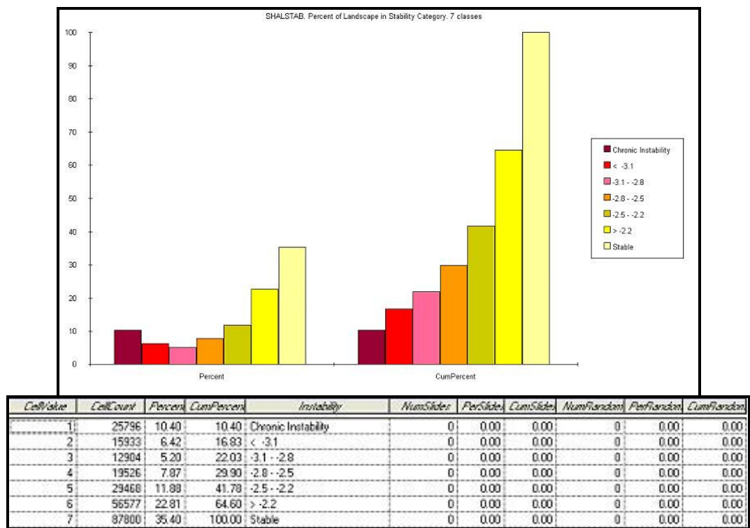
Figura 6.7 – Resultado do modelo SHALSTAB para a Situação 01.
