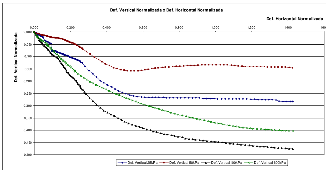
Figura 5.10 – Deslocamento Vertical Normalizado x Deslocamento Horizontal Normalizado – amostra amarelada.
