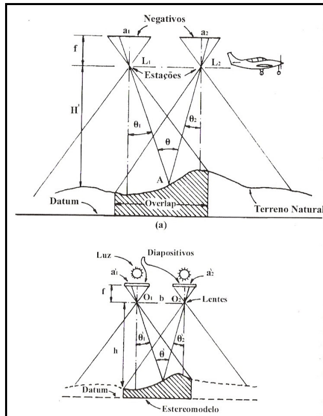
Figura 3.3 – Conceito básico de restituidores (WOLF, 1983 apud ROCHA, 2002).
