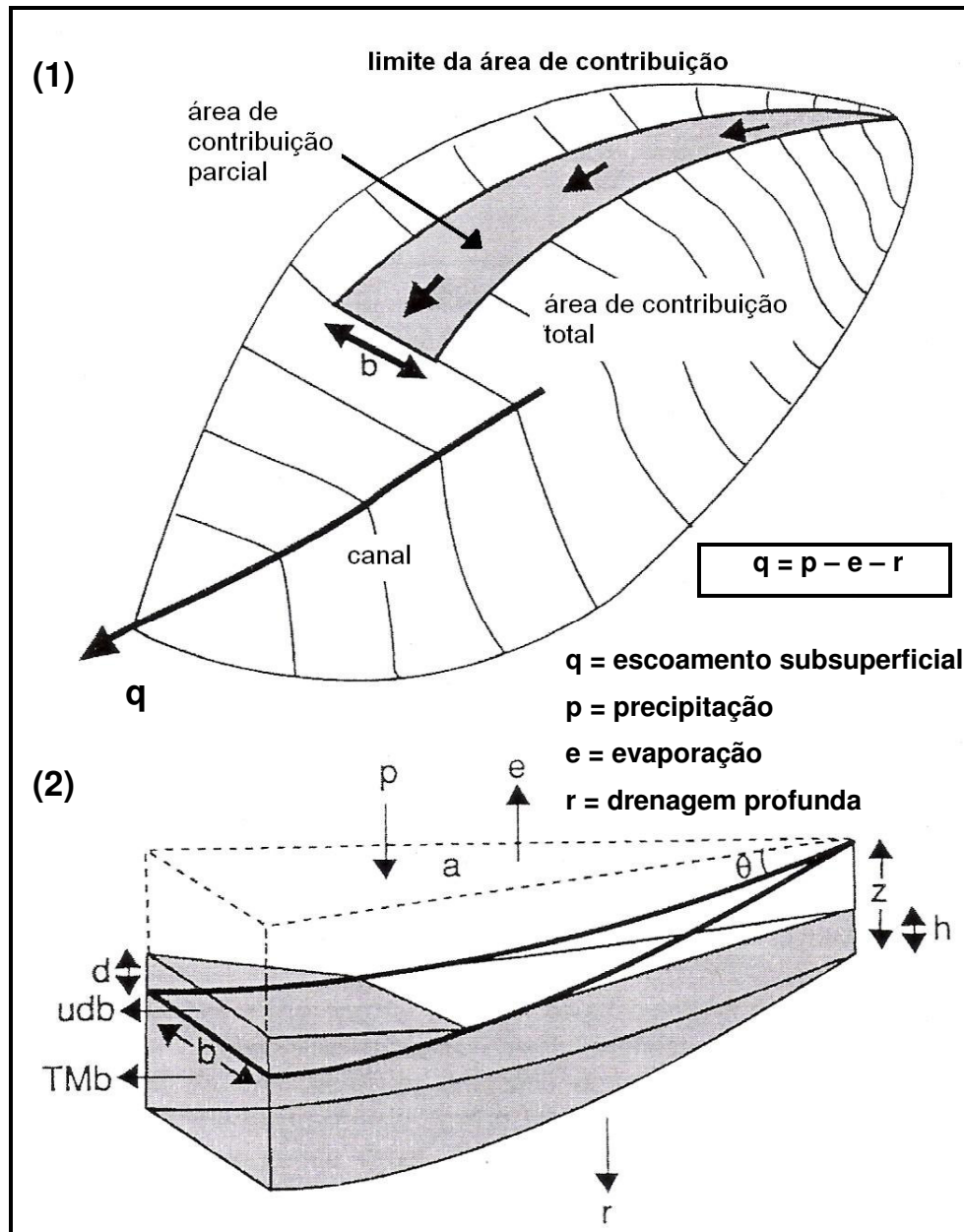
Figura 3.15 – Vista superior (1) e seção longitudinal (2) da área de drenagem ao longo do comprimento unitário b (modificada de DIETRICH et al. , 1993).
