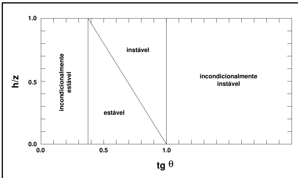
Figura 3.13 – Condição de estabilidade do talude de acordo com a relação entre a inclinação do talude ( \text{tg} \theta ) e o valor da taxa de umedecimento do solo ( h/z ), para um solo com \phi = 45^\circ e \rho_{\text{nat}}/\rho_w = 1,6 (modificado de MONTGOMERY & DIETRICH, 1998).
