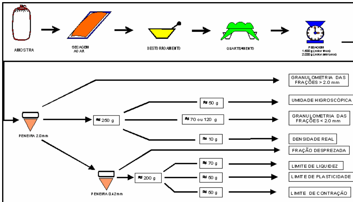
Figura 5.18 – Metodologia para a realização de ensaios de caracterização (IME, 1998).
