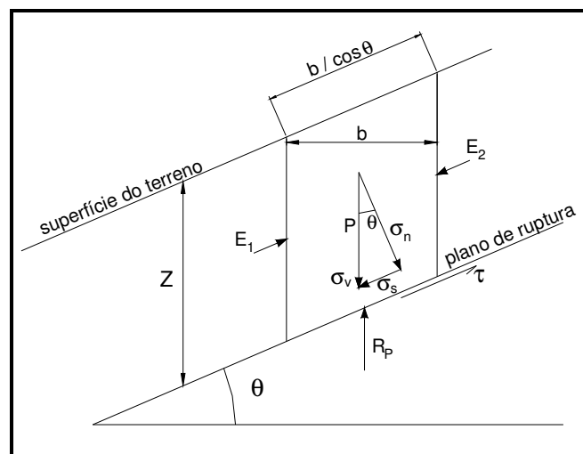
Figura 3.11 – Forças atuantes em um talude de terra sem percolação de água ( h=0 ).
