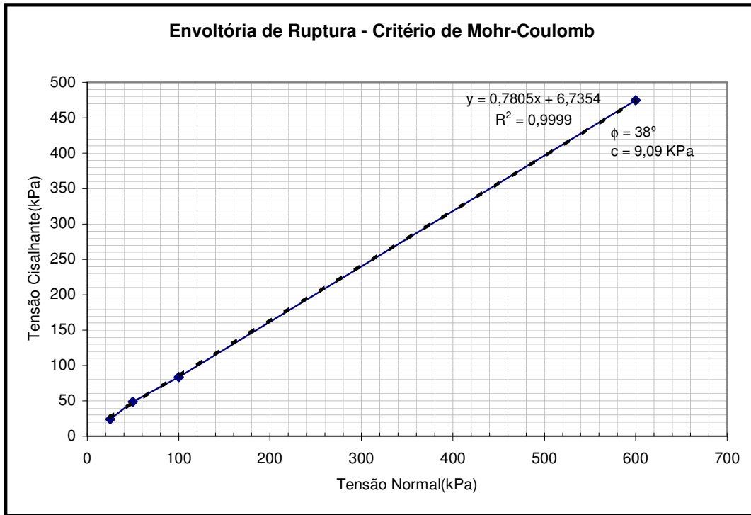
Figura 5.11 – Tensão Cisalhante x Tensão Normal – amostra amarelada.
