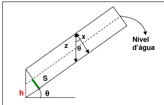
Figura 3.17 – Bloco esquemático de uma camada de solo, onde S é a área da seção transversal saturada e h é a altura da coluna d'água.
