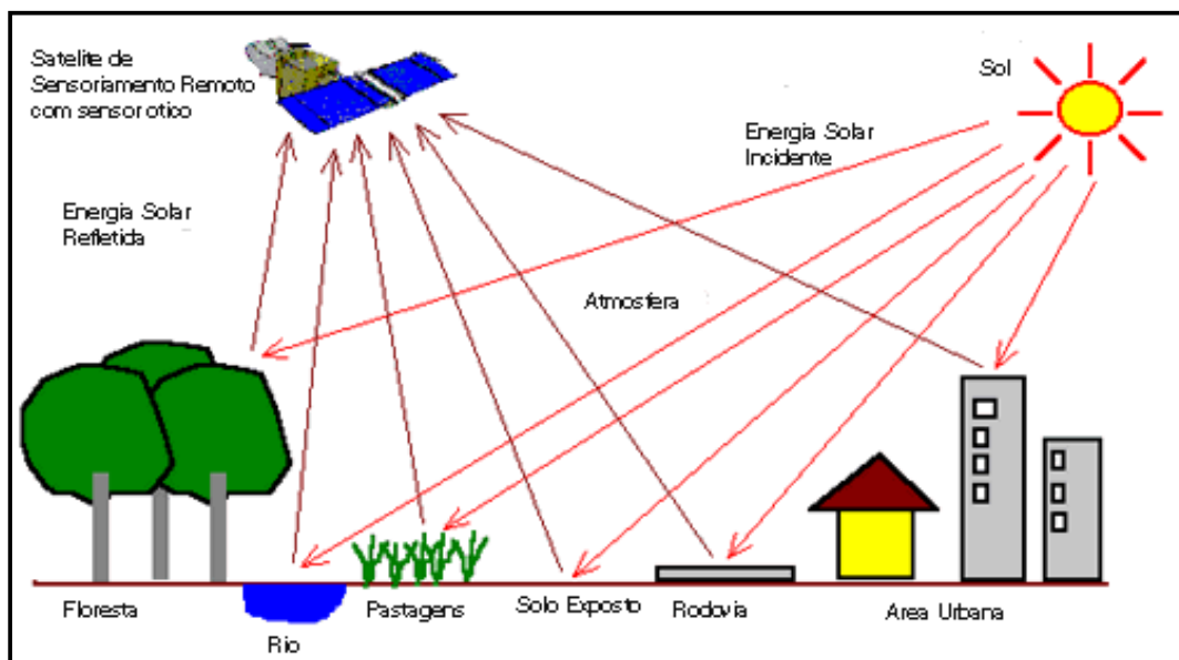
Figura 3.6 –Sistema de Sensoriamento Remoto (LNCC,2003).
