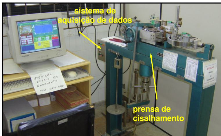
Figura 5.7 – Visão geral do equipamento e sistema de aquisição de dados para o ensaio de cisalhamento direto.
