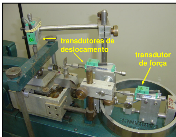
Figura 5.8 – Visão geral dos transdutores.
