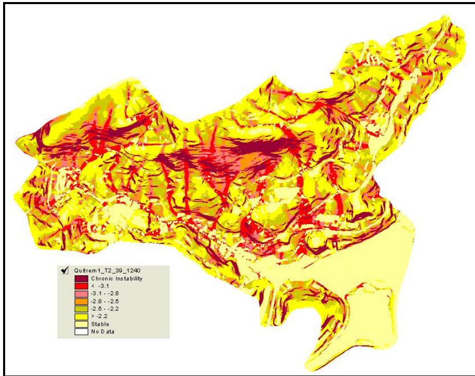
Figura 6.2 – Mapa resultante do modelo Shalstab considerando-se a Situação 02.
