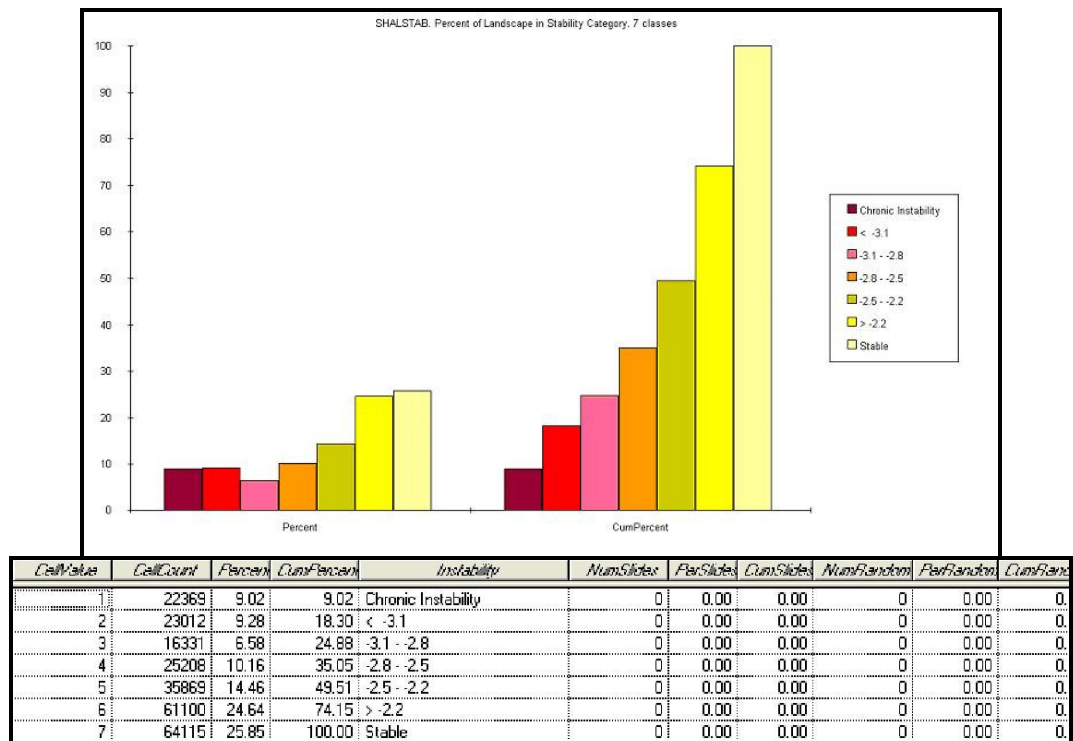
Figura 6.8 – Resultado do modelo SHALSTAB para a Situação 02.
