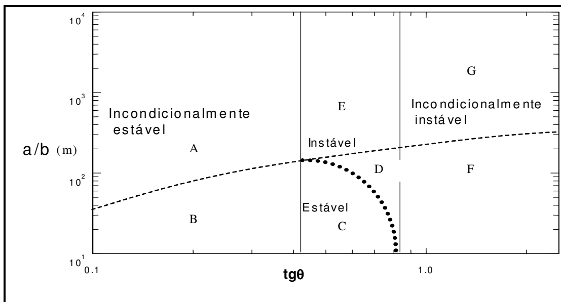
Figura 3.18 – Razão a/b em função da tg\theta (eixos em logaritmo). A linha tracejada representa o limite de saturação e a linha pontilhada é definida a partir dos valores obtidos pela equação 3.26 (GUIMARÃES, 2000 apud MONTGOMERY & DIETRICH, 1998).
