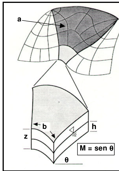
Figura 3.14 – Esquema da área de contribuição à montante a (área hachurada) que escoia através do comprimento b (modificado de MONTGOMERY & DIETRICH, 1994).
