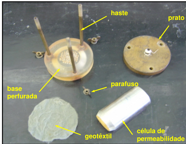
Figura 5.17 – Componentes do permeâmetro.
