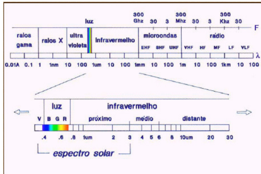
Figura 4. Espectro Eletromagnético.
