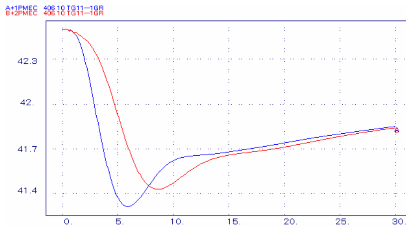
Figura 5.40 – Potência mecânica da unidade a gás.
