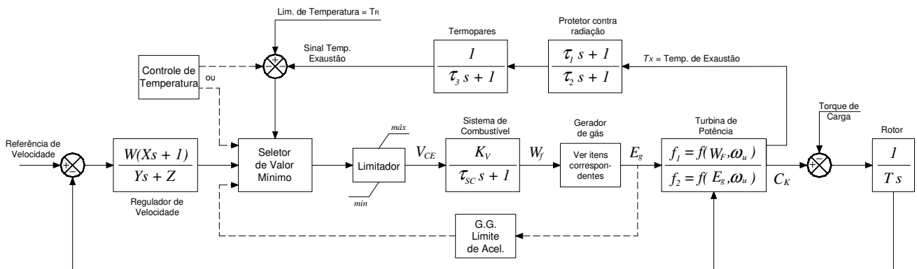
Figura 4.27 – Diagrama de blocos representativo da turbina aeroderivativa com múltiplos eixos.
