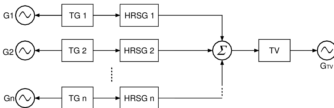
Figura 4.49 – Diagrama da configuração geral de múltiplos eixos da operação em ciclo combinado.
