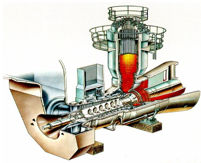
Figura 2.2 – Turbina a gás Alstom GT8C (Turbina Heavy-Duty ).
