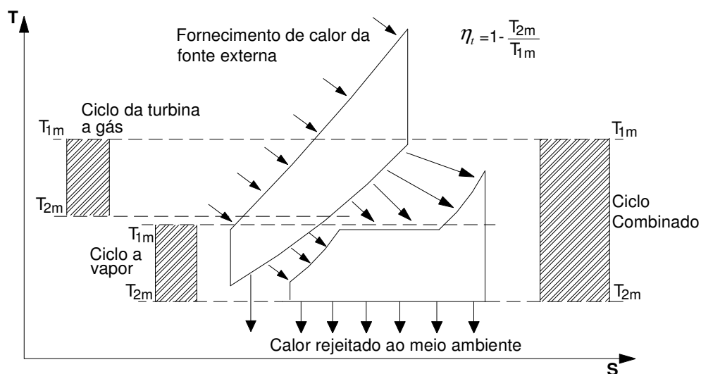
Figura 1.4 – Representação nas coordenadas T-s do ciclo equivalente de Carnot para uma instalação de ciclo combinado gás – vapor.
