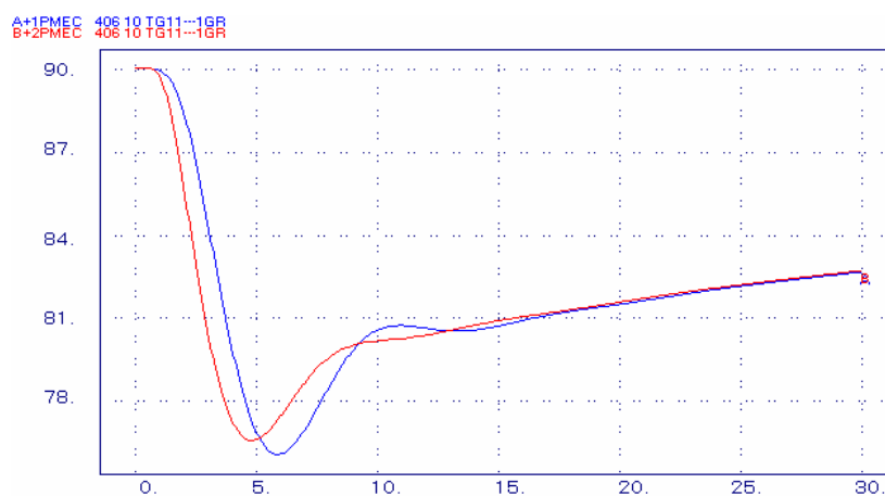
Figura 5.10 – Potência mecânica da unidade a gás.
