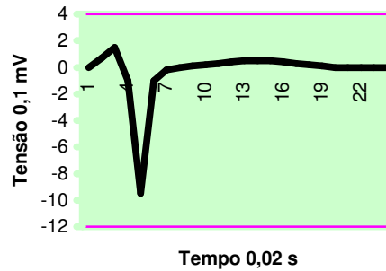
Derivação avr
