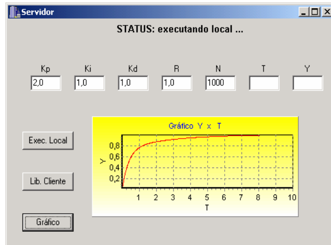
Figura 5.3 - Interface gráfica do módulo servidor.
