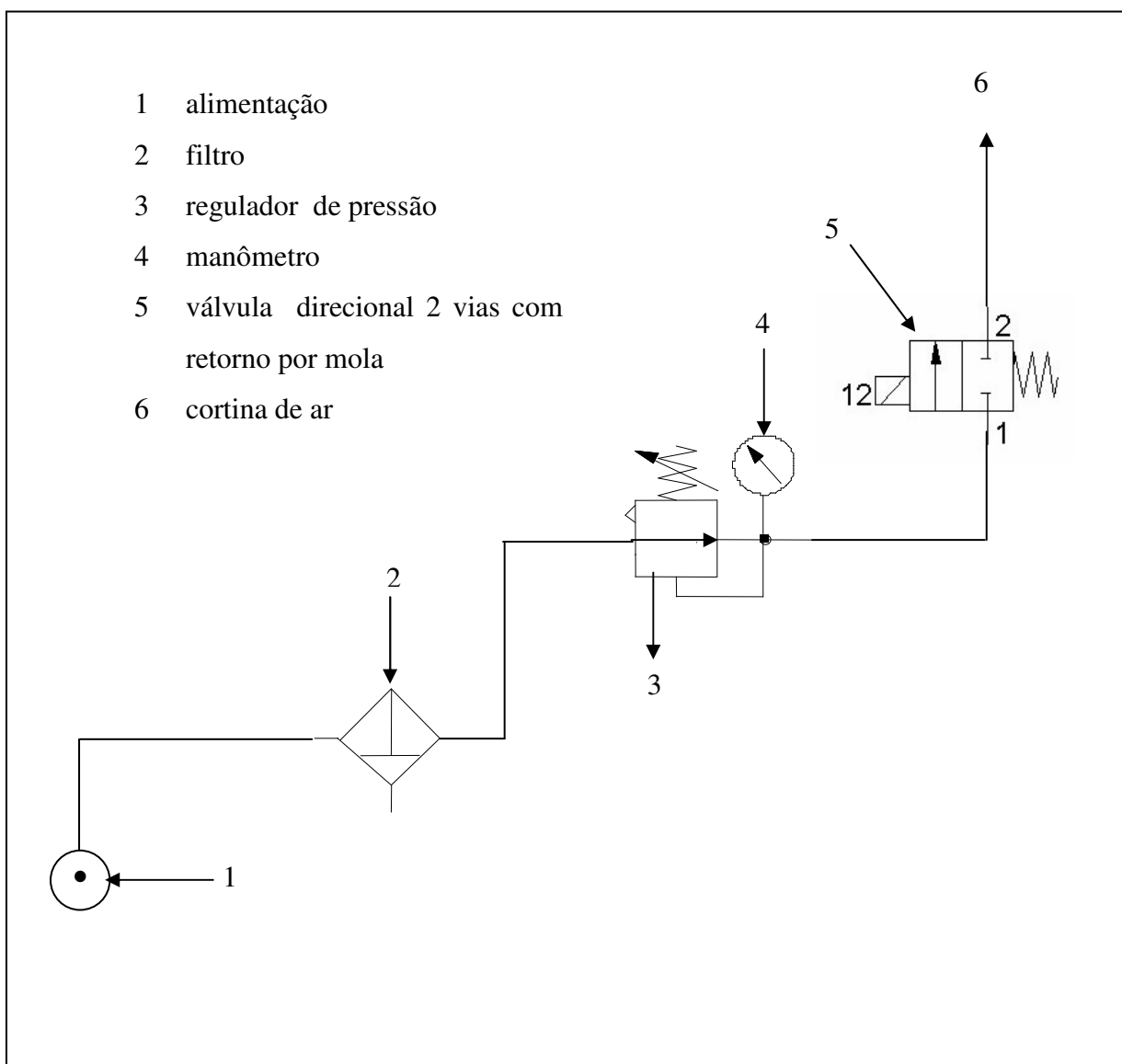
Figura 4.11 – Circuito do ar comprimido
