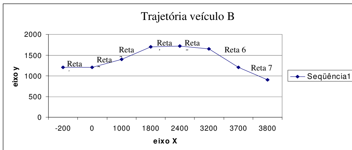
Gráfico 6.2 – Trajetória do veículo B
