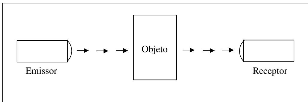
Figura 6.3 – Funcionamento do sensor óptico por barreira
