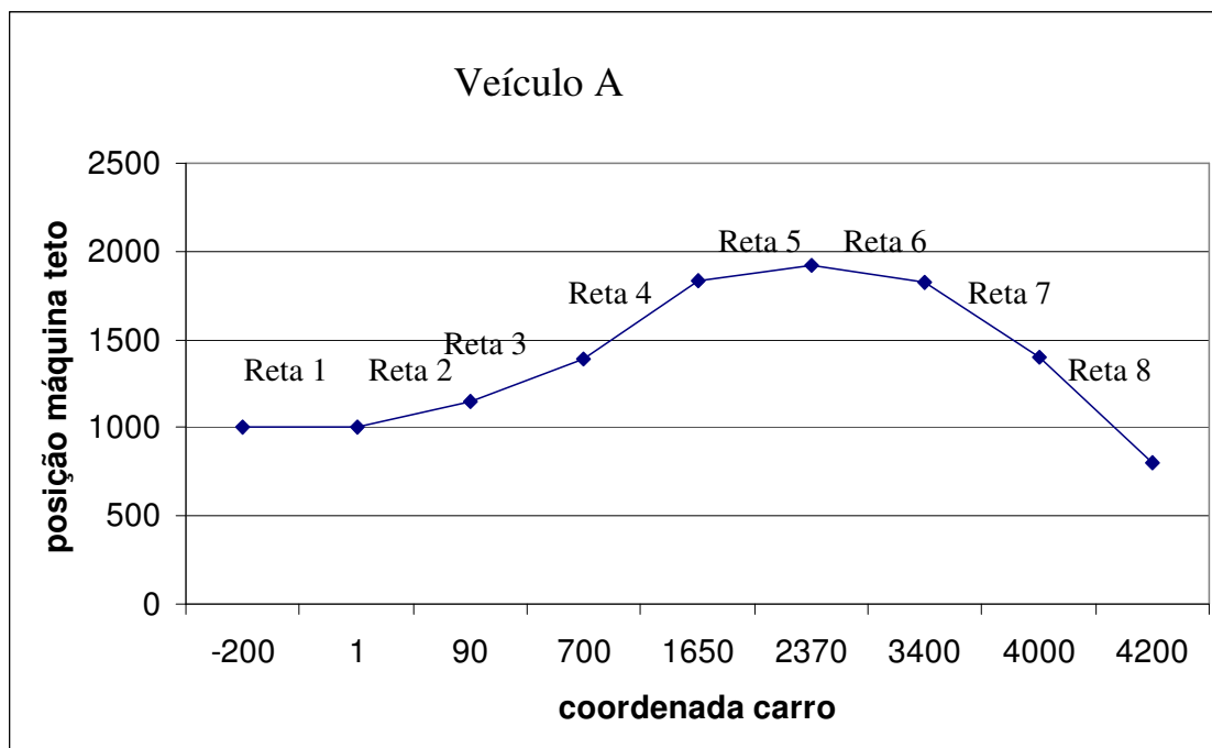
Gráfico 6.1 – Trajetória veículo A
