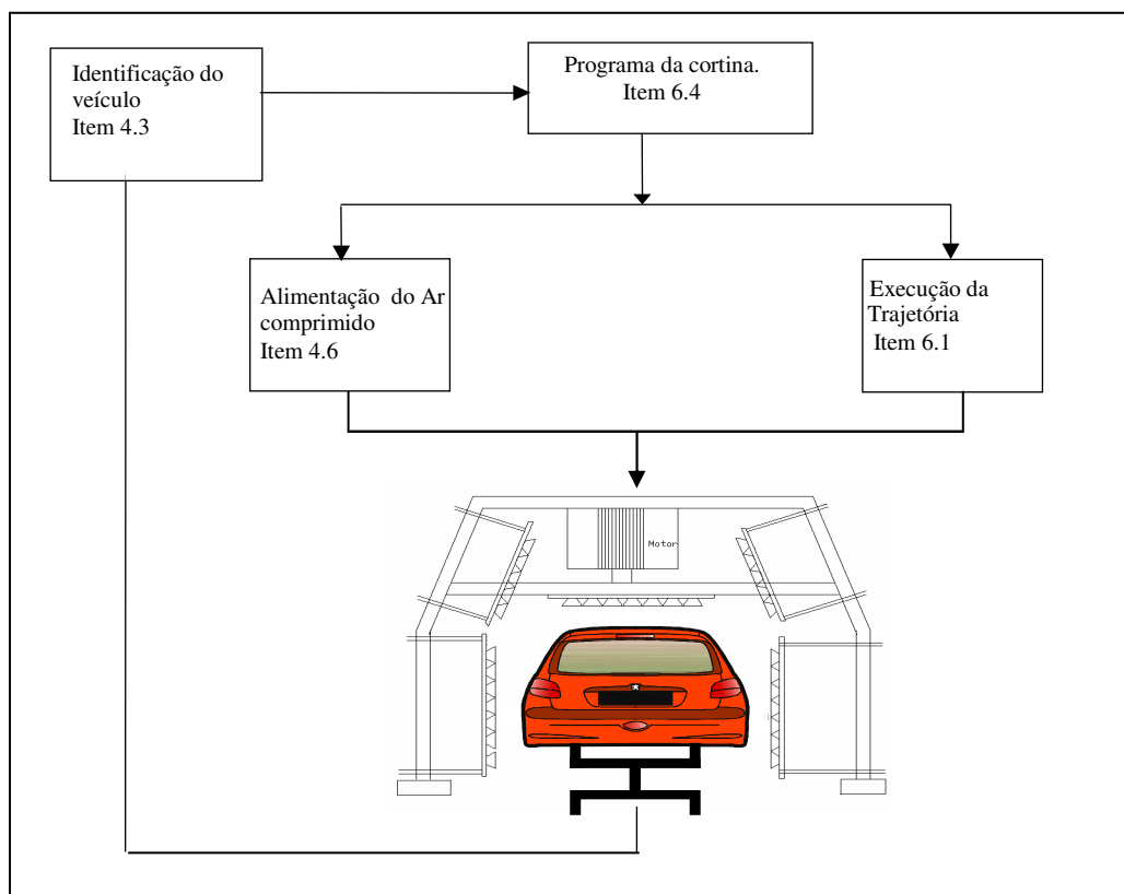
Figura 4.4 – Comunicação do sistema
