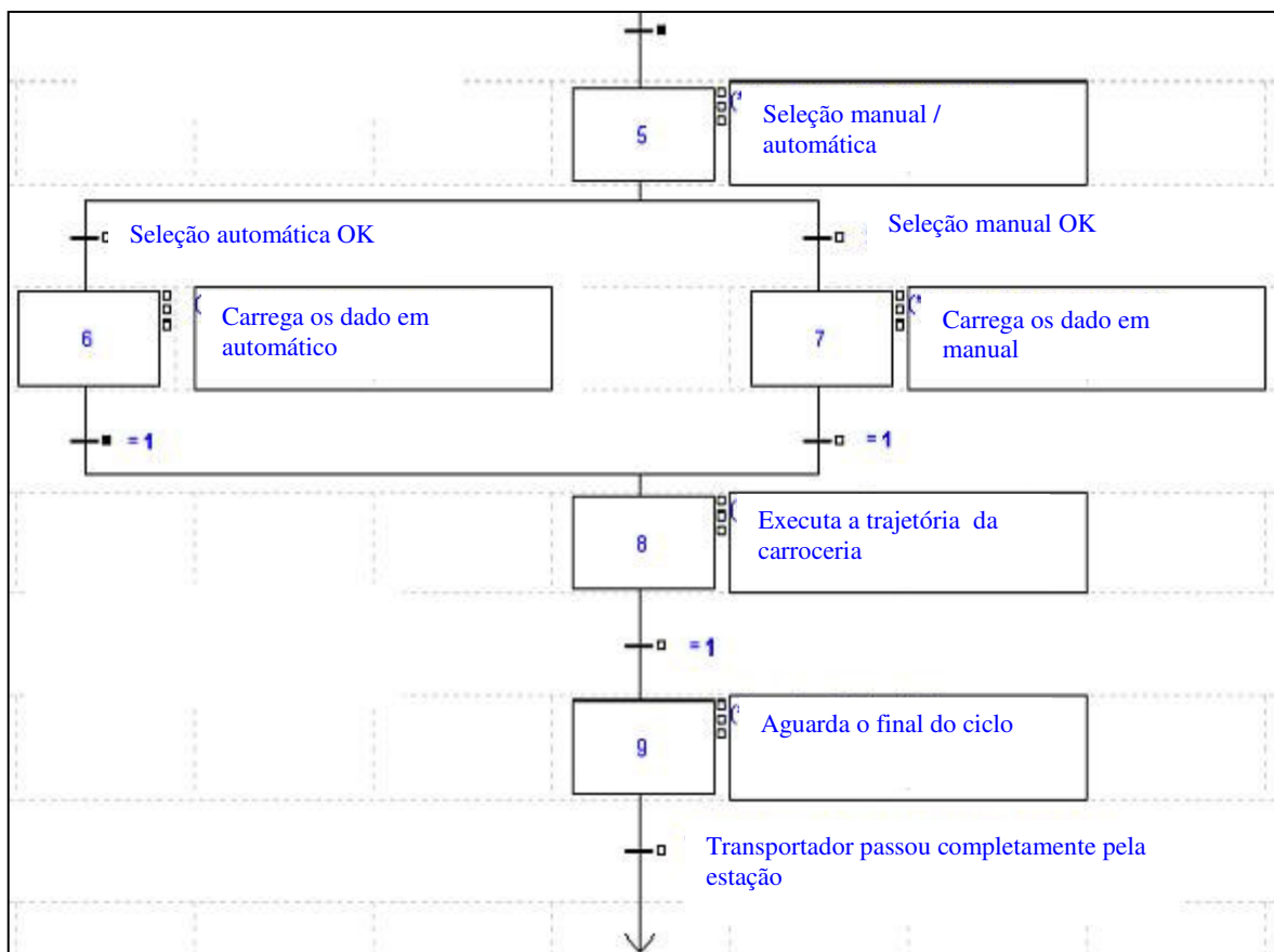
Figura 5.8 – “Grafcet” do sistema de funcionamento da cortina em manual e automático (tela do programa PL7 PRO da Schneider )
