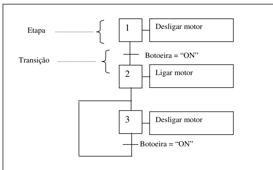
Figura 5.1 – Aplicação Grafcet
