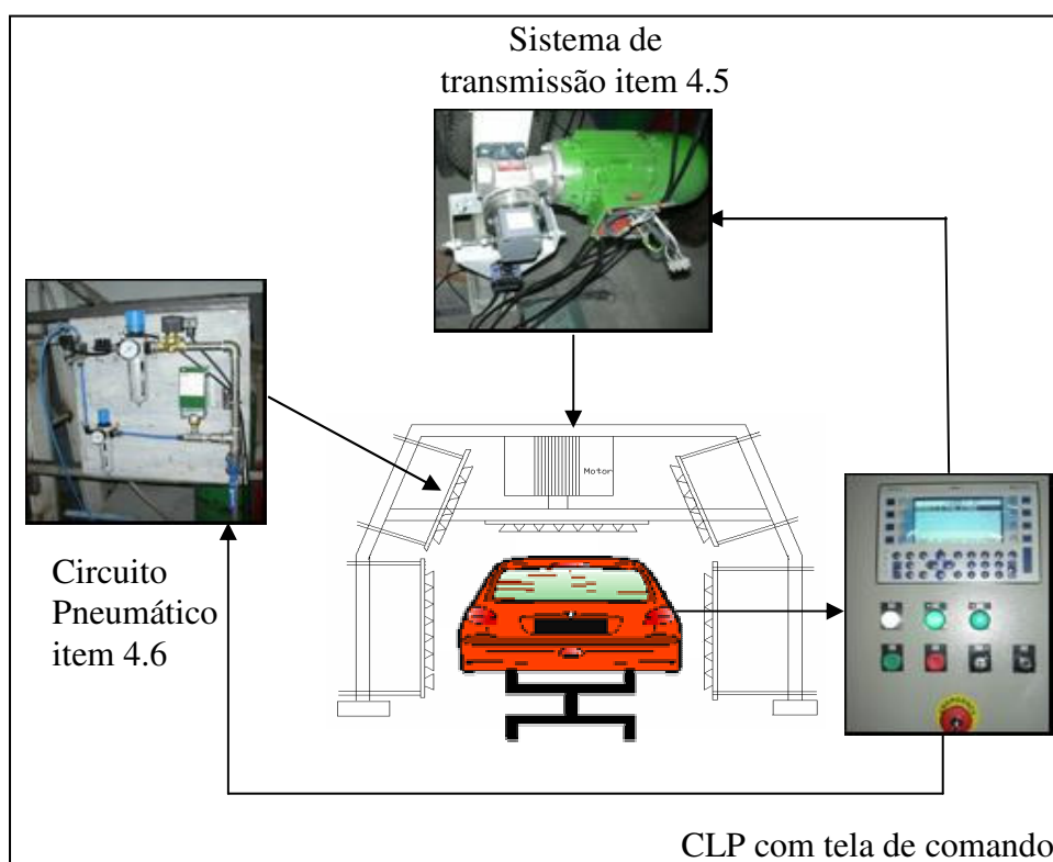
Figura 7.7 - Diagrama geral da cortina de ar
