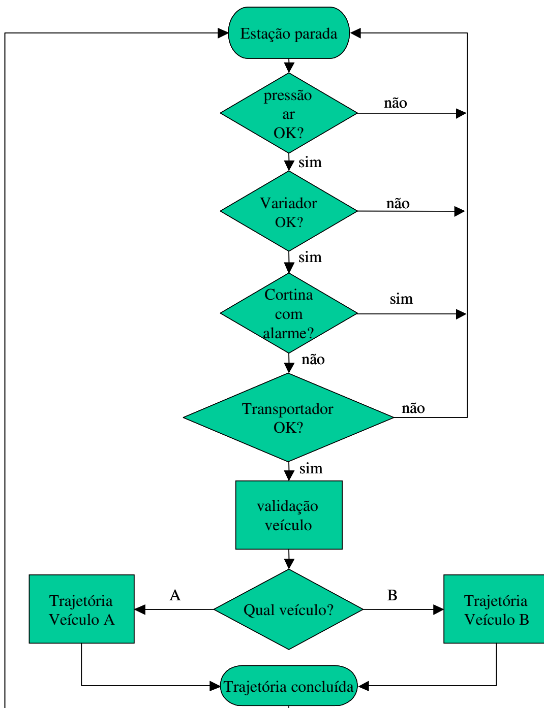
Figura 6.1 – Diagrama do funcionamento da cortina
