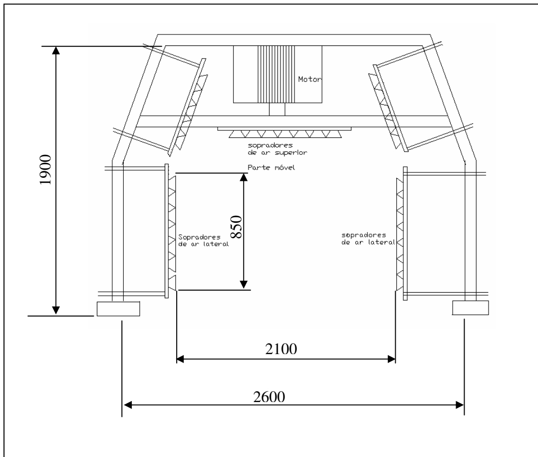
Figura 4.2 – Cortina de ar proposta
