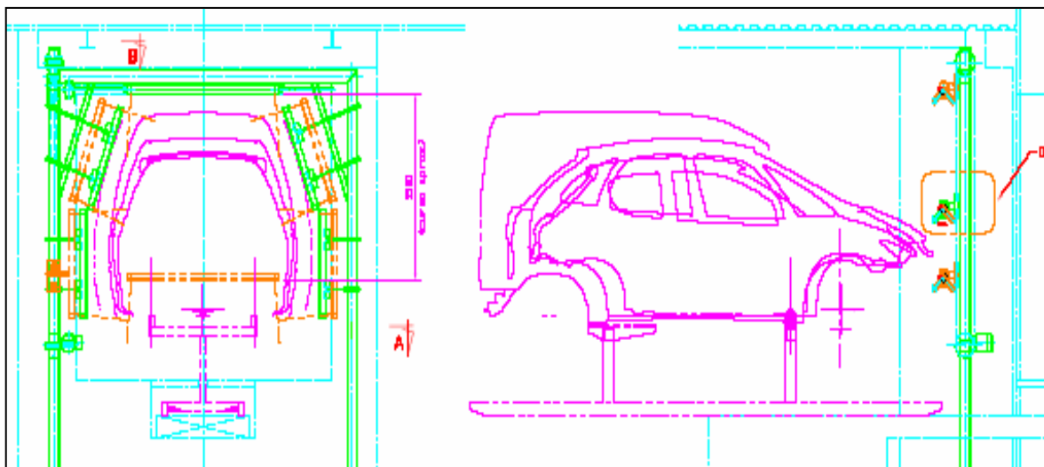
Figura 4.3 – Cortina de ar proposta vista lateral
