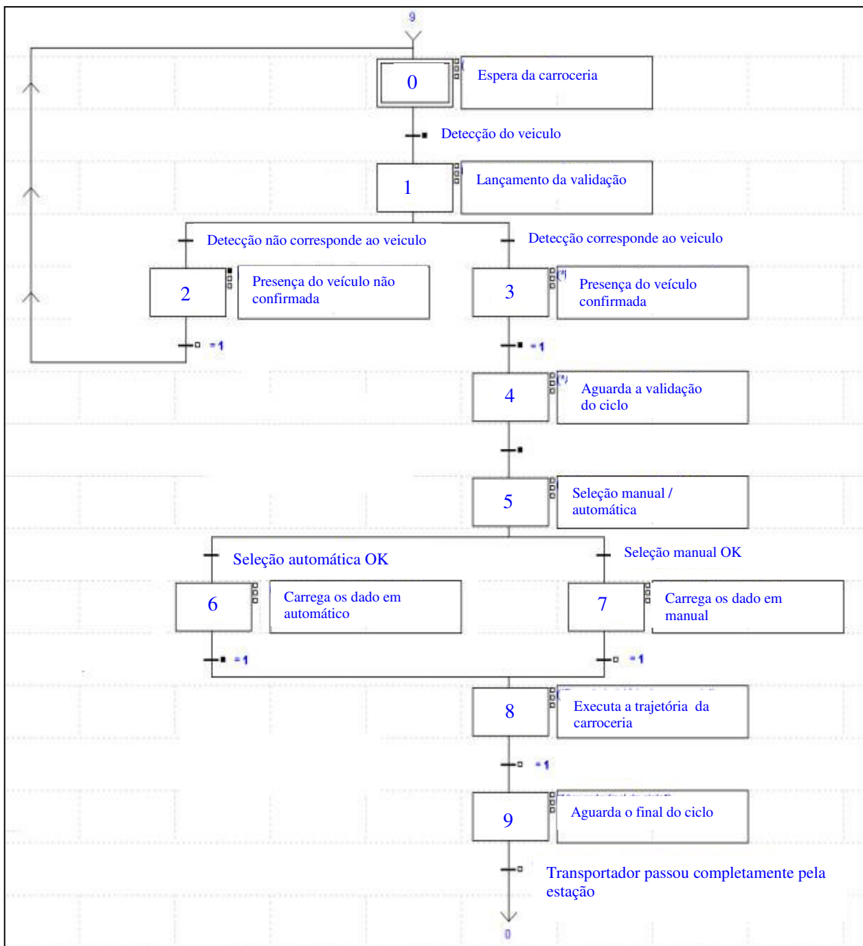
Figura 5.9 – Modelo final funcionamento da cortina em GRAFCET (tela do programa PL7 PRO da Schneider )
