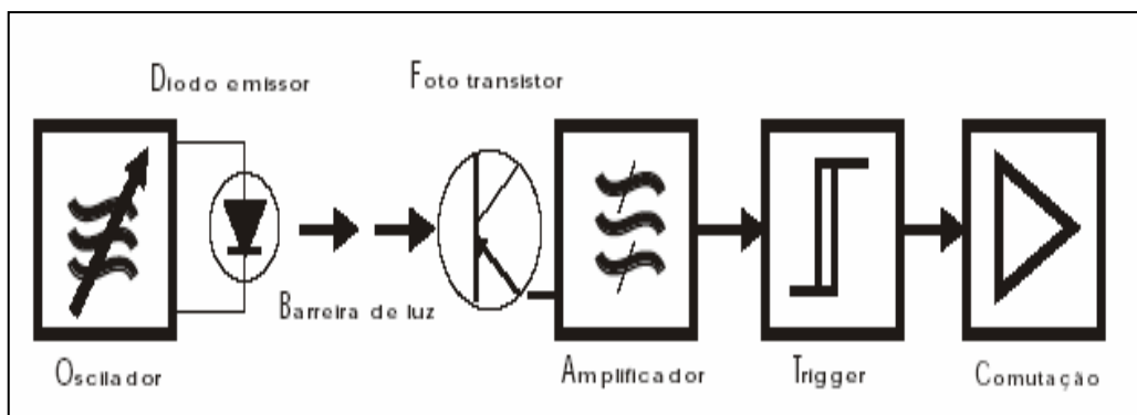
Figura 6.4 – Diagrama de blocos do sensor óptico por barreira
