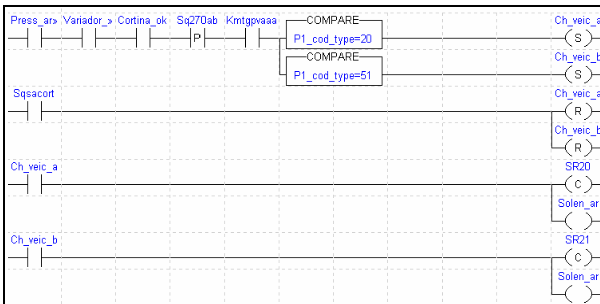
Figura 6.2 – Programação da movimentação da cortina em ladder
