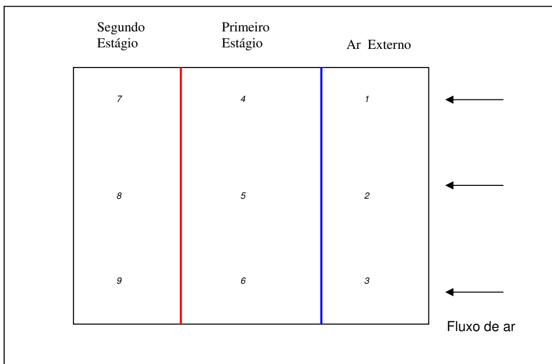
Figura 3.2 – Casa de ar das cabines
