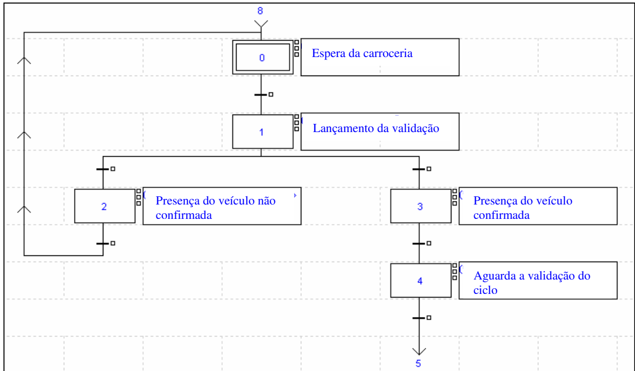
Figura 5.7 – Modelo Grafcet para a identificação do veículo (tela do programa PL7 PRO da Schneider )
