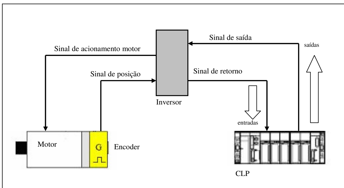
Figura 4.10 – Comunicação do motor com o CLP
