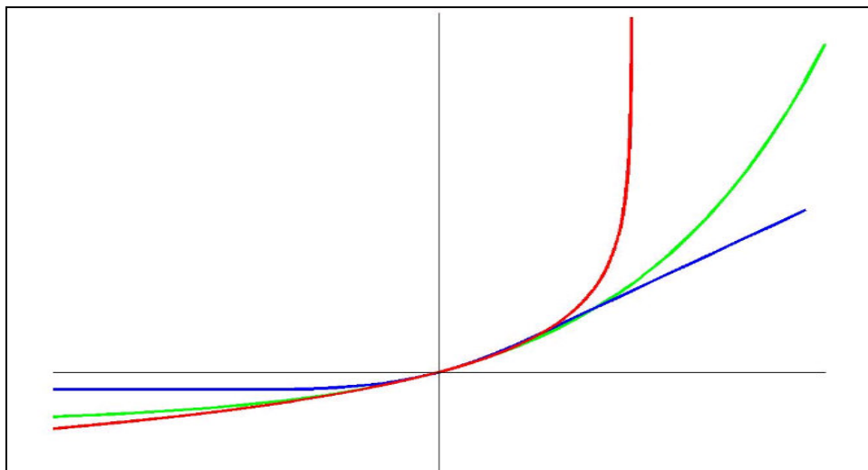
FIGURA 5.1 – FUNÇÕES DE PENALIDADES DA FAMÍLIA P .
