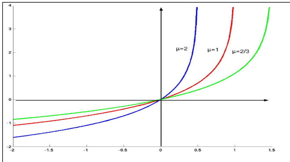
FIGURA 5.4 – PENALIDADE LOGARITMICA \theta(\mu y) COM VALORES FIXOS DE \mu .
