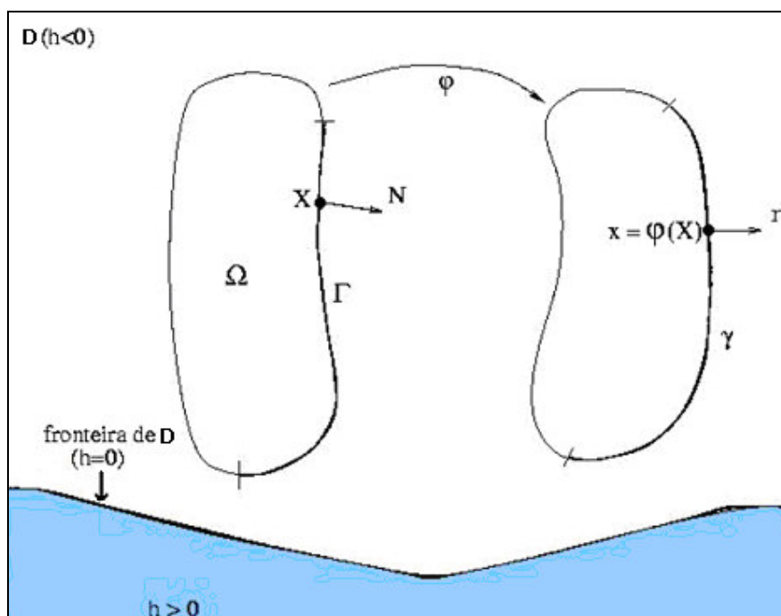
FIGURA 3.1 – NOTAÇÃO PARA O PROBLEMA DE CONTATO.
