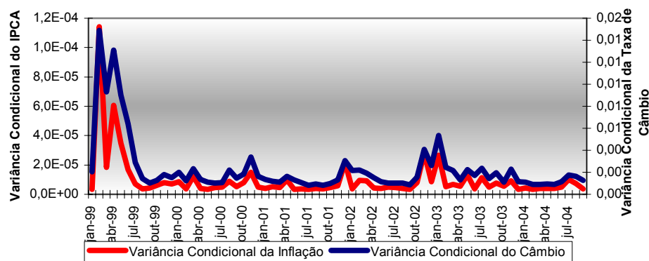
Gráfico 4.7 - Variâncias Condicionais - IPCA e Taxa de Câmbio R$/US$
