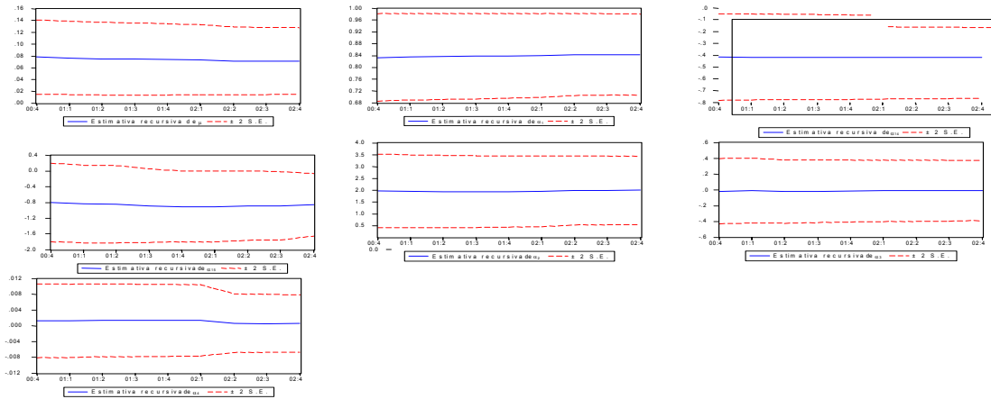
Gráfico B.16 – IGP - Coeficientes Recursivos - modelo com dummies
