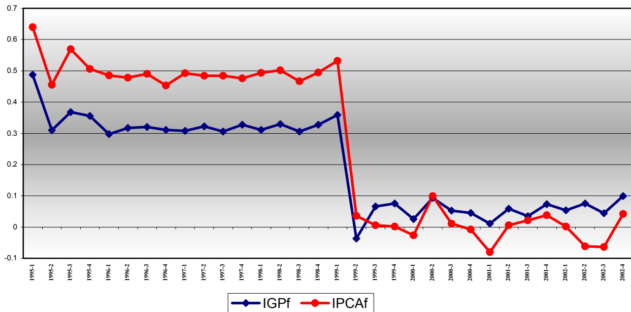
Gráfico 3.5 – Estimativa filtradas para o período pós-Real de \alpha_{1,t} : IGP-DI vs. IPCA
