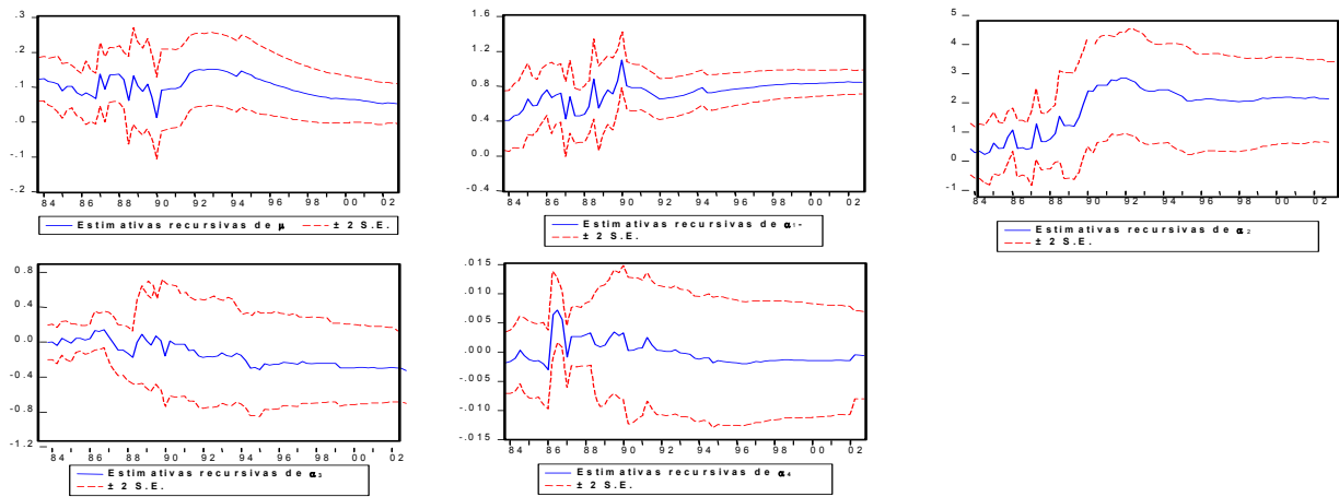
Gráfico B.2 – IPCA - Coeficientes Recursivos (período completo)
