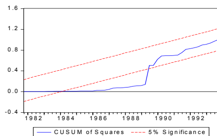
Gráfico B.11 – IGP - Teste Cusum dos Quadrados -Período pré-Real
