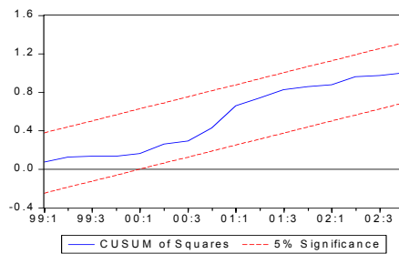
Gráfico B.15 – IGP - Teste CUSUM dos Quadrados - modelo com dummies
