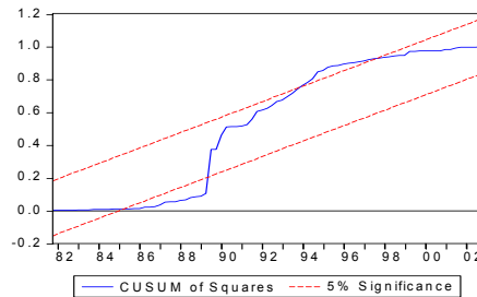
Gráfico B.9 – IGP - Teste Cusum dos Quadrados (período completo)
