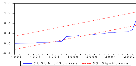
Gráfico B.21 – IPA - Teste Cusum dos Quadrados -Pós- Real
