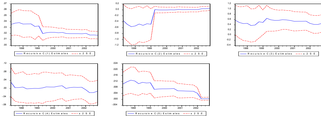
Gráfico B.6 – IPCA - Coeficientes Recursivos- período pós-Real
