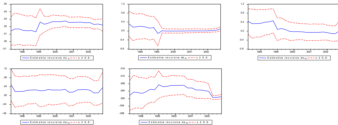
Gráfico B.14 – IGP - Coeficientes Recursivos Período pós-Real
