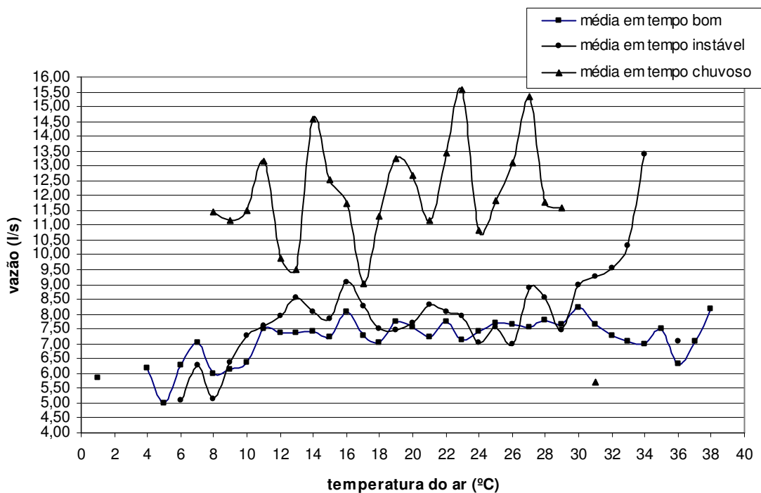
Figura 30 - Variação da vazão nos dias de tempo seco, instável e chuvoso em função da temperatura do ar
