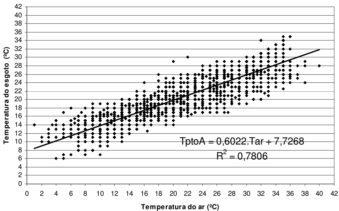
Figura 7 – Correlação entre a temperatura do ar e a temperatura do esgoto no ponto A
