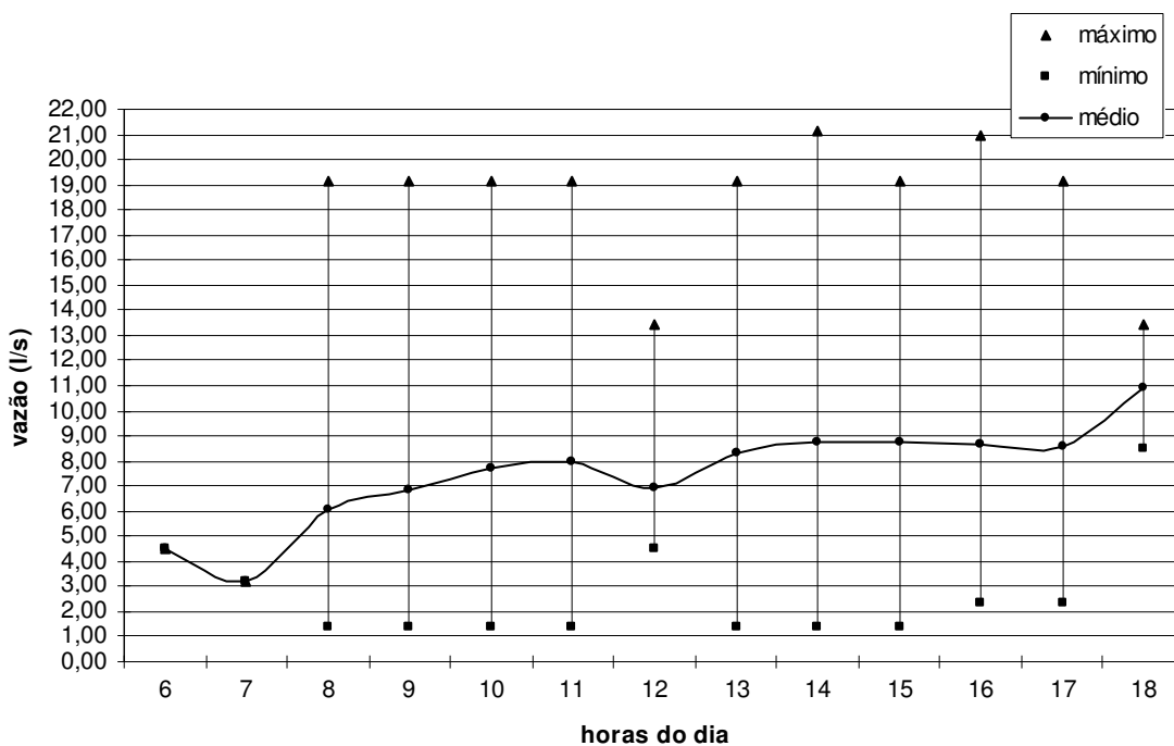
Figura 31 - Variação da vazão média em função das horas do dia
