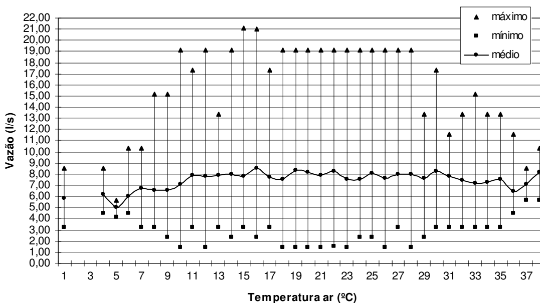
Figura 26 - Variação da vazão no sistema em função da temperatura do ar
