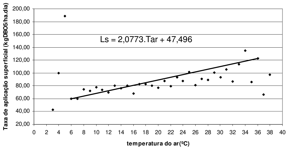
Figura 35 - Taxa de aplicação superficial no sistema em função da temperatura do ar
