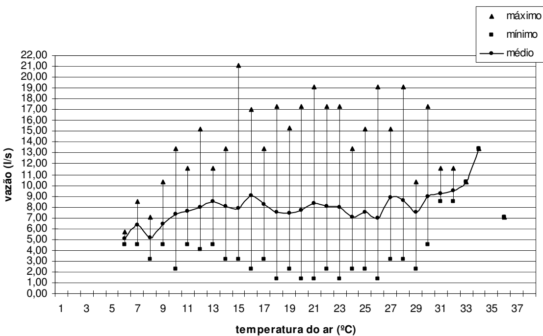
Figura 28 - Variação da vazão nos dias de tempo instável em função da temperatura do ar
