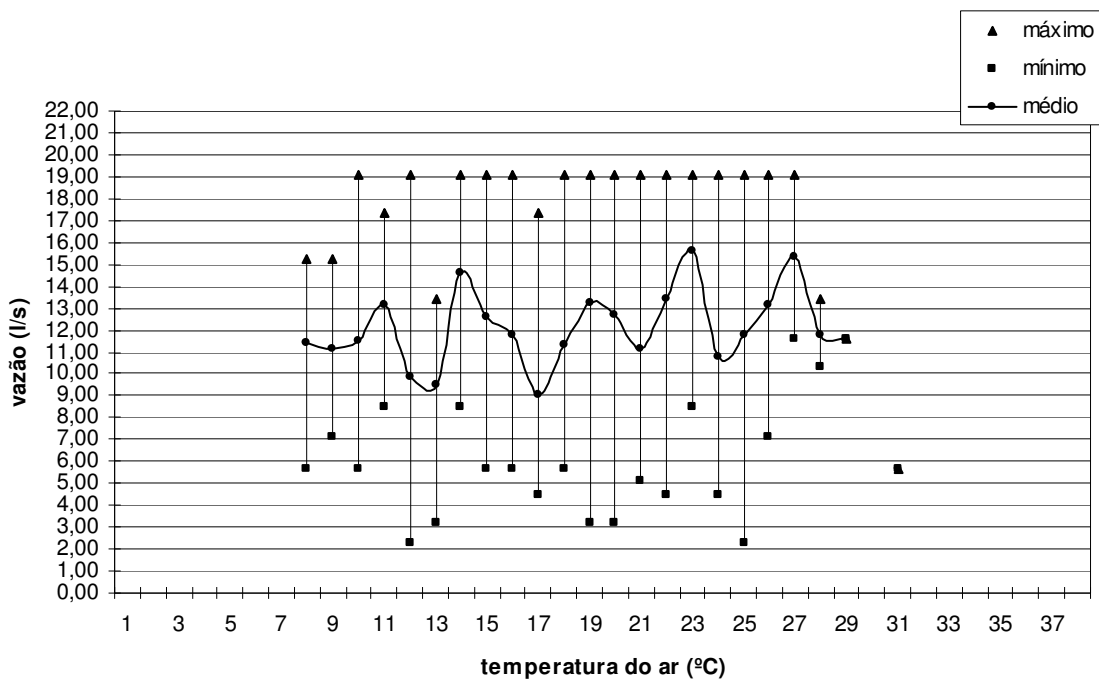
Figura 29 - Variação da vazão nos dias de tempo chuvoso em função da temperatura do ar
