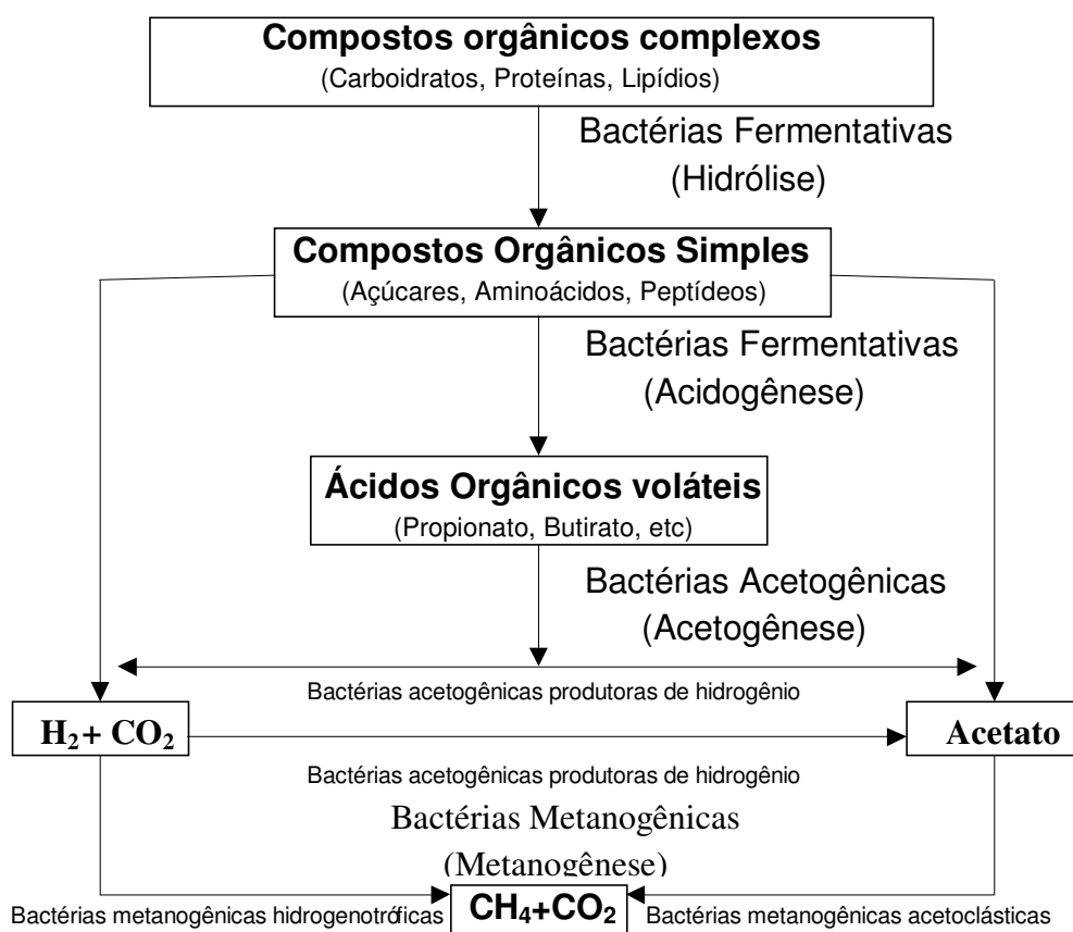
Figura 2 - Seqüência metabólica e microorganismos envolvidos na digestão anaeróbia
