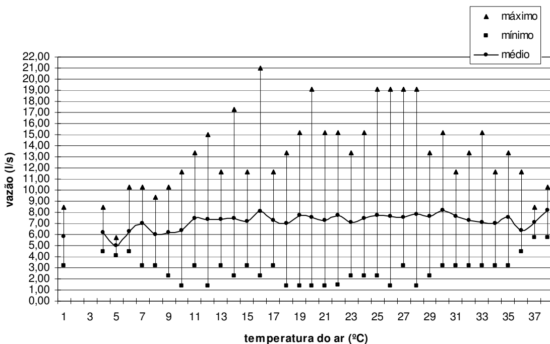
Figura 27 - Variação da vazão nos dias de tempo seco em função da temperatura do ar
