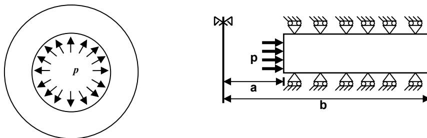
Figura 4.1 – Cavidade Cilíndrica – Problema Físico.
