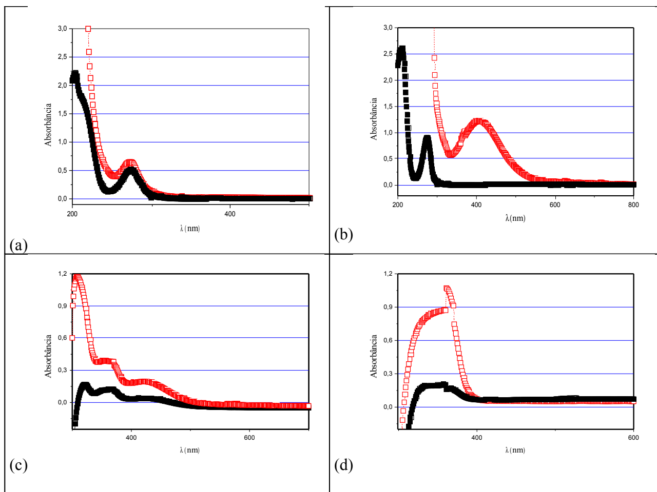
Figura 35: Espectros UV antes (símbolo aberto) e após 24 horas (símbolo fechado) de incubação da lacase imobilizada com soluções de (a) guaiacol, (b) pirocatecol, (c) pirogalol e (d) vanilina.
