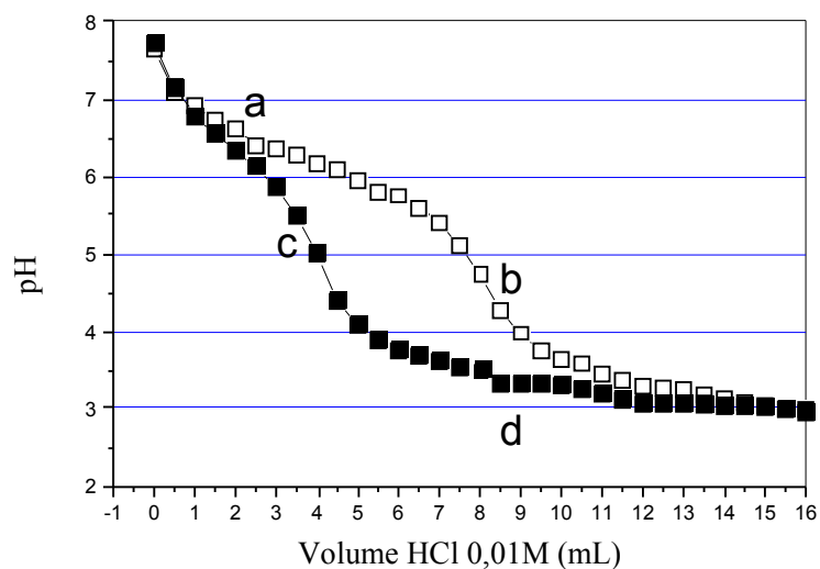
Figura 34: Curva de titulação potenciométrica do efluente antes e após incubação com a lacase imobilizada por 24 horas utilizando como titulante solução de HCl 0,01M. O (símbolo aberto) representa o efluente sem tratamento e o (símbolo fechado) após tratamento. Os pontos das curvas representam as médias de 3 repetições.
