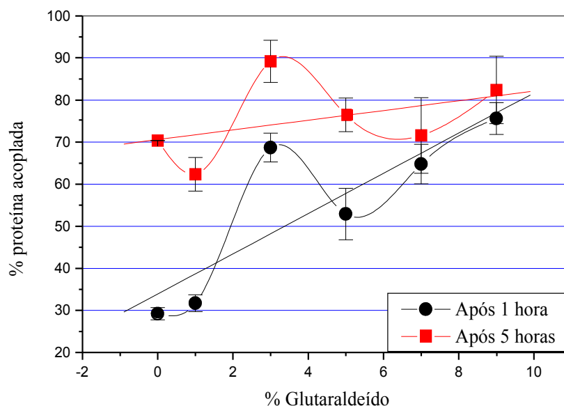
Figura 18: Porcentagem de proteínas acopladas após 1 e 5 horas de incubação da solução enzimática (0,5 g/L) com esferas de quitosana ativadas com diferentes porcentagens de glutaraldeído.
