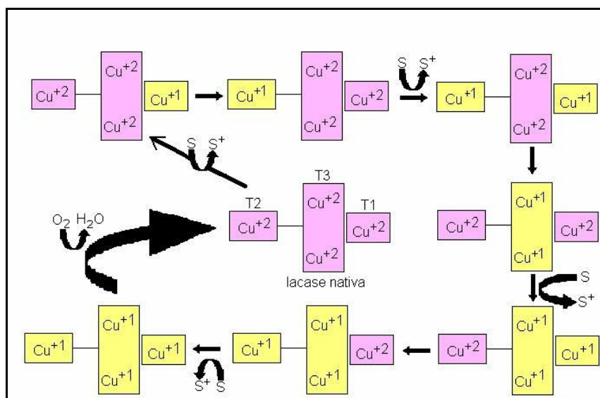
Figura 7: Ciclo catalítico das lacases (Modificado de DURÁN et al., 2002).
