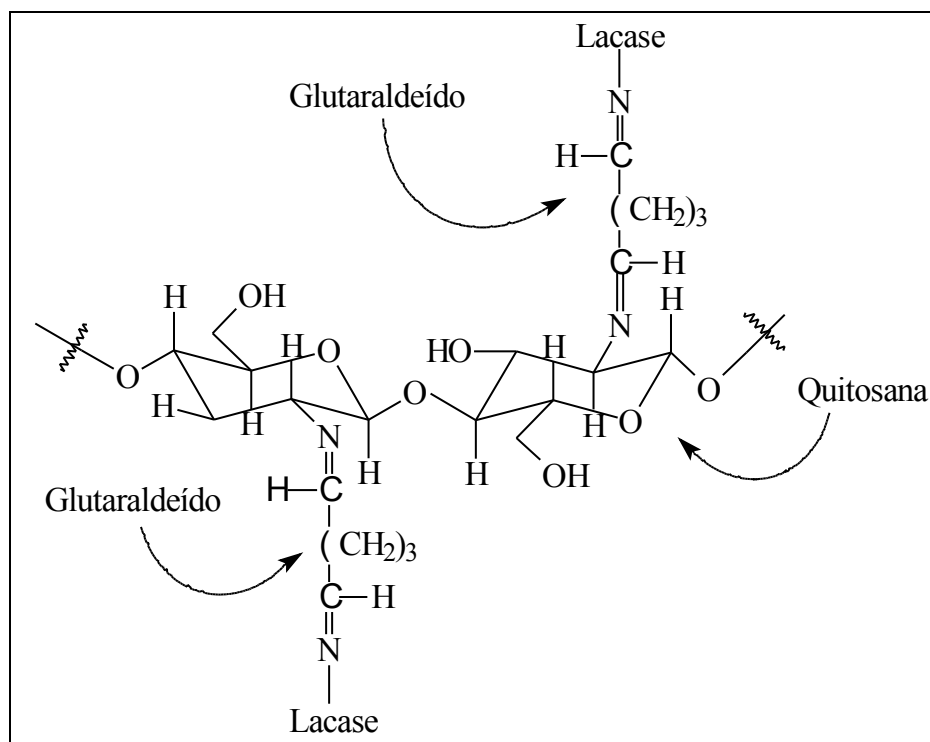
Esquema 2: Ilustração esquemática da enzima imobilizada sobre o suporte (esferas de quitosana) com auxílio do agente bifuncional (glutaraldeído) (JIANG et al., 2005).
