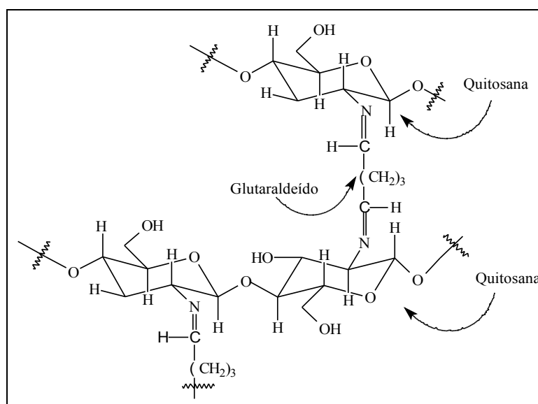
Esquema 1: Ilustração esquemática das ligações cruzadas entre duas cadeias poliméricas de quitosana com o glutaraldeído.
