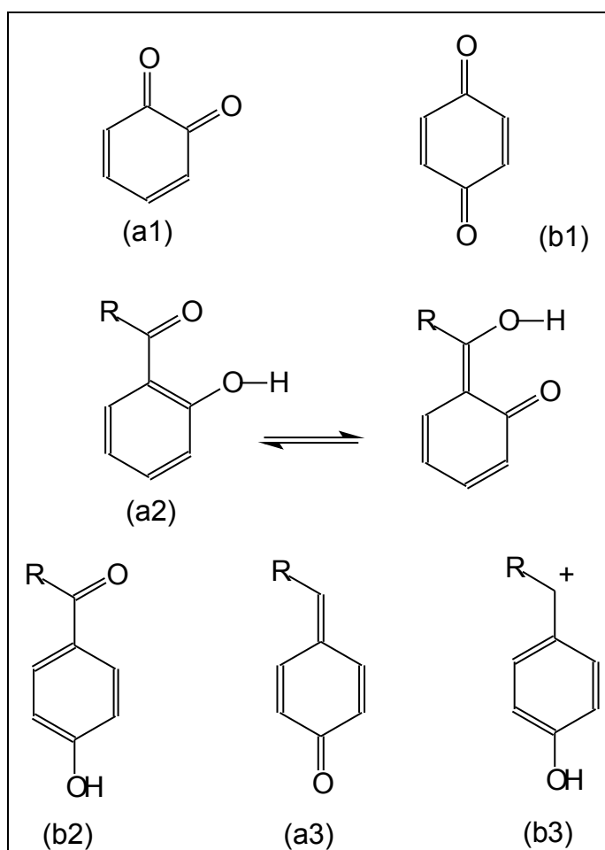
Esquema 4: Principais estruturas cromóforas básicas identificadas na madeira
