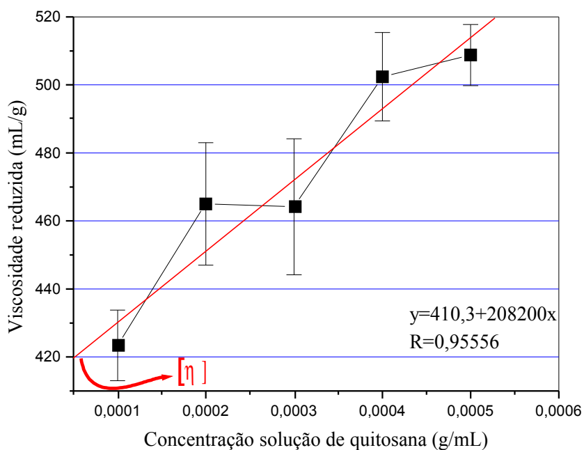
Figura 13: Curva de viscosidade reduzida versus concentração da solução de quitosana.
