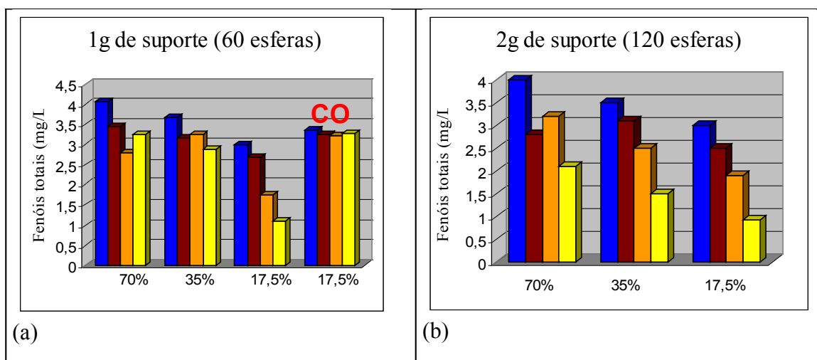
Figura 31: Concentração de fenóis totais em amostras de efluente de diferentes concentrações, incubadas com 1g (a) e 2g (b) de suporte contendo enzima imobilizada, após o tempo de reação: 0 h (azul); 1 h (vermelho); 3 h (laranja) e 24 h (amarelo) . CO representa o conjunto de dados da incubação do efluente com esferas de quitosana sem a enzima imobilizada.(controle).
