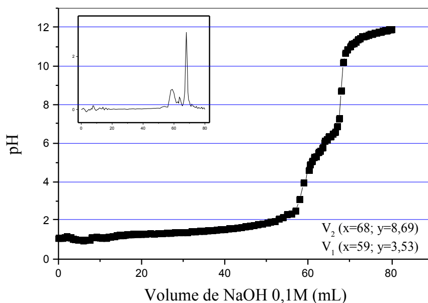
Figura 12: Curva de titulação potenciométrica da solução de quitosana e ácido clorídrico (0,3 M). Os pontos representam a média de três determinações. O quadro menor ilustra a derivada primeira da curva de titulação, onde os pontos máximos representam os pontos de inflexão.
