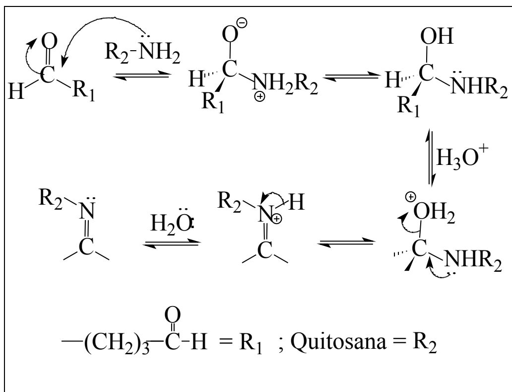
Esquema 3: Mecanismo proposto para formação do grupo imino.
