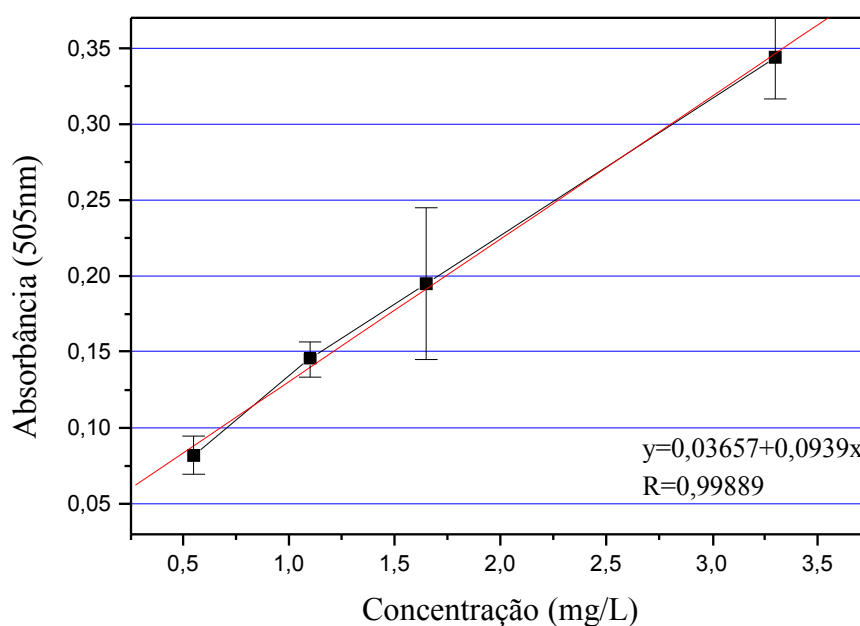
Figura 37: Curva de calibração para determinação de fenóis de baixa MM (método da 4-AAP) utilizando soluções com diferentes concentrações de fenol.
