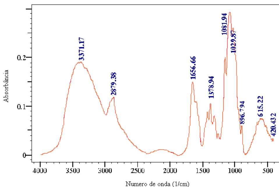
Figura 15: Espectro Infravermelho da quitosana em pastilha de KBr.
