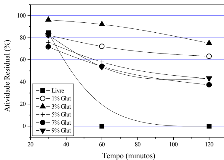
Figura 21: Atividade residual da enzima livre e imobilizada em esferas ativadas com soluções de diferentes porcentagens de glutaraldeído após 30, 60 e 120 minutos de pré-incubação em tampão tartarato (0,1M) pH=4,0 e temperatura de 50°C. Os pontos das curvas representam as médias de três repetições.
