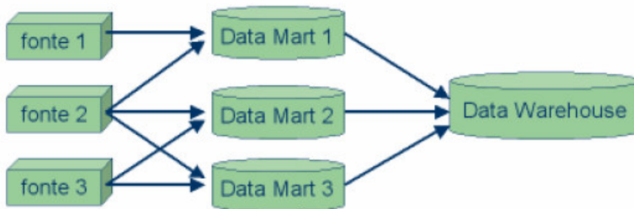
Figura 4 - Abordagem Botton - UP
