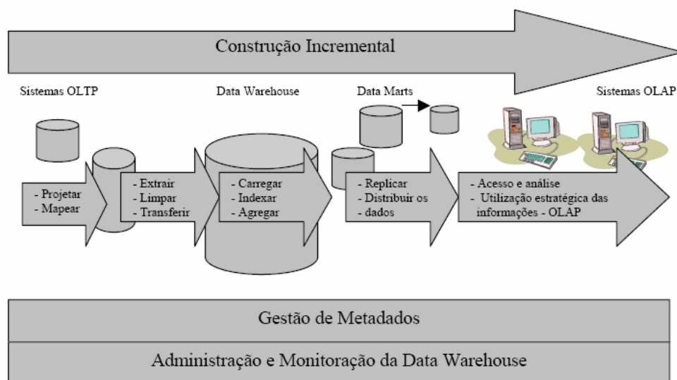
Figura 1 - O Processo de Data Warehousing
