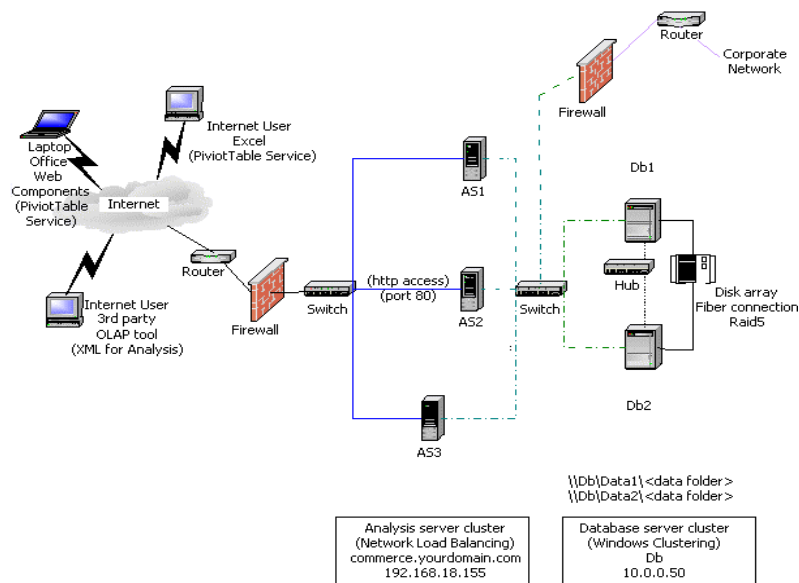
Figura 48 - Proposta de Ambiente para Solução BI Microsoft
