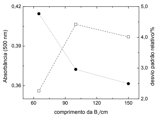
FIGURA 4.24 Efeito do comprimento da bobina reacional B_1 sobre o sinal analítico de uma solução de referência de acetilcisteína 9,6 \times 10^{-5} \text{ mol L}^{-1} ( n=3 ). Absorvância (--□--) e precisão (...●...).
