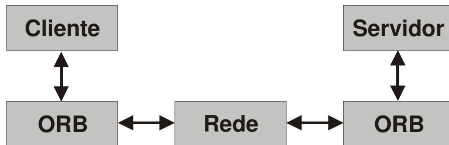
Figura 2.3. Arquitetura CORBA.
