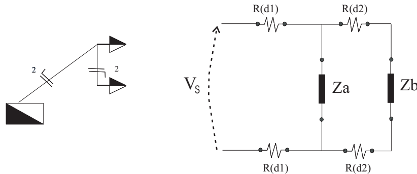
Figura A.3: Um circuito da instalação modelado com componentes de circuitos elétricos.
