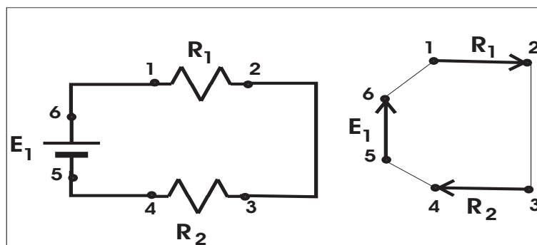
Figura 3.4: Formação de um circuito através das conexões .
