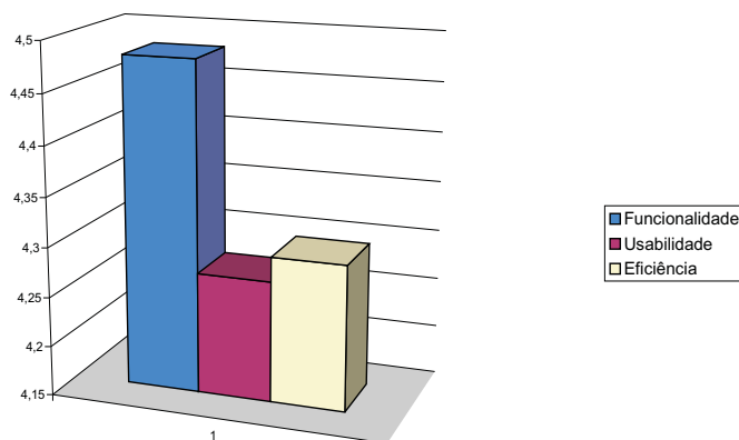
Figura 6.20: Critérios IsoNorm.
