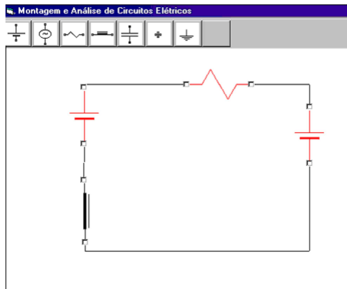
Figura 3.8: Circuito simulando.
