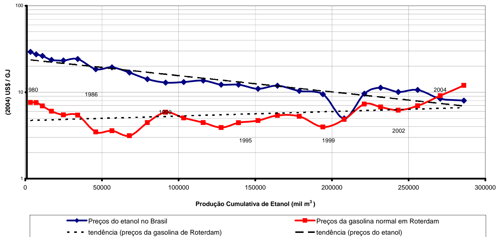
Figura 22 Curva de aprendizado do etanol de cana-de-açúcar
