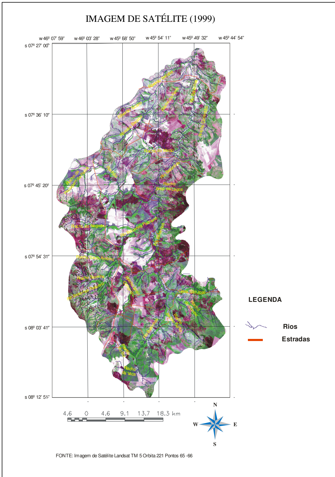
Figura 22. Imagem de satélite TM/LANDSAT 5 da bacia do rio Balsinhas (1999).
