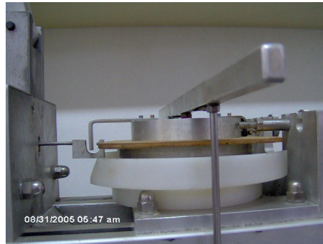
FIGURA 43 - Determinação do ângulo de atrito com a parede.
