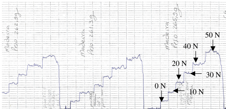
FIGURA 45 - Força registrada para cisalhar a amostra nos ensaios de cisalhamento com a parede
