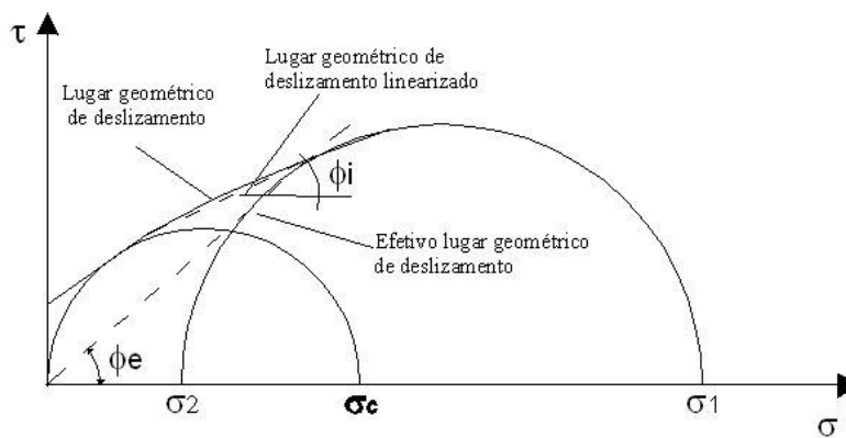
FIGURA 7 - Lugar geométrico de deslizamento.
