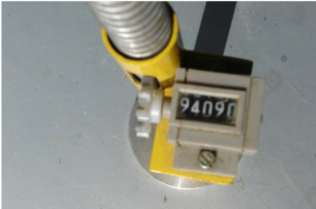
FIGURA 2. Detalhe do contador do disco medidor de forragem.
