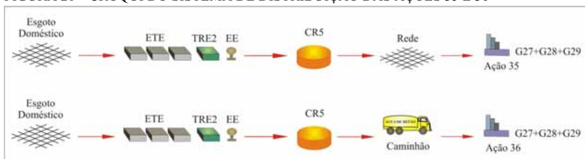
FIGURA 21 – CROQUI DO SISTEMA DE DISTRIBUIÇÃO DAS AÇÕES 35 E 36
