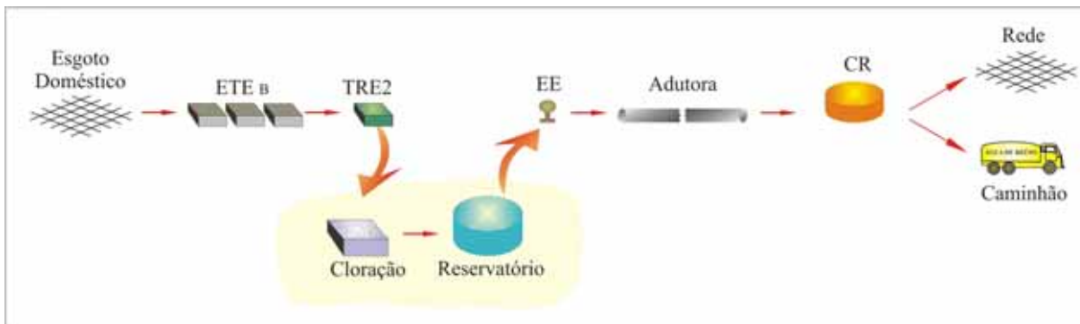
FIGURA 22 – SISTEMA GERAL DO TRATAMENTO E DISTRIBUIÇÃO DE ESGOTO DA ETE BELÉM
