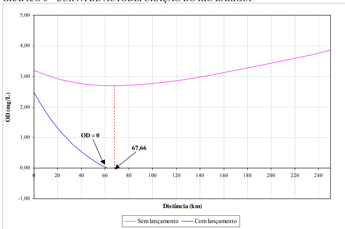
GRÁFICO 8 – CURVA DE AUTODEPURAÇÃO DO RIO BARIGÜI
