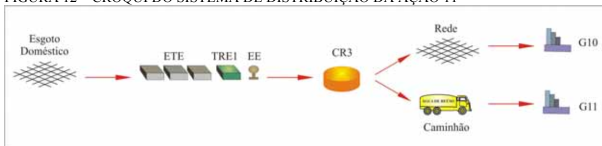
FIGURA 12 – CROQUI DO SISTEMA DE DISTRIBUIÇÃO DA AÇÃO 11
