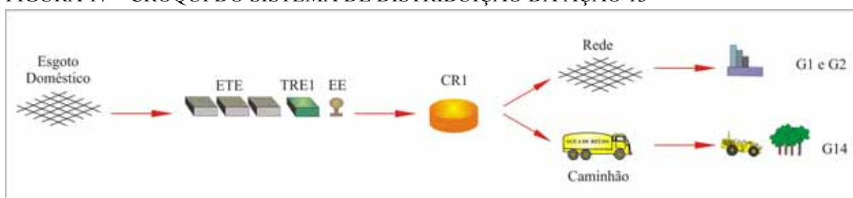
FIGURA 17 – CROQUI DO SISTEMA DE DISTRIBUIÇÃO DA AÇÃO 13
