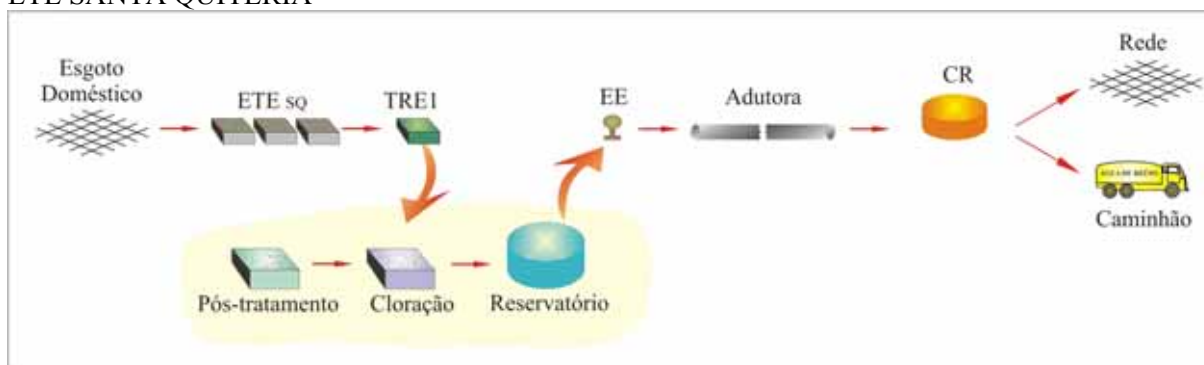
FIGURA 13 – SISTEMA GERAL DO TRATAMENTO E DISTRIBUIÇÃO DE EFLUENTE DA ETE SANTA QUITÉRIA
