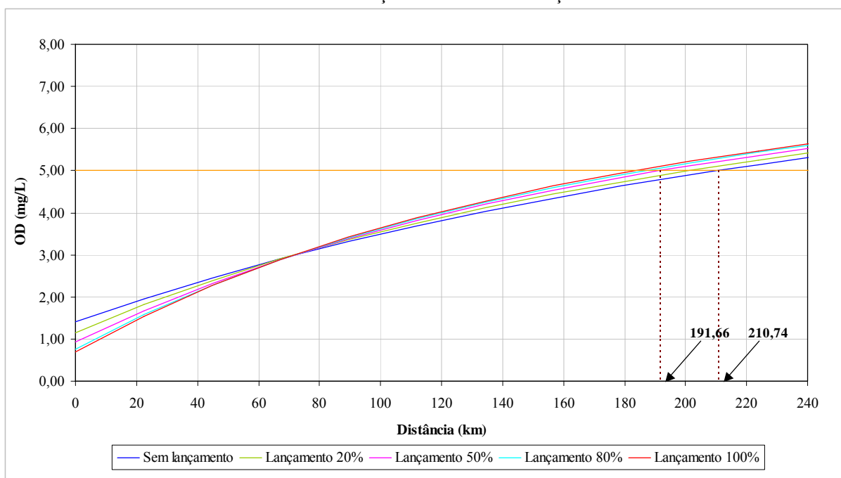
GRÁFICO 7 – CURVA DE AUTODEPURAÇÃO DO RIO IGUAÇU
