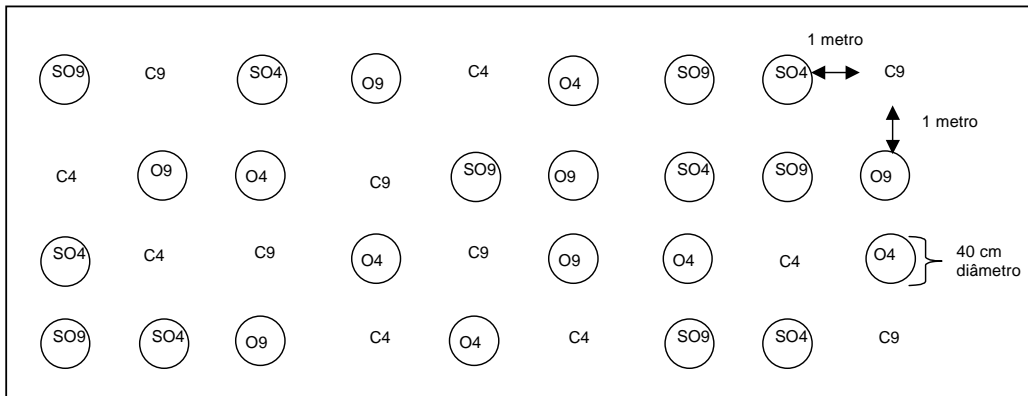
Figura 2: Desenho amostral esquemático do experimento em campo (O – corer com óleo bruto; SO – corer sem óleo; C – controle natural; 4 - horas após adição do óleo, 9 - horas após a adição do óleo).
