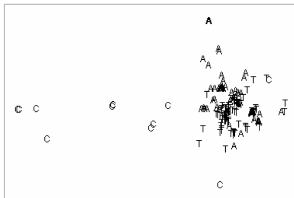
Figura 3: MDS (Multi-dimensional Scaling) realizado com a densidade das espécies da macrofauna (stress = 0,01), encontrada nas amostras coletadas na laguna Armazém (A), Canal (C) e laguna Tramandaí (T).
