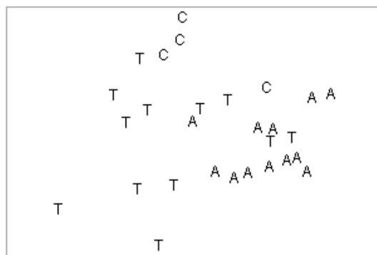
Figura 2: Análise MDS (Multi-dimensional Scaling ordination), realizada com a densidade média da meiofauna (stress=0,19), considerando a laguna Armazém (A), Canal (C) e laguna Tramandaí (T).
