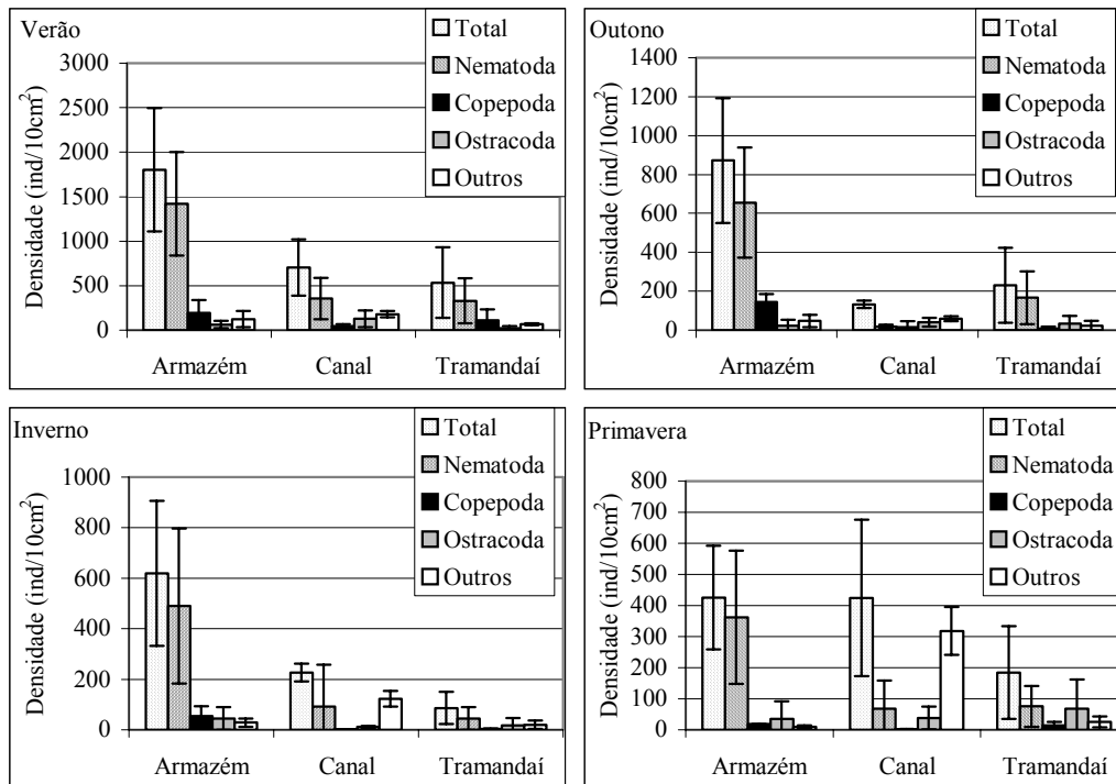
Figura 4: Densidade média (ind/10cm 2 ) e desvio padrão das amostras de meiofauna total, e grupos mais representativos, por laguna, coletadas no verão, outono, inverno e primavera de 2000.
