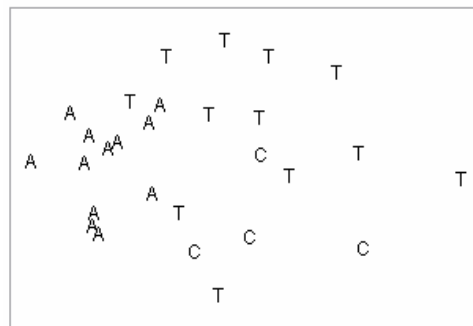
Figura 3: MDS (Multi-dimensional Scaling ordination) realizado com a densidade dos gêneros de Nematoda, considerando a média das amostras (stress = 0,08), coletadas na laguna Armazém (A), Canal (C) e laguna Tramandaí (T).
