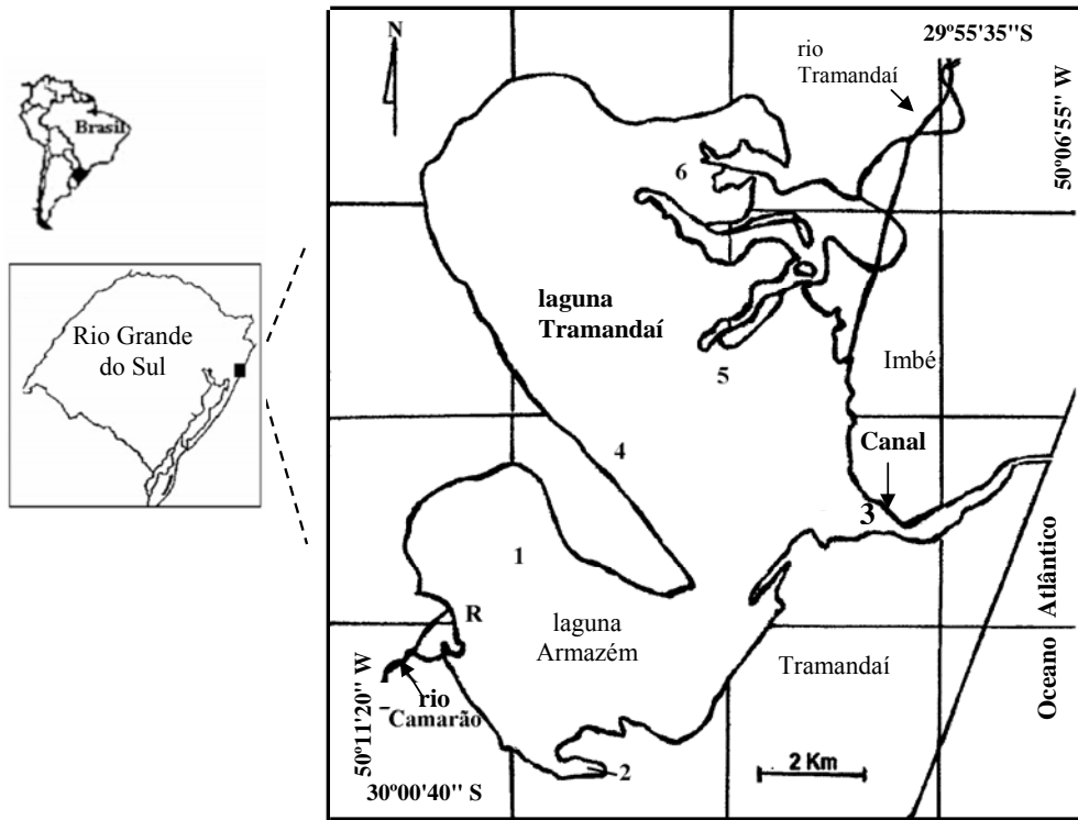
Figura 1: Mapa com a localização das áreas amostrais, no estuário Tramandaí-Armazém (modificado de Tabajara, 1994).
